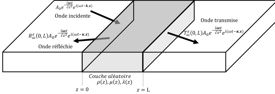
FIGURE 2.1 – Représentation du problème de propagation d'onde en milieu aléatoire. En amont est située l'onde incidence et l'onde réfléchie, et l'onde transmise est situé en aval de la couche aléatoire
