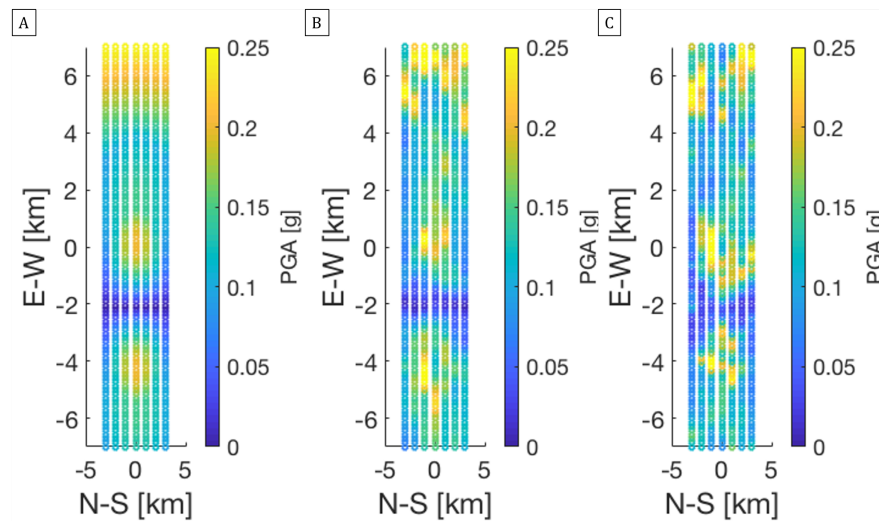
FIGURE 3.15 – Représentation des valeurs des PGA verticaux dans le cas des 3 milieux considérés différents. (A) correspond au cas homogène, (B) au cas hétérogène 1 et (C) au cas hétérogène 2
