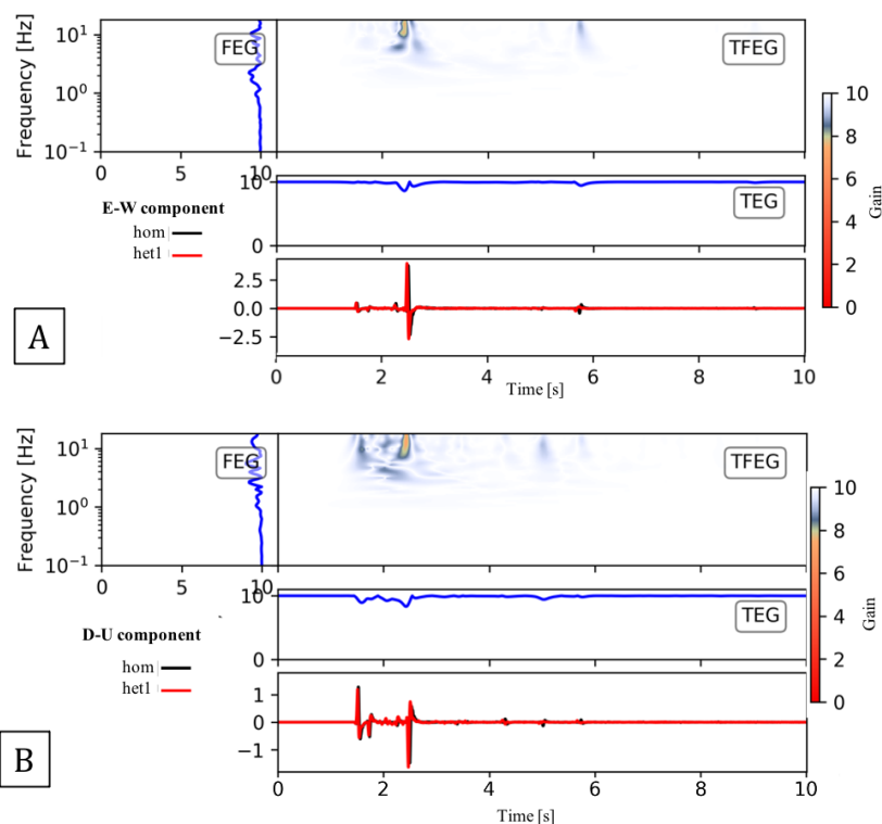
FIGURE 3.24 – Tracé de la transformée temps-fréquence du signal pour la composante EW (en haut) et la composante verticale (en bas). On indique le gain en se basant sur le critère de Kristekova pour une station placée à 4000 m de l'épicentre dans le cas homogène (en noir) et hétérogène 1 (en rouge)
