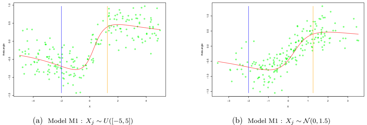
Figure 1.6: Une illustration pour les données simulées \{\Theta_j\}_{j=1}^n (points verts) du modèle-M1 avec n = 200 . La courbe rouge présente la vraie fonction de régression m , tandis que la ligne verticale bleue affiche le point x = -2 et la ligne verticale orange affiche le point x = 1.25 où nous estimons m(x) .
