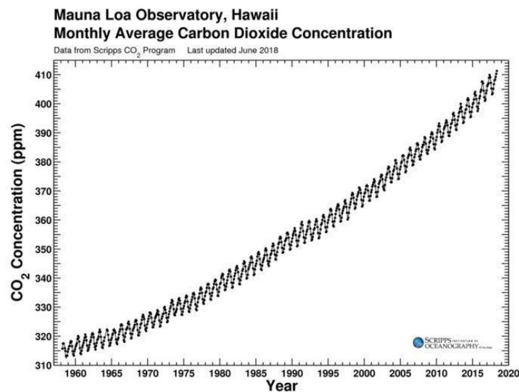
Figure 1 : variations de la concentration en carbone atmosphérique depuis 1960 (Keeling et al., 2005)
