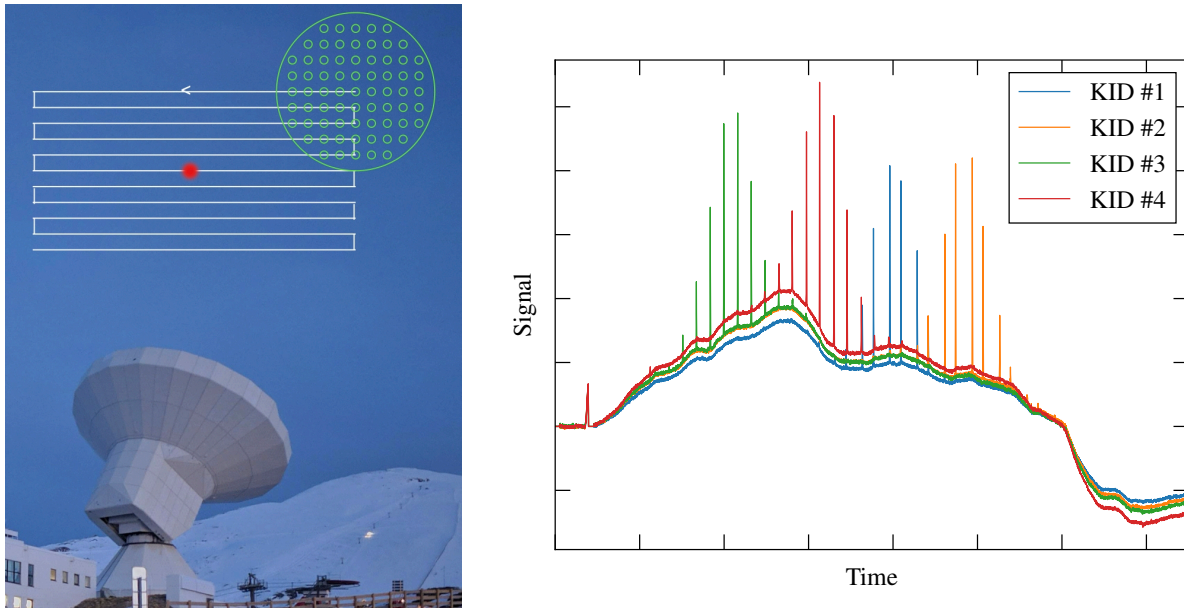
Figure 3.5 : Gauche : illustration du mouvement effectué par le télescope dans le ciel (en blanc) lors d'un scan OTF. La matrice de détecteurs est représentée en vert, et la source observée en rouge. Droite : représentation des données ordonnées en temps obtenues par scan d'Uranus pour trois KID. La détection de la source se manifeste par un pic de signal détecté.
