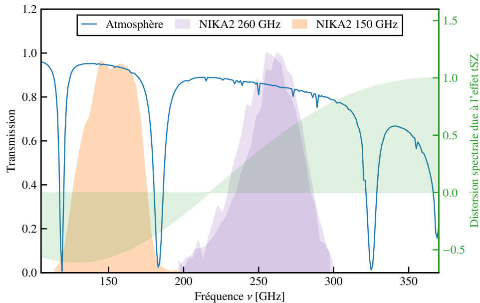
Figure 3.4 : Bandes passantes de NIKA2 à 260 GHz (violet) et 150 GHz (orange). La transmission atmosphérique calculée à partir du modèle de Pardo et al. [127] pour 2 mm de vapeur d'eau précipitable est également représentée en bleu. La distorsion spectrale due à l'effet tSZ est montrée en vert.
