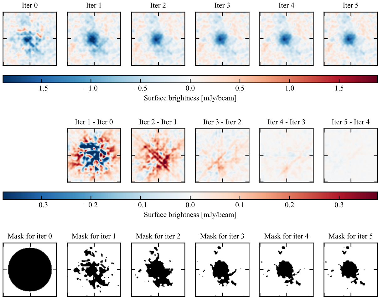
Figure 4.3 : Évolution (de gauche à droite) des résultats avec les itérations de la décorrélation pour les observations NIKA2 de l’amas PSZ2-G183.90+42.99. Haut : Carte de brillance de surface obtenue pour chaque itération. Centre Différence entre la carte de brillance de surface obtenue pour une itération et pour l’itération précédente. Bas : Masque utilisé pour l’évaluation du mode commun pour chaque itération.
