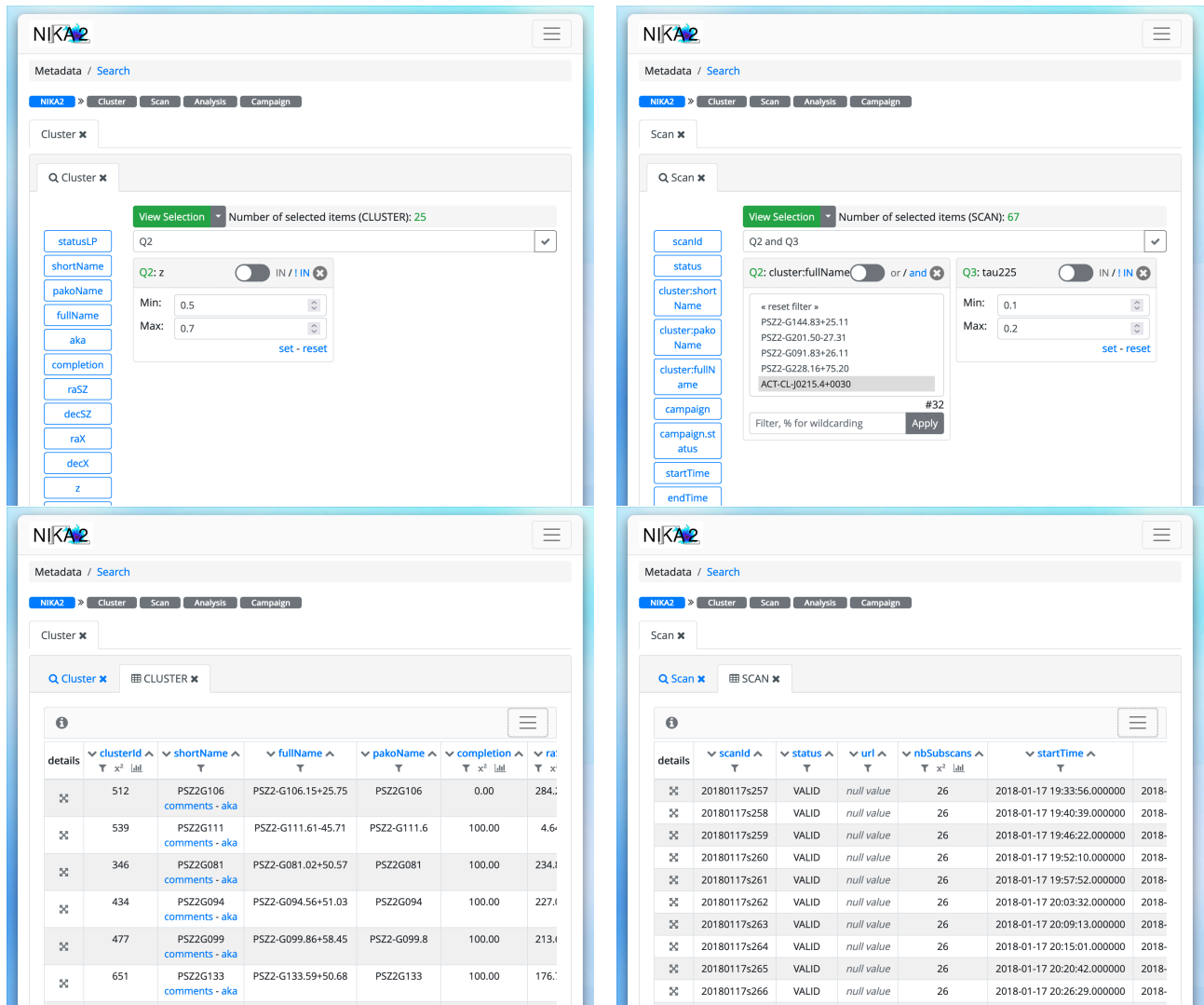
Figure 3.12 : Deux exemples de requêtes dans l’interface graphique de AMI (haut) et leurs résultats (bas). Gauche : recherche des amas du grand programme SZ dont le redshift est compris entre 0.5 et 0.7. Droite : recherche des scans de l’amas ACT-CL J0215.4+0030 ayant été effectués pour une opacité atmosphérique \tau_{225} entre 0.1 et 0.2.
