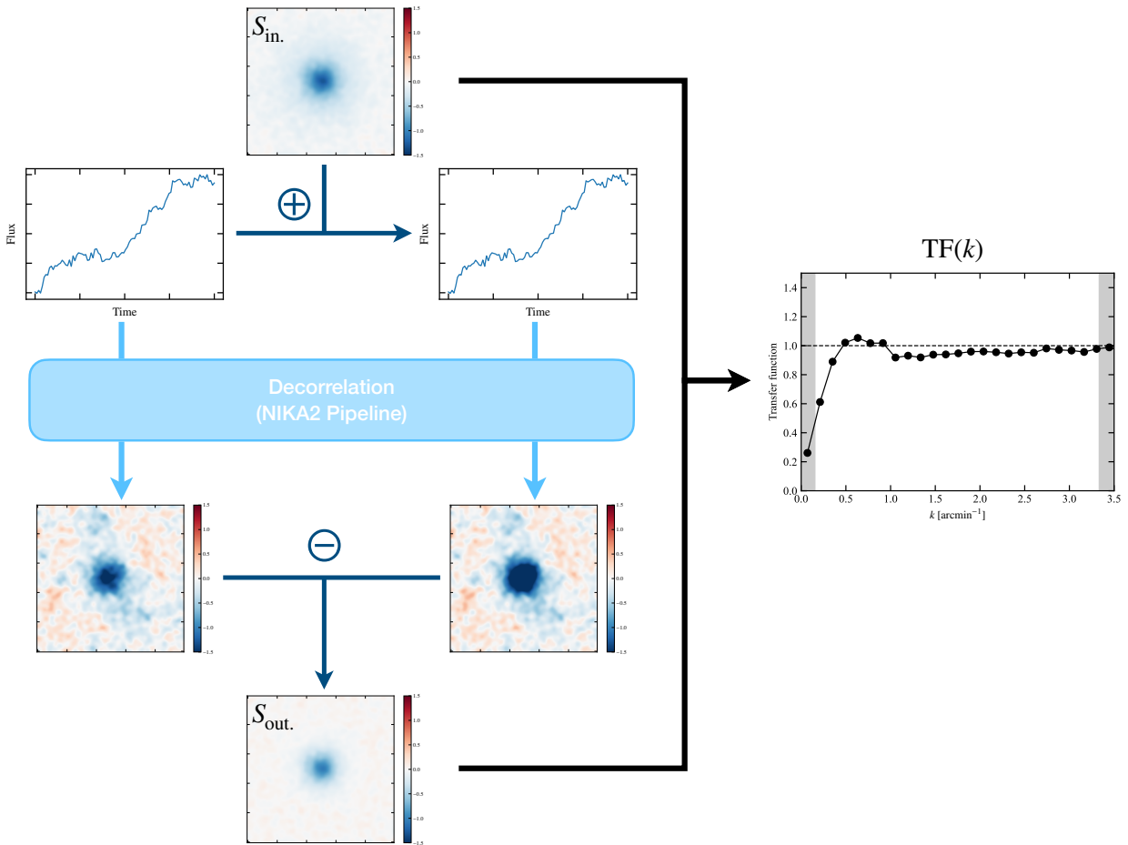
Figure 4.6 : Illustration du calcul de la fonction de transfert pour la décorrélation common mode one block de l'amas PSZ2-G183.90+42.99 (voir figure 4.3). Le rapport entre les spectres de puissance d'une carte simulée d'entrée ( S_{in.} , haut) et de la carte après décorrélation ( S_{out.} , bas) donne la fonction de transfert de la décorrélation.
