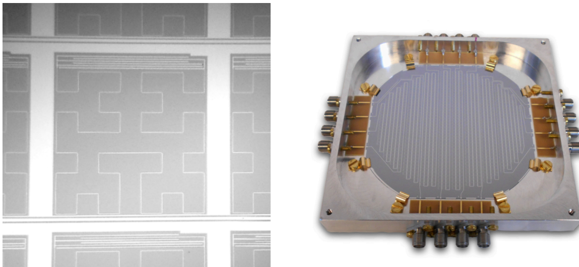
Figure 3.3 : Gauche : Image d'un détecteur KID de NIKA, de taille 2.3 \text{ mm} \times 2.3 \text{ mm} . Le méandre inductif du détecteur couvre la plupart de sa surface, tandis que la partie capacitive C est située dans la partie haut du détecteur. Droite : Matrice de KID dans la bande à 260 GHz de NIKA2, comportant 1140 KID et 8 lignes de transmission. Figures extraites de [123].
