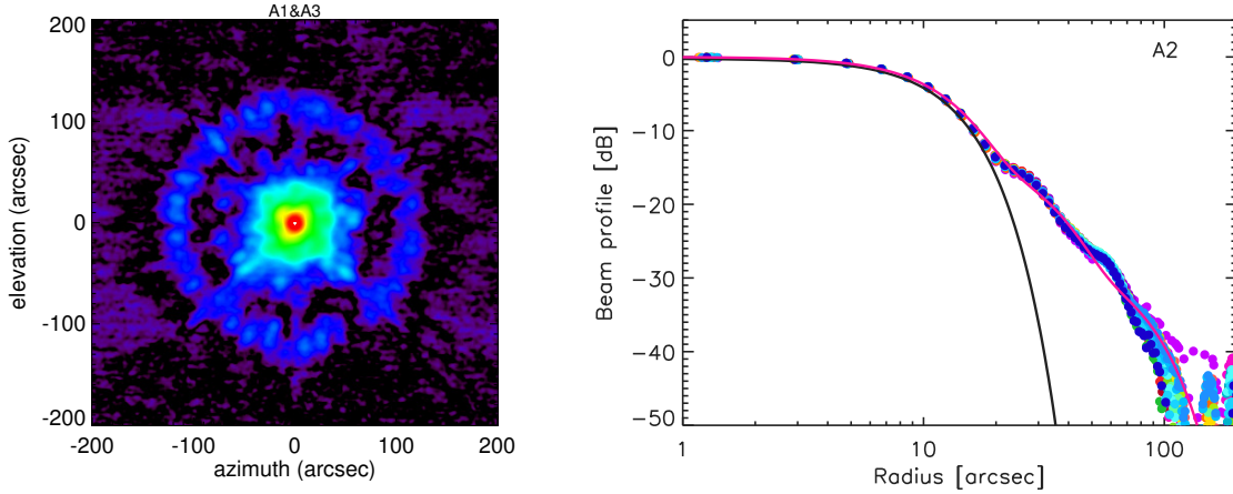
Figure 3.8 : Gauche : Lobe de NIKA2 à 260 GHz mesuré par empilement de cartes d’Uranus. Droite : Profils radiaux du lobe à 150 GHz mesurés pour plusieurs beammaps (points colorés). Le lobe principal et complet, ajusté avec un modèle à trois gaussiennes, sont respectivement représentés en noir et magenta. Figures extraites de [12].
