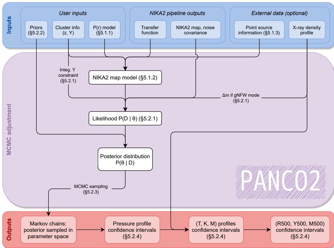
Figure 5.1 : Schéma représentant le principe de fonctionnement de PANC02. Les données d'entrée sont les produits standards pour les observations NIKA2 d'amas de galaxies, produits par le pipeline d'analyse des données brutes présenté au chapitre 4, ainsi que des données externes telles que les profils radiaux mesurés en X ou les informations sur les sources ponctuelles.
