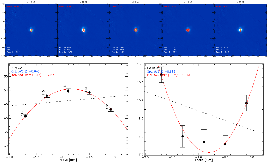
Figure 3.7 : Exemple de procédure de focalisation du télescope. Haut : cartes à 150 GHz d’Uranus obtenue pour cinq distances primaire-secondaire. Bas : Flux d’Uranus ( gauche ) et largeur à mi-hauteur ( droite ) mesurées dans chacune des cartes (noir). L’ajustement des points avec une loi parabolique (rouge) permet de mesurer la distance permettant une focalisation optimale du télescope (bleu).
