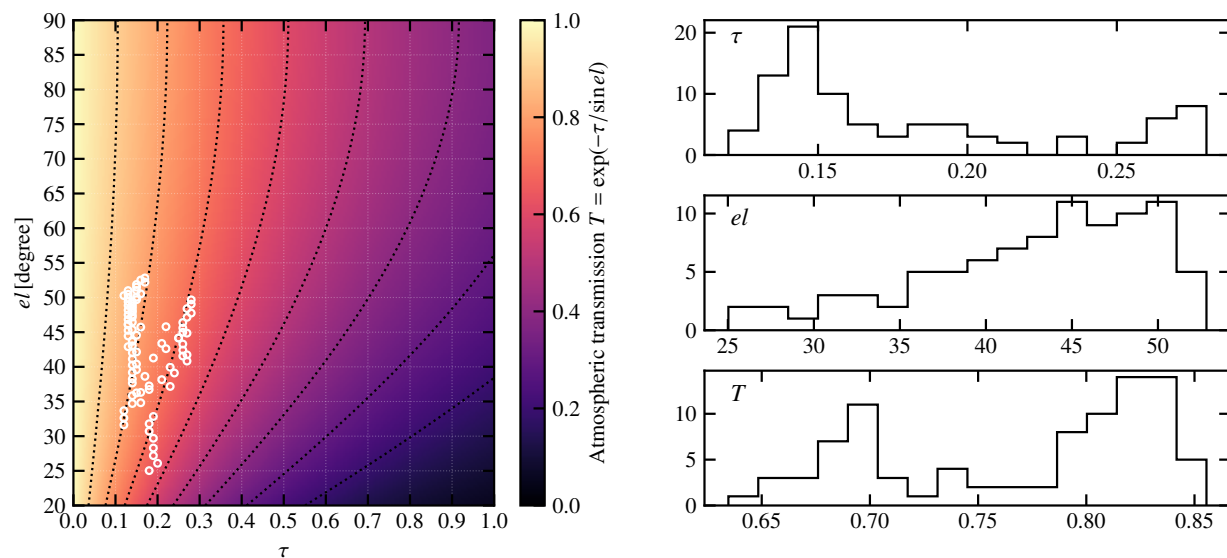
Figure 6.1 : Gauche : transmission atmosphérique T en fonction de l'opacité \tau et de l'élévation el . Chaque point blanc représente un scan de ACT-CL J0215.4+0030. Droite : Distribution des opacités ( haut ), élévations ( centre ), et transmissions atmosphériques ( bas ) pour les scans de ACT-CL J0215.4+0030.
