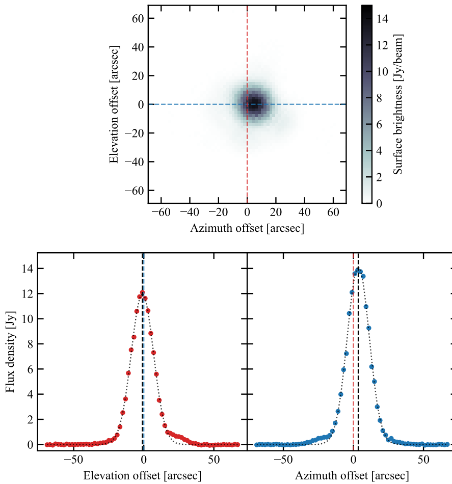
Figure 3.6 : Exemple de procédure de pointage. Haut : carte d'Uranus obtenue avec un scan en croix, suivant les directions des lignes bleue puis rouge, projetée en utilisant la matrice de pointage avant correction de pointage. Bas : profils de la planète le long de l'axe des élévations ( gauche ) et des azimuts ( droite ). L'ajustement des profils par une gaussienne (courbes pointillées noires) permet de mesurer le centre de la source dans les deux directions (lignes noires verticales). La différence entre la position de la source et celle du centre de la carte donne les corrections de pointage utilisées pour réaligner le KID de référence.
