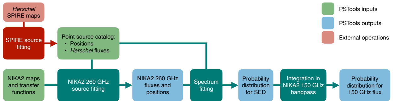
Figure 4.7 : Schéma illustrant le fonctionnement de PSTools. Les données d'entrée sont représentées en vert, et les données de sortie en bleu. La partie rouge représente les opérations externes au logiciel, c'est-à-dire la détection des sources dans les cartes SPIRE.
