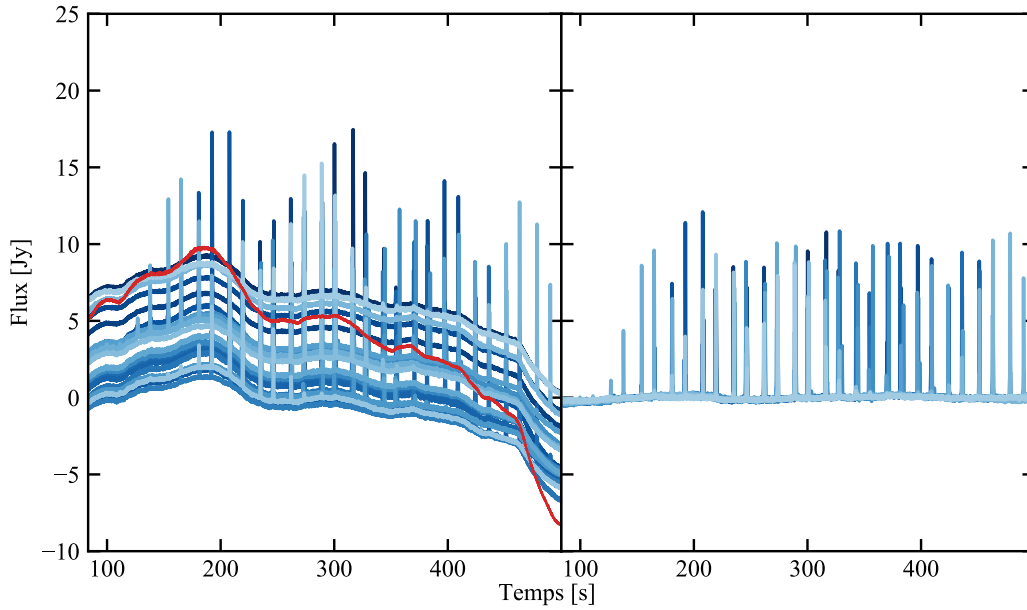
Figure 4.1 : Gauche : Données en temps pour 20 détecteurs de la matrice à 150 GHz de NIKA2 lors d’une observation d’Uranus (bleu). Le passage de chaque KID sur la planète est visible par les pics d’émission décalés en temps. Le mode commun estimé sur les TOI de la matrice entière est représenté en rouge.
