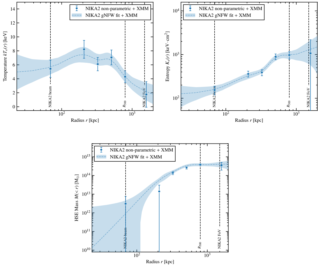
Figure 5.8 : Profils de température ( haut gauche ), d’entropie ( haut droit ), et de masse hydrostatique ( bas ) obtenus par combinaison du profil de pression ajusté par PANC02 et du profil de densité mesuré en X pour ACT-CL J0215.4+0030. Les points bleus représentent la combinaison du meilleur ajustement du profil de pression en non-paramétrique avec le profil de densité mesuré en X. Les enveloppes bleues représentent l’incertitude sur ces profils obtenue par interpolation gNFW des résultats non-paramétriques.
