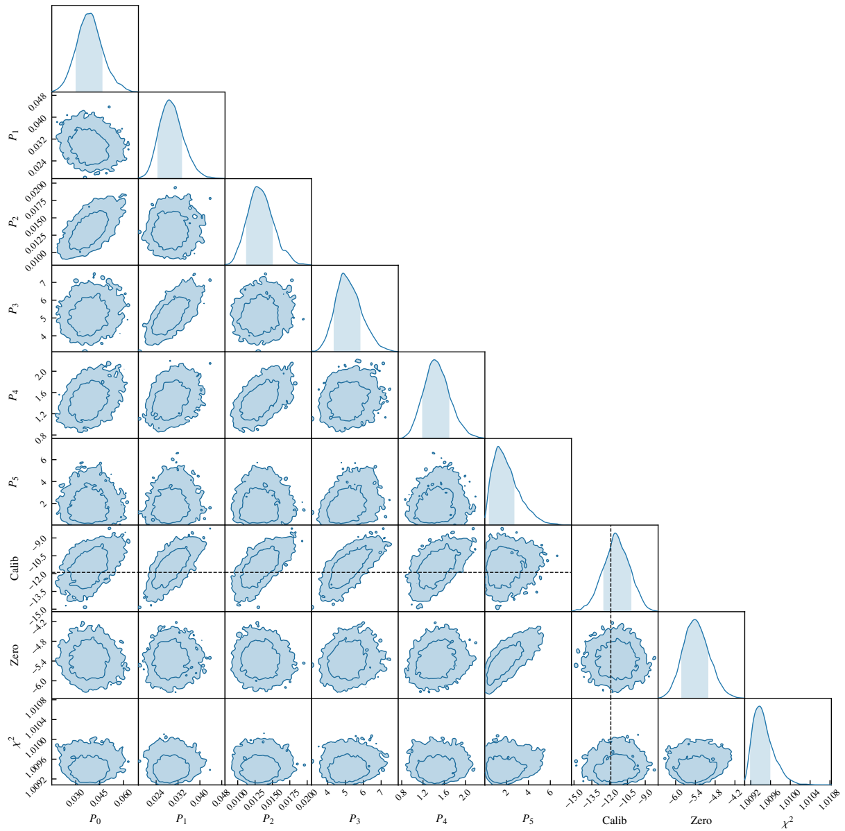
Figure 5.6 : Distribution postérieure dans l'espace des paramètres. Les éléments diagonaux représentent les distributions marginalisées sur chacun des paramètres, et les extra-diagonaux les distribution à deux dimensions pour chaque couple de paramètres. Les contours représentés sont les intervalles de confiance à 1\sigma et 2\sigma . La ligne noire pointillée correspond à la vraie valeur du coefficient de conversion.
