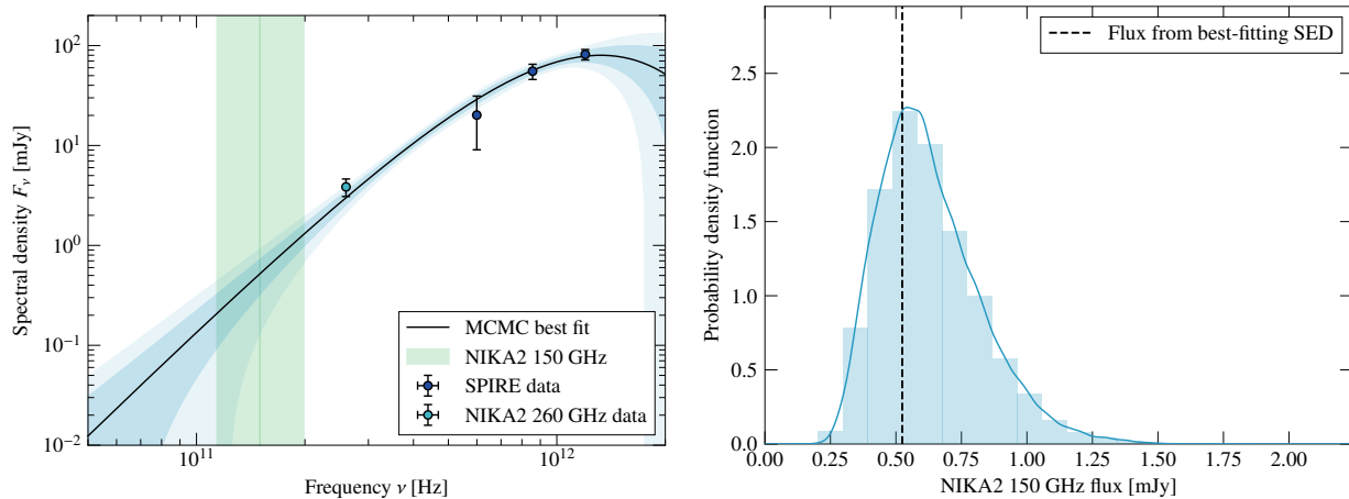
Figure 4.9 : Gauche : Résultat de l’ajustement de la SED de la source SMG1 dans le champ de l’amas ACT-CL J0215.4+0030, présenté au chapitre 6. Les points bleu foncé représentent des flux SPIRE. Les points bleu clair représentent le flux mesuré dans la carte NIKA2 à 260 GHz. La ligne bleue montre la SED ajustant le mieux les données, et les enveloppes l’entourant montrent les intervalles de confiance à 1\sigma et 2\sigma . La région verte correspond à la bande passante à 150 GHz de NIKA2. Droite : Distribution de probabilité du flux de SMG1 dans la bande passante à 150 GHz de NIKA2. L’histogramme représente la distribution des flux calculés grâce au MCMC (voir texte). La courbe bleue montre la densité de probabilité obtenue en appliquant une estimation par noyau à cette distribution. La ligne verticale noire montre le flux obtenu grâce à la SED ajustant le mieux les données.
