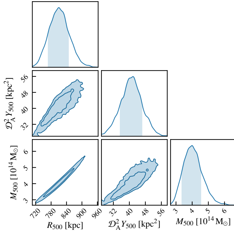
Figure 5.10 : Distributions des grandeurs caractéristiques intégrées R_{500} , Y_{500} , et M_{500} obtenues par l'ajustement avec PANCO2 de la carte simulée d'un amas synthétique. Les distributions présentées sont les distributions marginalisées à une dimension (éléments diagonaux) et à deux dimensions (éléments extra-diagonaux). Les contours présentés sont les intervalles de confiance à 1\sigma et 2\sigma .
