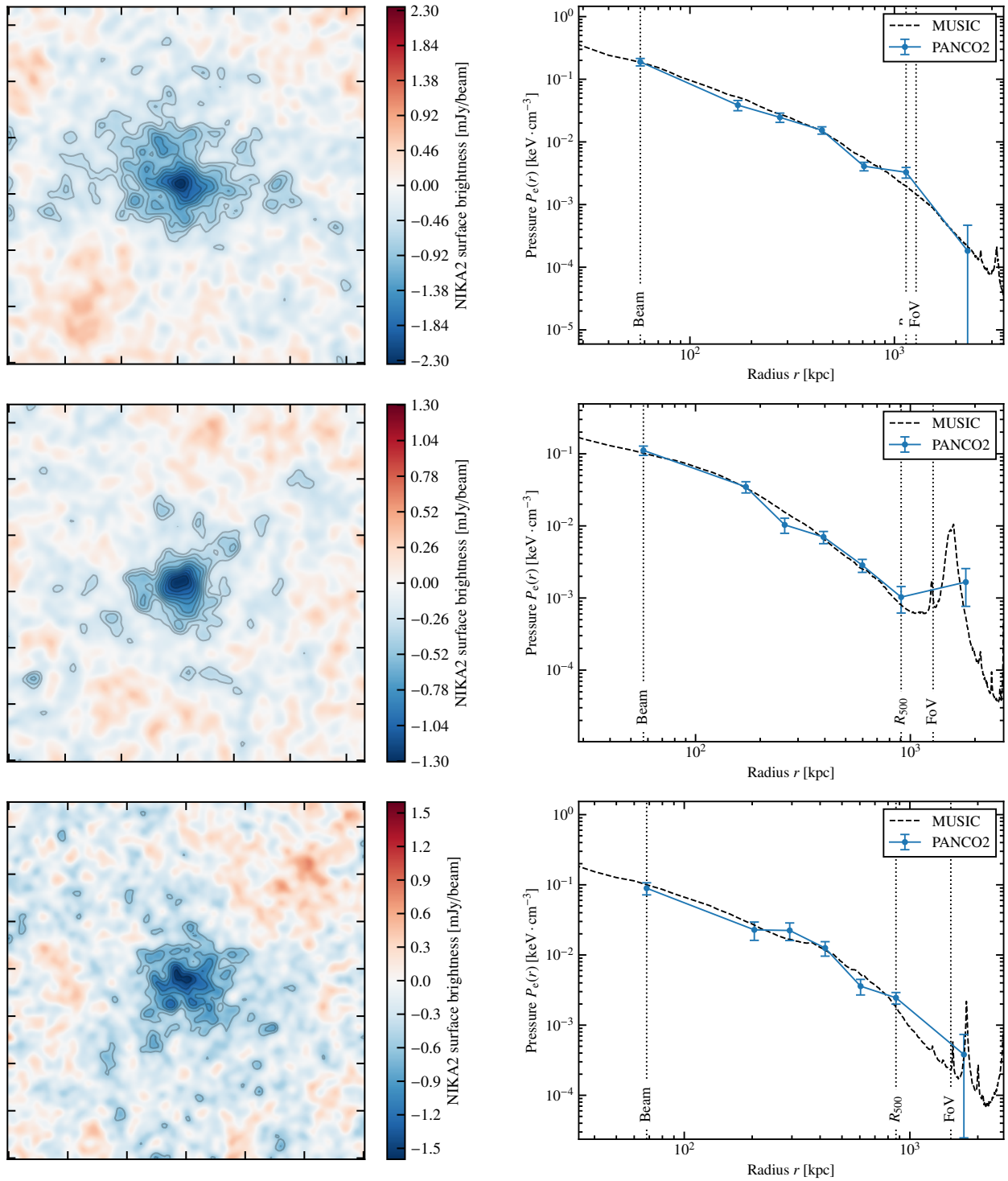
Figure 5.13 : Illustration des cartes NIKA2 simulées ( gauche ) et profils de pression mesurés ( droite ) pour trois amas MUSIC : deux à z = 0.54 ( haut, milieu ) et un à z = 0.82 ( bas ). La légende des cartes est la même que pour la figure 5.12. Les lignes pointillées noires représentent les profils de pression réels des amas tels qu’extraits de la simulation MUSIC. Les profils bleus sont ceux obtenus par ajustement avec PANCO2. Tous les profils sont centrés sur le pic de potentiel gravitationnel des amas tels que mesurés dans la simulation MUSIC.
