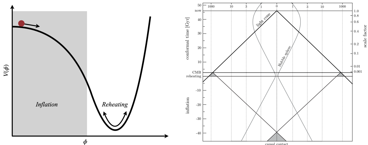
Figure 1.2 : Gauche : Exemple de comportement du champ d'inflaton illustrant les deux régimes de l'équation (1.16) : le champ commence en slow roll dans une région de potentiel élevé, puis se stabilise dans une région de bas potentiel, avec des oscillations rapides correspondant au reheating . Droite : Diagramme d'espace-temps illustrant le contact causal de régions opposées dans le CMB au début de l'inflation. Figure extraite de [29].
