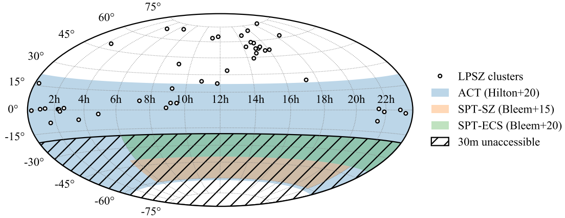
Figure 3.2 : Couvertures spatiales des relevés ACT (bleu, [3]) et SPT (orange et vert [4, 5]) en coordonnées équatoriales. Les axes horizontaux et verticaux représentent respectivement l'ascension droite et la déclinaison. La région hachurée marque les déclinaisons inaccessibles par le télescope de 30 mètres de l'IRAM. Les points représentent les coordonnées des amas du grand programme SZ de NIKA2 (voir section 3.4 page 65).
