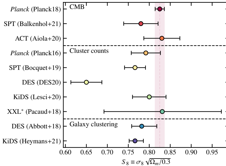
Figure 2.9 : Contrainte sur la combinaison de paramètres cosmologiques S_8 obtenues par différentes mesures du CMB (haut), de comptage d'amas (milieu), et de distribution de galaxies (bas). De haut en bas, les résultats sont issus de [14][119][120][101][100][104][108][103][121][122].
