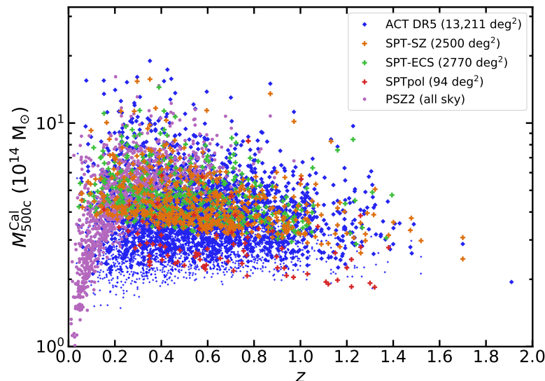
Figure 2.8 : Distribution dans le plan masse-redshift des amas détectés par les relevés ACT (bleu, [3]), SPT (orange [4], vert [5] et rouge [114]) et Planck (violet, [6]). Figure extraite de [3].
