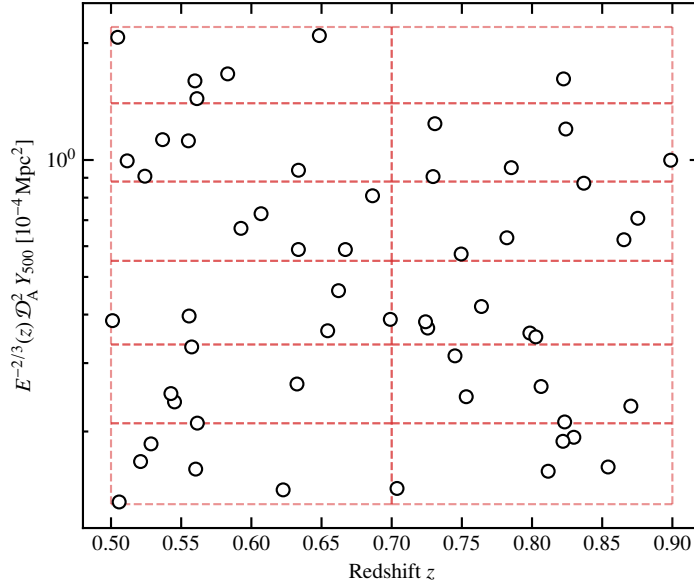
Figure 7.8 : Exemple d'échantillon combinant celui du grand programme SZ (voir figure 3.10) et une extension à basse masse. Deux boîtes (bas redshift et haut redshift) sont ajoutées correspondant à des faibles valeurs d'observable Y .
