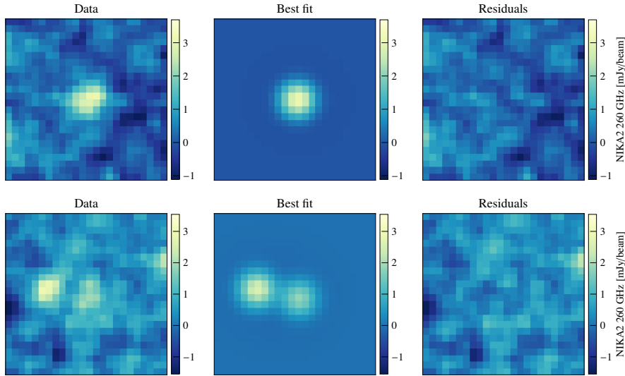
Figure 4.8 : Résultats d'un ajustement de source à 260 GHz pour une source simple ( haut ) et pour deux sources proches traitées comme double ( bas ) dans le champ de l'amas ACT-CL J0215.4+0030. De gauche à droite, les cartes représentent les données NIKA2 à 260 GHz, le modèle correspondant au meilleur ajustement, et la différence entre les deux cartes.
