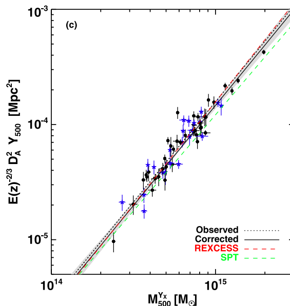
Figure 7.1 : Mesure de la relation d'échelle Y_{500} - M_{500} par la collaboration Planck . Chaque point représente un amas de galaxies. La relation ajustant le mieux les données est présentée en noir, et comparée aux relations issues des analyses de l'échantillon REXCESS en X (rouge, [95]) et SPT en SZ (vert, [189]). Figure extraite de [148].
