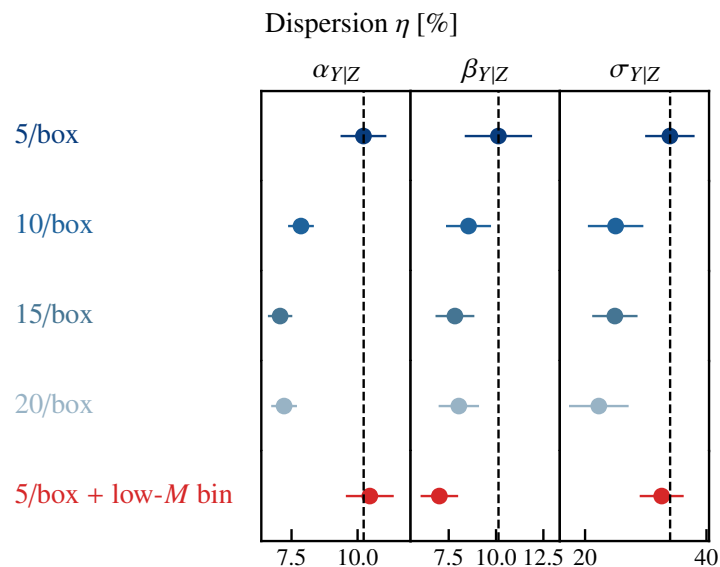
Figure 7.7 : Évolution de l'incertitude relative sur les paramètres d'intérêt avec les extensions du grand programme SZ : ajout d'amas avec la même fonction de sélection (bleu) et ajout d'amas de 10 amas de basse masse (rouge).
