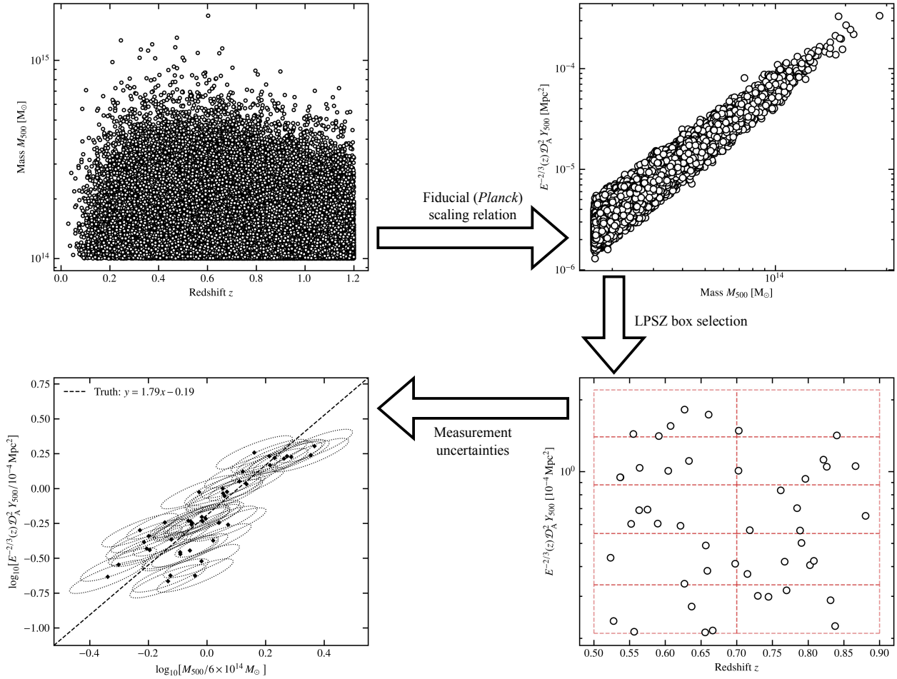
Figure 7.3 : Procédure de génération d'un échantillon d'amas similaire à celui du LPSZ. Un échantillon de halos est généré aléatoirement dans le plan (M_{500}, z) à partir d'une fonction de masse donnée ( haut gauche ). Une relation d'échelle fiducielle est utilisée pour obtenir des valeurs d'observable SZ correspondantes ( haut droit ). Une sélection similaire à celle du LPSZ sur les valeurs d'observable SZ est réalisée pour obtenir un échantillon de 50 amas ( bas droit ). Des incertitudes de mesure corrélées sur la masse et sur l'observable sont ensuite générées ( bas gauche ). L'ellipse autour de chaque point représente l'intervalle 1\sigma de la gaussienne à deux dimensions utilisée comme incertitude.
