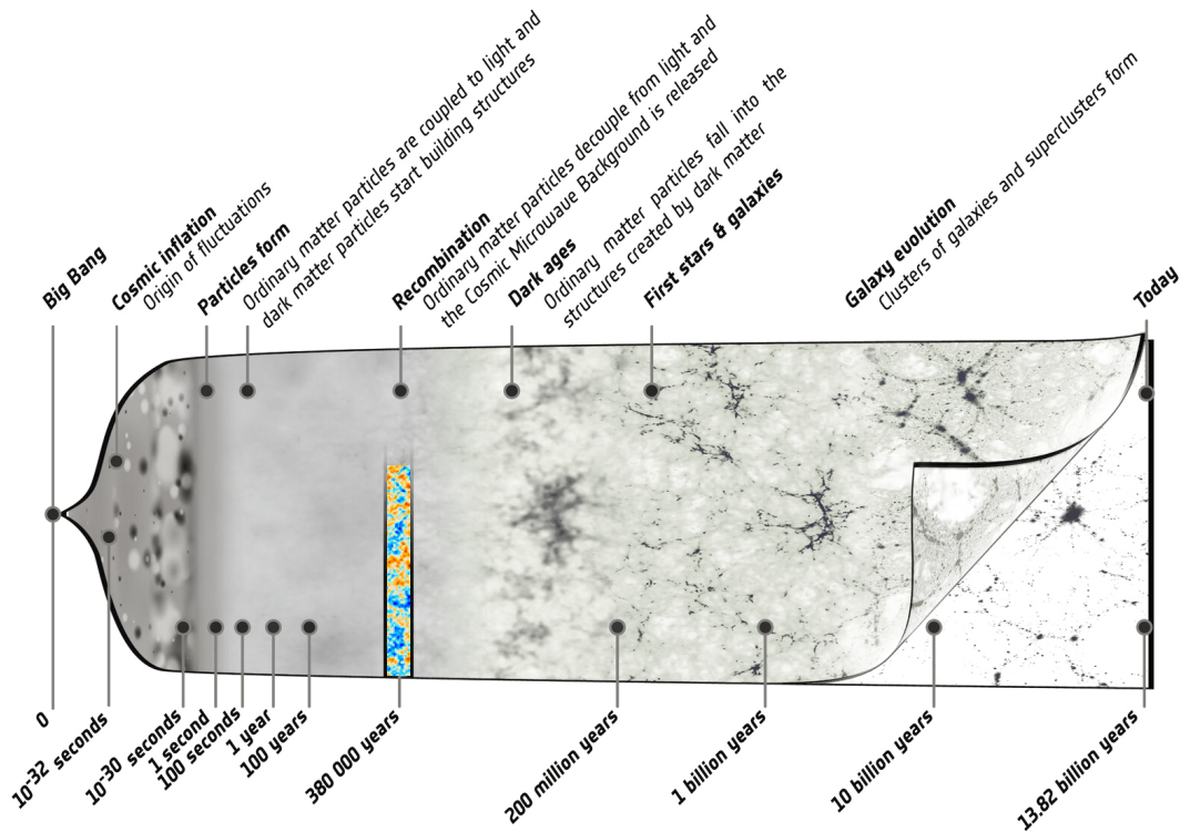
Figure 1.1 : Résumé des étapes de l'histoire thermique de l'Univers, du Big Bang à aujourd'hui. Crédit : ESA – C. Carreau
