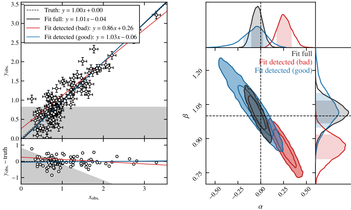
Figure 7.2 : Illustration du biais de Malmquist dans l'ajustement d'une relation d'échelle. Gauche : représentation des données et des relations d'échelles ajustées dans le plan (x, y) ( haut ) et résidus autour de la relation d'échelle réelle ( bas ). Droite : intervalles de confiance à 1\sigma et 2\sigma dans le plan (\alpha, \beta) obtenus par régression. Voir texte pour le détail des différentes régressions.
