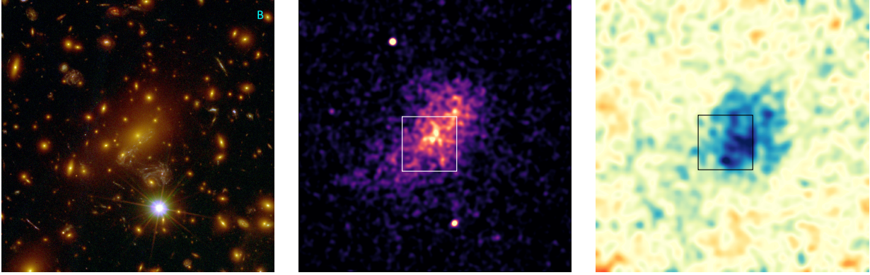
Figure 2.2 : Cartographie de l’amas de galaxies MACSJ1149.5+2223 par le Hubble Space Telescope en optique et infrarouge ( gauche , extraite de [59]), en X avec Chandra ( centre ), et en millimétrique par l’effet Sunyaev-Zeldovich avec NIKA2 ( droite ). La taille de la région cartographiée est de 1 arcmin pour la carte optique, et de 5 arcmin pour les cartes X et SZ. La région cartographiée en optique est représentée par un carré sur les cartes X et SZ.
