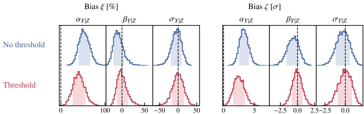
Figure 7.5 : Biases \xi et \zeta sur les paramètres d'intérêt de la relation d'échelle pour une dispersion intrinsèque deux fois supérieure à celle supposée par Planck ( \sigma_{Y|Z} = 0.15 ). La légende est identique à celle de la figure 7.4.
