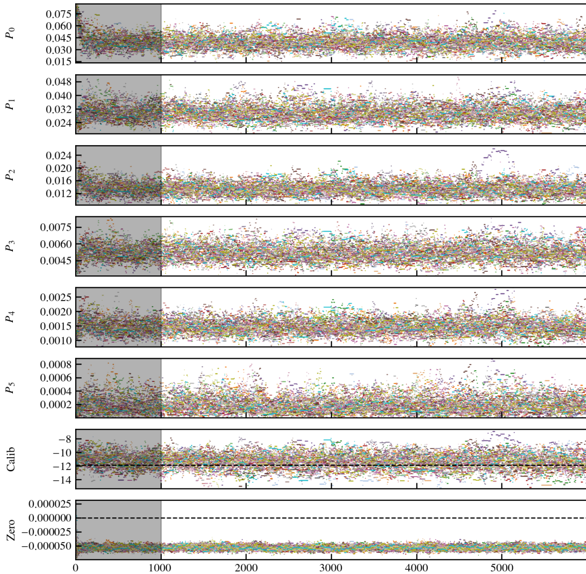
Figure 5.5 : Évolution des chaînes de Markov dans l'espace des paramètres avec le nombre de pas. Chaque couleur représente une chaîne distincte. La région grise correspond au burn-in retiré pour l'analyse. Les lignes noires pointillées correspondent aux vraies valeurs du coefficient de conversion et du niveau zéro de la carte.
