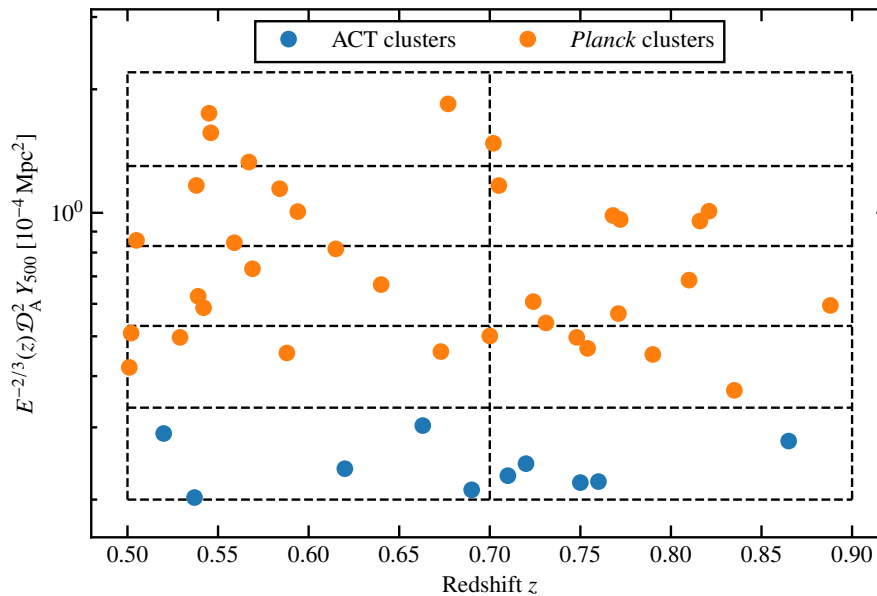
Figure 3.10 : Distribution des amas du grand programme SZ dans le plan redshift – paramètre de Compton intégré. Les points bleu et orange représentent respectivement les amas extraits des catalogues ACT [136] et Planck [6]. Les lignes noires pointillées représentent les limites des boites utilisées pour construire l'échantillon.
