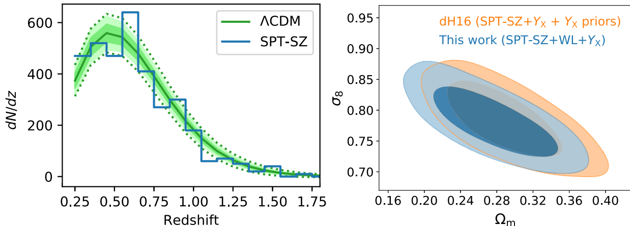
Figure 2.7 : Gauche : Comptage d'amas par intervalles de redshift dans le relevé SPT-SZ 2500 deg 2 (bleu) et résultats de l'ajustement du modèle de l'équation (2.24) (vert). Droite : Intervalles de confiance à 1\sigma et 2\sigma obtenus sur les paramètres ( \Omega_m, \sigma_8 ) par l'ajustement représenté dans le panneau gauche (bleu). L'ellipse orange montre les résultats de l'étude antérieure de [102] pour comparaison. Figures adaptées de [100].
