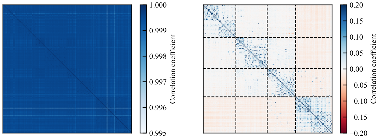
Figure 4.2 : Matrice de corrélation entre les TOI des détecteurs de la matrice NIKA2 à 150 GHz lors d'une observation d'Uranus. Gauche : Corrélations des données brutes, avant soustraction d'un mode commun. Droite : Corrélations après soustraction d'un mode commun calculé à partir de tous les détecteurs de la matrice. Les lignes noires pointillées délimitent les détecteurs appartenant à chacune des quatre boîtes de l'électronique de lecture de NIKA2.
