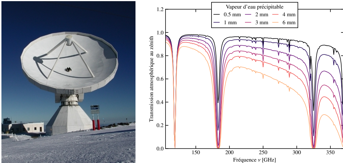
Figure 3.1 : Gauche : Photo du télescope de 30 mètres de l'IRAM. Crédit : IRAM . Droite : spectre de transmission atmosphérique en fonction de la quantité de vapeur d'eau précipitable, d'après le modèle de Pardo et al. [127].
