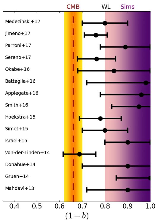
Figure 2.1 : Estimation du biais hydrostatique par comparaison de mesures de masse hydrostatique et par lentillage faible (voir section 2.2.1) pour différentes études (noir). La valeur nécessaire pour concilier les résultats du CMB et des amas de galaxies, mesurée par [52], est indiquée en orange. La région violette représente les valeurs de (1-b) permises par plusieurs analyses d'amas simulés [53]. Figure extraite de [52].
