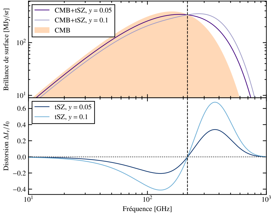
Figure 2.3 : Haut : Spectre des photons du CMB (orange) et de photons ayant interagi avec un amas pour deux valeurs de paramètres de Compton y (violet). Au premier ordre, l'effet tSZ représente un décalage du spectre vers les grandes fréquences. Bas : Distorsion spectrale due à l'effet tSZ pour les mêmes valeurs de paramètre de Compton. La signature observationnelle de l'effet tSZ apparaît comme un décrétement dans la brillance de surface du CMB aux fréquences inférieures à 217 GHz (ligne noire verticale), et un incrément au-delà. Les valeurs de paramètre de Compton utilisées sont grandement exagérées pour des raisons visuelles. Les corrections relativistes à l'effet tSZ sont négligées.
