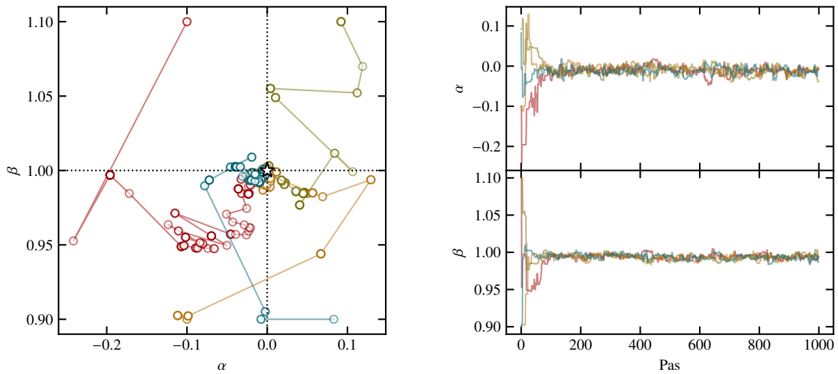
Figure 5.3 : Illustration du mouvement des chaînes d'un échantillonneur MCMC dans le cas d'une régression à deux paramètres (\alpha, \beta) , dans l'espace des paramètres ( gauche ) et projeté pour chacun des paramètres individuellement ( droite ). Chaque couleur représente une chaîne de Markov. L'étoile dans le panneau gauche représente le maximum de la distribution postérieure considérée.
