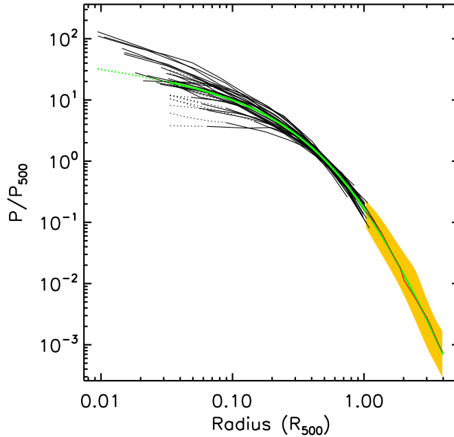
Figure 2.6 : Profils de pression des amas de galaxies de l'échantillon REXCESS mesurés par XMM-Newton (noir) et profil de pression moyen de l'échantillon, dit universel (vert). Figure extraite de [95].
