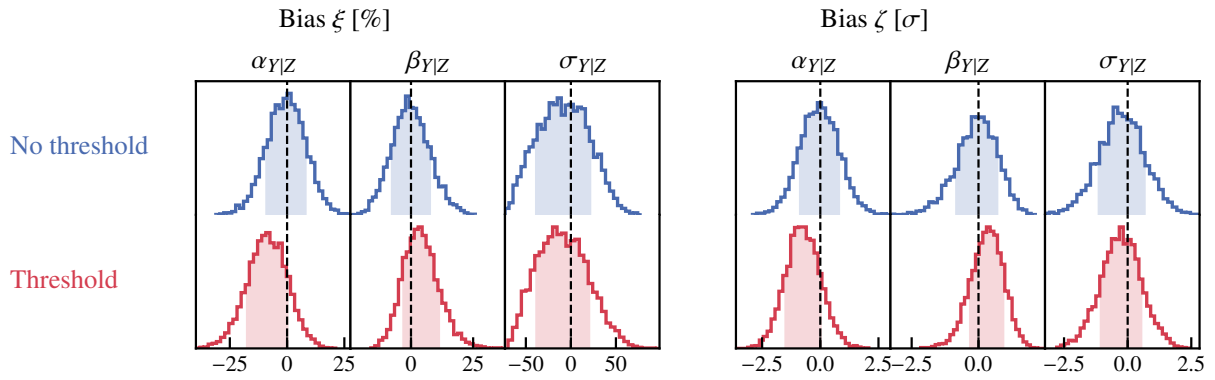
Figure 7.4 : Distribution des biais \xi (gauche) et \zeta (droite) sur les trois paramètres d'intérêt de la relation d'échelle pour les 5000 réalisations d'échantillons. Les ajustements sont réalisés sans tenir compte de coupure en observable (bleu) et en tenant compte d'une coupure à Y_{low} (rouge). Les régions colorées correspondent aux intervalles de confiance à 1\sigma .
