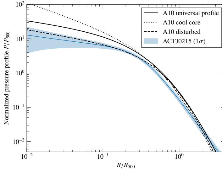
Figure 6.10 : Comparaison du profil de pression obtenu à partir des données NIKA2 (bleu) avec les profils moyens de Arnaud et al. [95] (noir). ACT-CL J0215.4+0030 présente un profil similaire aux amas identifiés comme ayant un cœur perturbé (ligne noire pointillée).
