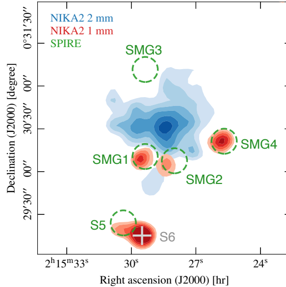
Figure 6.5 : Carte composite multifréquence de la région de l'amas. Les niveaux de bleu correspondent aux niveaux de signal sur bruit du décrément SZ dans la carte NKA2 à 150 GHz, commençant à 3\sigma et espacés de 1\sigma . De même, les niveaux de rouge correspondent au signal sur bruit des sources ponctuelles dans la carte NKA2 à 260 GHz. Les cercles verts sont centrés sur les positions des sources dans le catalogue HerS82 [178] et leur diamètre est la FWHM du lobe instrumental de SPIRE à 250 \mu\text{m} . La croix grise marque la position de S6, la source identifiée par NKA2 qui n'a pas de contrepartie dans le catalogue HerS82.
