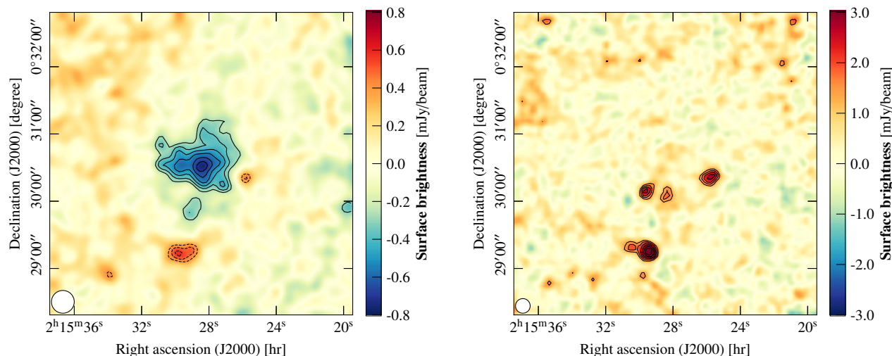
Figure 6.3 : Cartes NIKA2 du champ de l'amas à 150 GHz ( gauche ) et 260 GHz ( droite ). Chaque carte est montrée dans un champ carré de 4.5' \times 4.5' centré sur les coordonnées observées. Dans chacune des cartes, les contours noirs montrent les niveaux de signal sur bruit commençant à 3\sigma et espacés de 1\sigma . Les cartes de gauche et droite sont lissées avec un noyau Gaussien de 10'' et 6'' respectivement pour des raisons visuelles. Pour chaque carte, la FWHM de sa résolution effective est illustrée par un disque blanc en bas de la carte.
