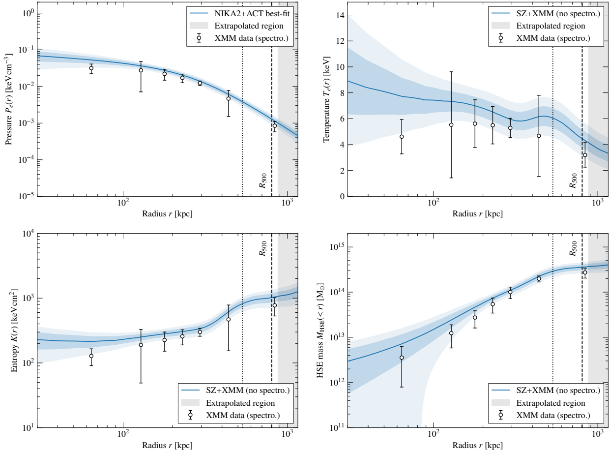
Figure 6.9 : Profils radiaux de la pression ( haut gauche ), température ( haut droit ), entropie ( bas gauche ), et masse hydrostatique ( bas droit ) du milieu intra-amas de ACT-CL J0215.4+0030. Pour le profil de pression, la courbe bleue représente le profil de pression correspondant au meilleur ajustement des données NIKA2. Pour les autres profils, elle montre la combinaison entre ce profil de pression et le profil de densité obtenue avec XMM-Newton . Les enveloppes bleues montrent les intervalles de confiance à 1\sigma et 2\sigma sur ces profils. Les points blancs représentent les profils obtenus en combinant les profils de densité et de température mesurés en X, avec des erreurs à 1\sigma . La ligne noire en pointillés montre la limite à l'intérieur de laquelle le rapport signal sur bruit sur le profil de brillance de surface de la carte NIKA2 à 150 GHz est supérieur à 3\sigma . La zone grisée représente la région dans laquelle les profils ne sont pas contraints par les données SZ, c'est-à-dire au delà de R_{500}^{\text{ACT}} .
