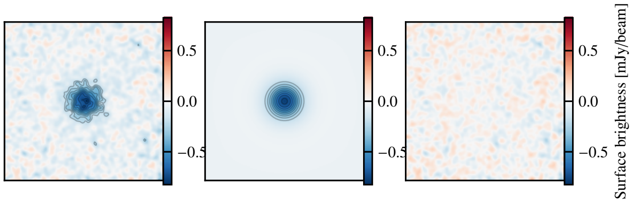
Figure 5.4 : Carte simulée de ACT-CL J0215.4+0030 ( gauche ), carte de modèle ajustée par PANC02 ( centre ), et différence entre les deux cartes ( droite ). La région représentée est la même pour les trois cartes, et représente un carré de 5' de côté centré sur le centre simulé de l'amas. Les contours gris sont les niveaux de signal-sur-bruit, commençant à 3\sigma et espacés de 1\sigma .
