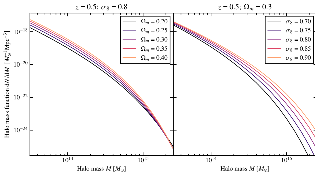
Figure 1.3 : Illustration de l'évolution de la fonction de masse avec les paramètres cosmologiques. La fonction de masse de Tinker et al. [33] est représentée pour différentes valeurs de \Omega_m (gauche), et de \sigma_8 (droite). Le redshift est fixé à z = 0.5 .
