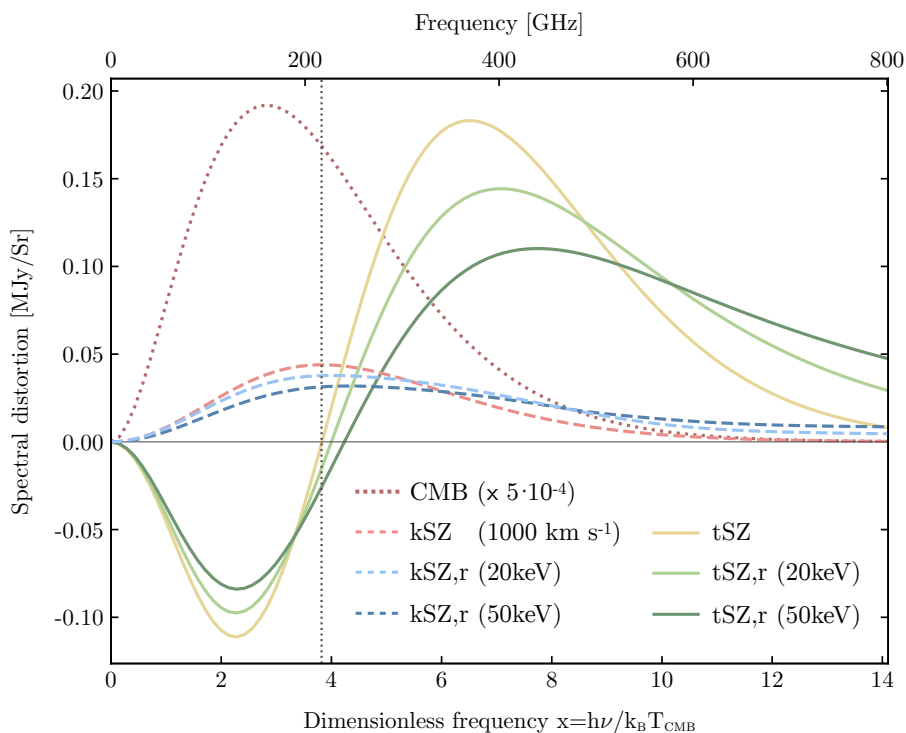
Figure 2.5 : Spectres de l'effet tSZ (courbes pleines) et kSZ (courbes pointillées), incluant les corrections relativistes pour différentes valeurs de température. La profondeur optique considérée est de \tau_e = 10^{-2} . Le spectre des photons du CMB sans interaction par effet SZ est également représenté en rouge pour comparaison. Figure extraite de [81].
