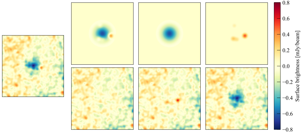
Figure 6.8 : Résultats de l’ajustement de la carte NIKA2 à 150 GHz de ACT-CL J0215.4+0030 (panneau de gauche). Le modèle ajustant le mieux les données et les résidus sont respectivement montrés dans les panneaux haut et bas de la colonne du centre gauche. Les colonnes de centre droit et droite représentent le meilleur modèle et les résidus en considérant seulement le signal SZ et les sources ponctuelles, respectivement. Les cartes sont représentées dans la même région et lissées par le même filtre que dans la figure 6.3. Les deux sources dans le sud de la carte (S5 et S6) ont été soustraites.
