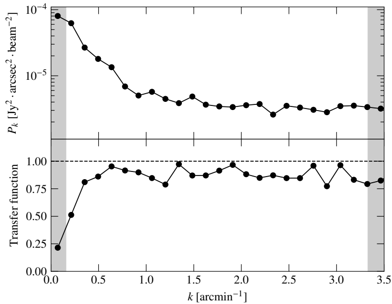
Figure 6.2 : Spectre de puissance du bruit résiduel ( haut ) et fonction de transfert ( bas ) correspondant à l'analyse des observations de ACT-CL J0215.4+0030 avec NIKA2. La procédure d'obtention est décrite dans 4.4. Le spectre de puissance montre un bruit résiduel corrélé à grande échelle, et la fonction de transfert montre le filtrage du signal aux grandes échelles angulaires.
