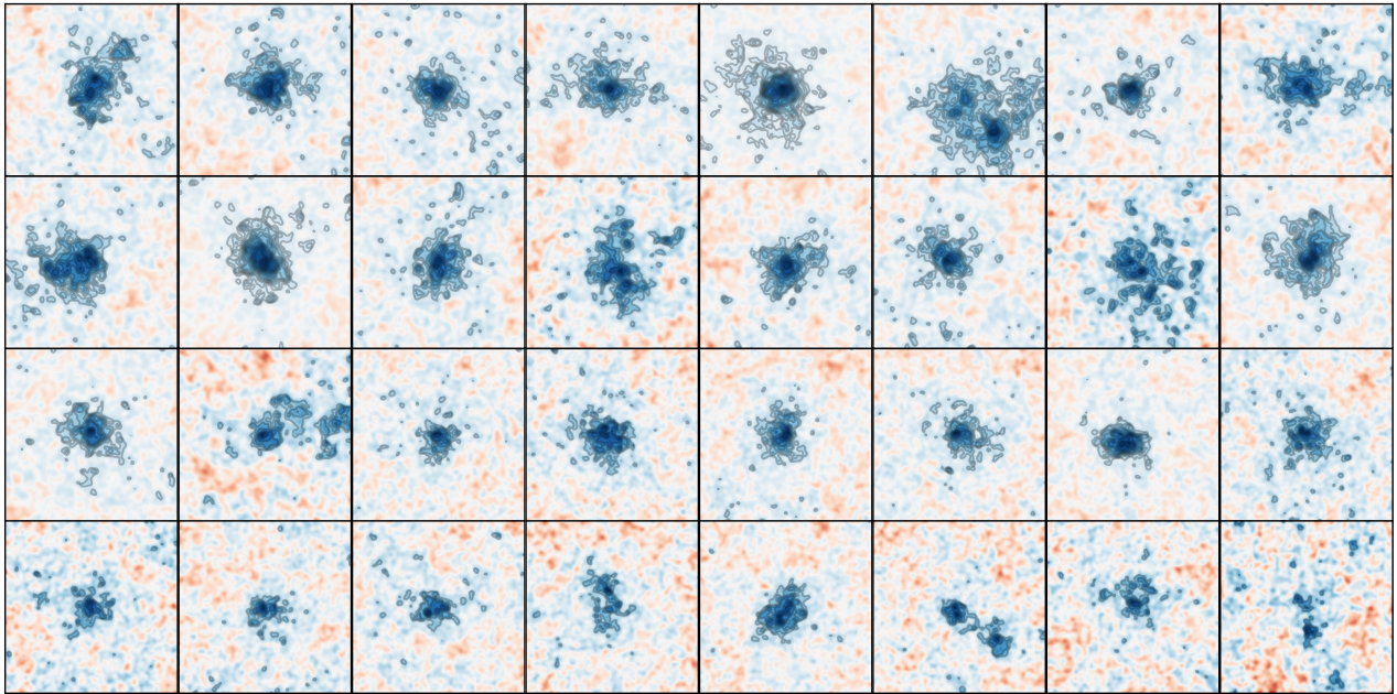
Figure 5.12 : Cartes simulées des 32 amas de l'échantillon utilisé pour la validation du code. Les échelles de couleurs sont arbitraires. Chaque carte est représentée dans un carré de 6.5' de côté, centré aux coordonnées du pic de densité du halo considéré. Les contours représentent les niveaux de signal sur bruit commençant à 3\sigma espacés de 1\sigma . Les cartes sont lissées par un noyau gaussien de largeur à mi-hauteur 10'' pour des raisons visuelles.
