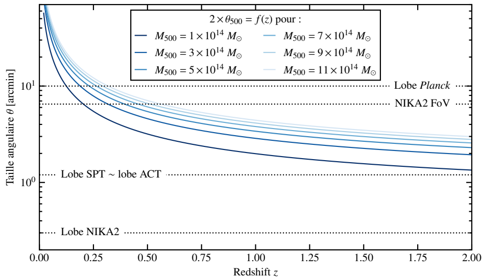
Figure 3.9 : Évolution du diamètre angulaire caractéristique 2\theta_{500} d'amas de galaxies de différentes masses avec le redshift. Les lobes de NIKA2 ( \sim 18'' à 150 GHz), SPT ( \sim 1.2' ), ACT ( \sim 1.4' ), et Planck ( \sim 10' ) sont représentés à titre indicatif, de même que le champ de vue instantané (FoV pour field of view ) de NIKA2 ( 6.5' ).
