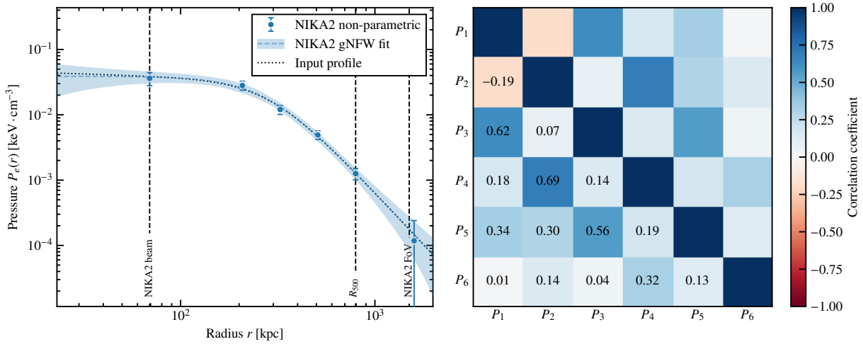
Figure 5.7 : Gauche : Profil de pression obtenu avec PANC02. Les points bleus représentent le meilleur ajustement en non-paramétrique. L’enveloppe bleue représente l’incertitude sur ce profil obtenue par interpolation gNFW des résultats non-paramétriques. La courbe pointillée noire est le profil de pression utilisé pour générer la carte de l’amas. Droite : Matrice de corrélation entre les points du profil de pression, obtenue à partir des chaînes de Markov.
