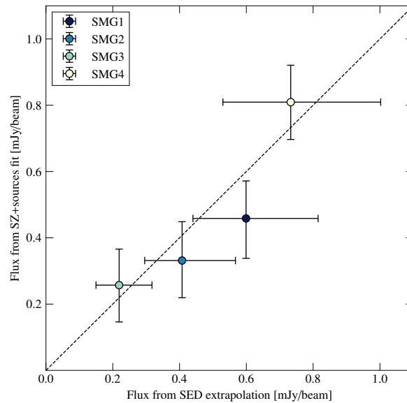
Figure 6.7 : Comparaison des densités de flux des sources ponctuelles estimées par extrapolation de SED (abscisse) et par l'analyse jointe SZ-sources ponctuelles avec un a priori uniforme sur les flux (ordonnée, voir section 6.3.3). Les barres d'erreur représentent les 16èmes et 84èmes percentiles des distributions. Les deux estimateurs sont compatibles dans ces barres d'erreur pour chacune des sources.
