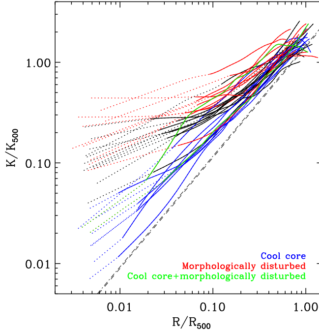
Figure 3.11 : Profils d'entropie mesurés à partir des observations XMM-Newton des amas de l'échantillon REXCESS. Les lignes pointillées noires marquent le profil en r^{-1.1} attendu pour une formation d'amas purement par effondrement gravitationnel. Les courbes bleues et rouges sont respectivement les profils d'amas classifiés comme cool-core et à cœur perturbé. Figure extraite de [112].
