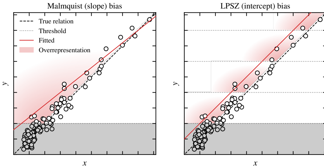
Figure 7.6 : Illustration de la cause du biais sur l'ordonnée à l'origine. Pour une coupure en observable ( gauche ), une surreprésentation de points au dessus du seuil (région rouge) entraîne une rotation de la relation d'échelle ajustée (droite rouge), et donc un biais sur la pente. Pour une sélection en boîtes comme celle du LPSZ ( droite ), des coupures correspondant aux seuils des boîtes créent des surreprésentations au dessus de ces seuils. Le résultat est un décalage de la relation d'échelle ajustée, correspondant à un biais sur l'ordonnée à l'origine.
