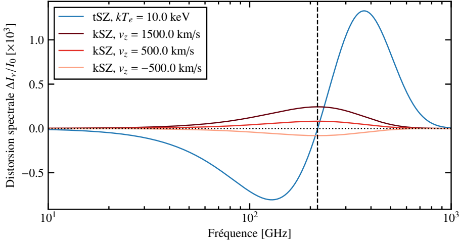
Figure 2.4 : Signatures spectrales de l'effet tSZ (bleu) et kSZ (rouge) pour un amas de profondeur optique \tau_e = 10^{-2} . L'amplitude de l'effet tSZ est calculée en supposant un milieu intra-amas isotherme avec k_B T_e = 10 keV. Les amplitudes pour l'effet kSZ sont calculées pour différentes valeurs de vitesse le long de la ligne de visée. Dans les deux cas, les corrections relativistes sont négligées.
