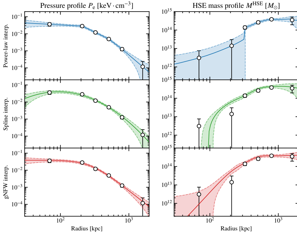
Figure 5.9 : Gauche : Interpolations possible du profil de pression non-paramétrique (points blancs) pour un amas simulé : interpolation en loi de puissance (bleu), en splines (vert), et en gNFW (rouge). La ligne continue montre le profil correspondant à l’interpolation du profil de pression ajustant le mieux les données Droite : Profils de masse hydrostatique obtenus par combinaison des profils de pression SZ et de densité X pour les trois méthodes d’interpolation. La ligne continue montre le profil correspondant au profil de masse obtenu à partir du profil de pression interpolé à partir du meilleur ajustement. Les régions colorées correspondent aux intervalles de confiance à 1\sigma sur les profils.
