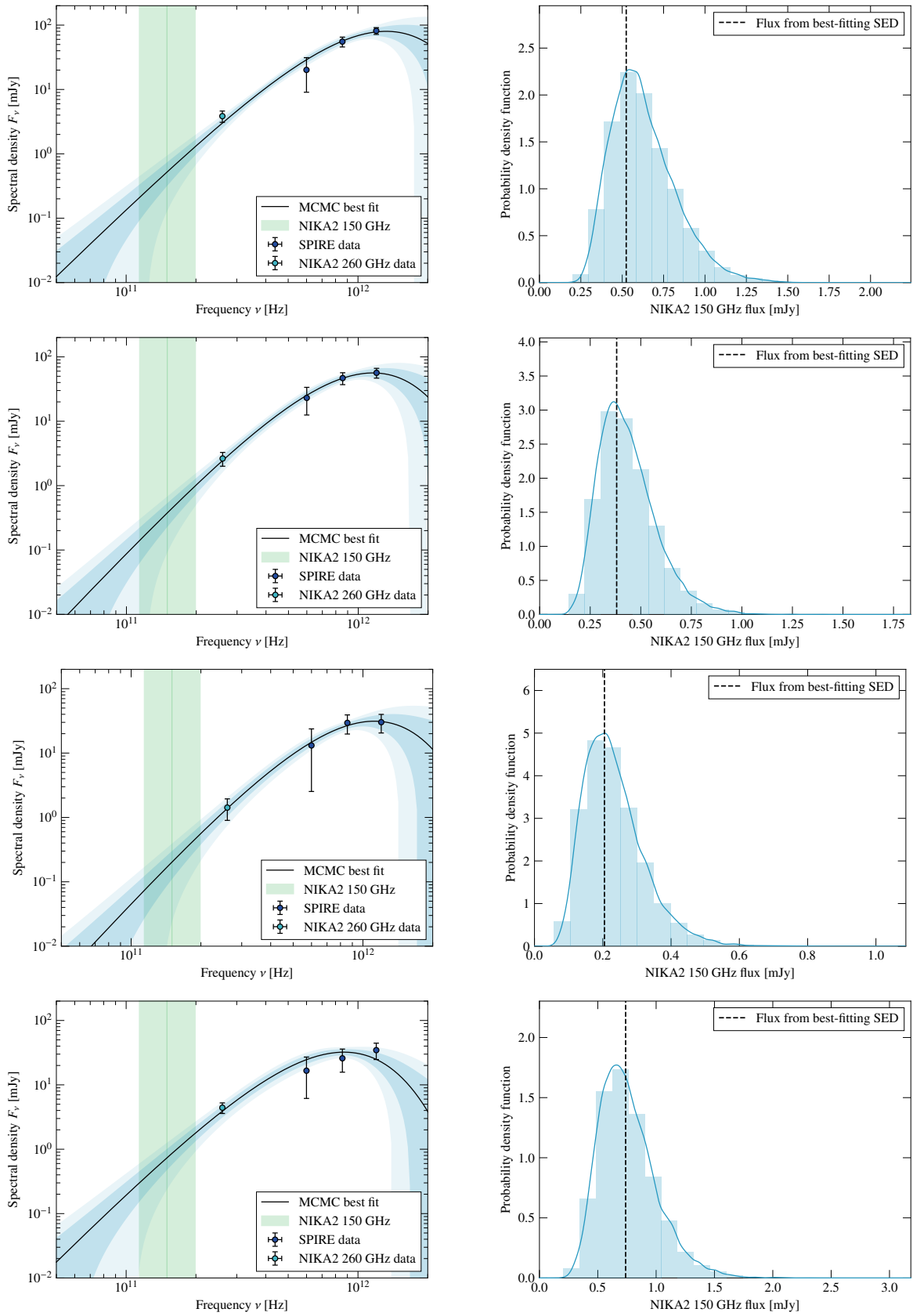
Figure 6.6 : De haut en bas, résultats de PSTools pour les sources SMG1 à SMG4 dans le champ de l'amas ACT-CL J0215.4+0030. Gauche : ajustement de la SED sur les flux SPIRE (bleu foncé) et NIKA2 à 260 GHz (bleu clair). La région verte correspond à la bande passante de NIKA2 à 150 GHz. Les régions bleues correspondent aux intervalles de confiance à 1\sigma et 2\sigma sur l'ajustement de la SED. Droite : distribution de probabilité du flux à 150 GHz. L'histogramme représente les flux obtenus pour les chaînes de Markov, et la courbe bleue est la distribution de probabilité résultante.
