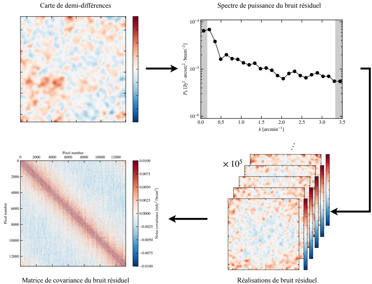
Figure 4.5 : Illustration du calcul de la matrice de covariance du bruit résiduel pour la décorrélation common mode one block de l'amas PSZ2-G183.90+42.99 (voir figure 4.3). La carte de demi-différences ( haut gauche ) est utilisée pour calculer le spectre de puissance du bruit résiduel ( haut droit ), à son tour utilisé pour générer des réalisations de bruit corrélé de même spectre de puissance ( bas droit ). La covariance de ces réalisations donne la matrice de covariance pixel-à-pixel du bruit résiduel ( bas gauche ).
