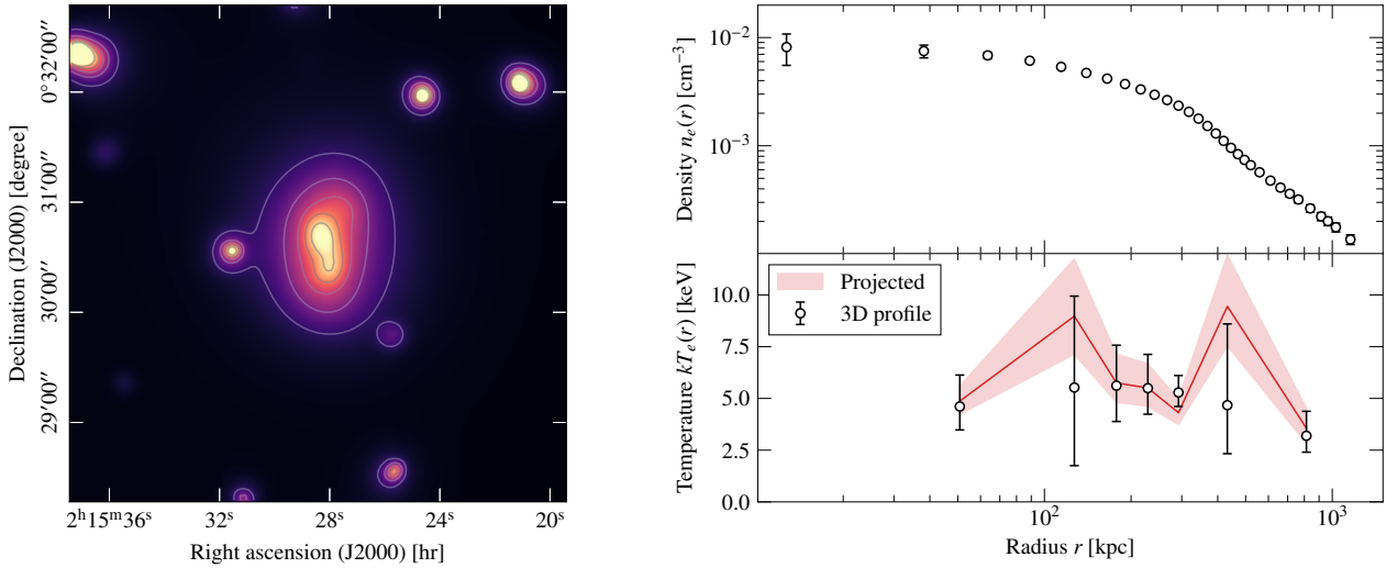
Figure 6.4 : Gauche : Carte d'évènements XMM-Newton lissée par ondelettes. La région montrée est la même que dans la figure 6.3. Les iso-contours sont montrés en gris. Droite : Profils de densité ( haut ) et température ( bas ) électronique extraits à partir des observations XMM de l'amas. Les profils sont extraits aux coordonnées du pic SZ, comme décrit dans le texte (6.1.3). Les barres d'erreur montrent les incertitudes à 1\sigma . Pour le profil de température, la ligne rouge représente le profil projeté, tandis que les points blancs représentent le profil 3D reconstruit ; pour une explication détaillée de la différence entre les deux quantités, voir [112].
