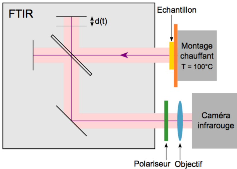
FIGURE 3.9 – Schéma du montage expérimental pour la caractérisation de l'emissivité. L'échantillon est porté à une température de 150°C, son émission est analysée par le FTIR et sa polarisation TM ajustée à l'aide d'un polariseur.
