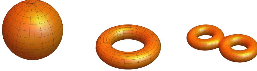
FIGURE 1: Variétés topologiques avec différents genres g . A gauche : Une sphère avec g = 0 . Au milieu : Un tore avec g = 1 . A droite : Un tore double avec g = 2 .
