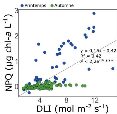
Figure E3.3. Amplitude du NPQ en fonction de la DLI. Les données de l'expérience de Printemps et d'Automne sont représentées en bleu et en vert, respectivement. La droite en noir représente la régression linéaire de type II.
