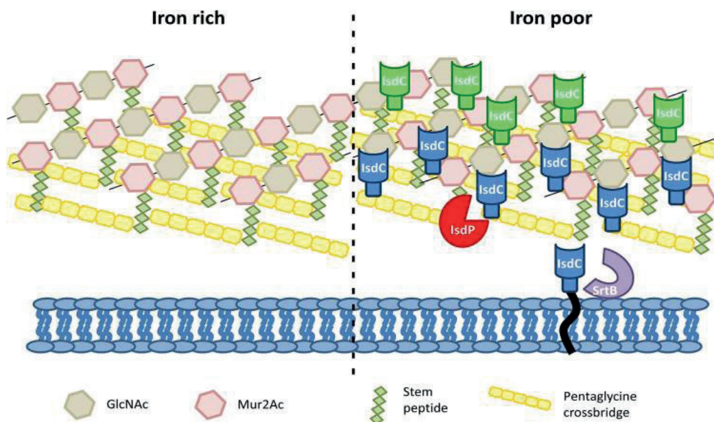
Figure 58 : Modèle de contribution de la protéine IsdP à l'acquisition d'hème chez S. lugdunensis .
