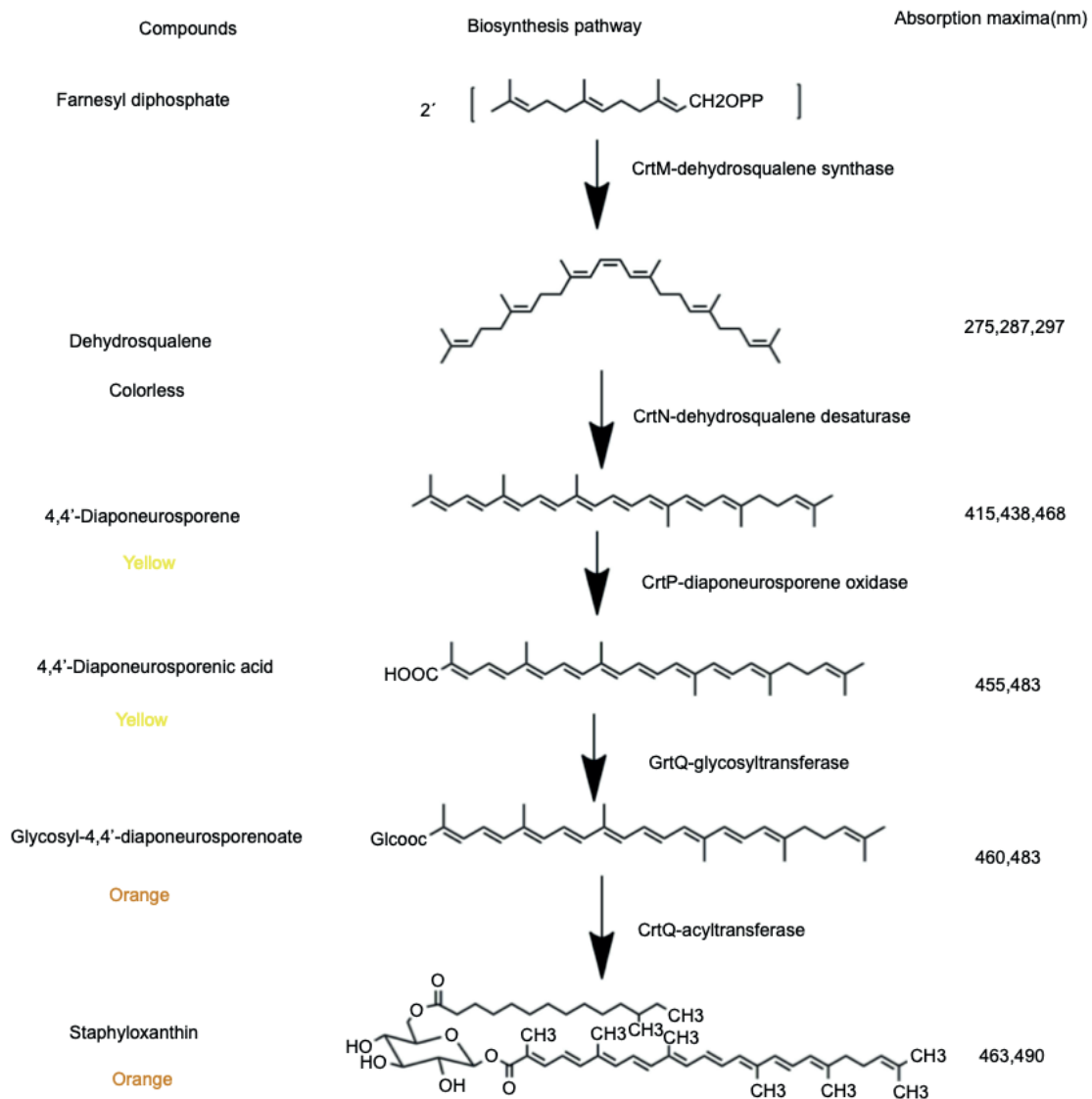
Figure 33 : La voie de la biosynthèse de la staphyloxanthine.
