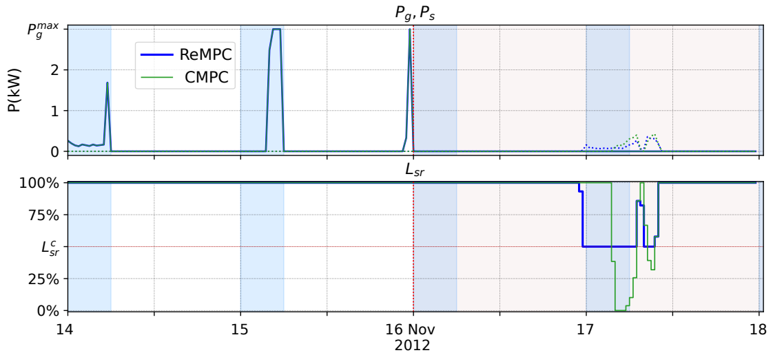
Figure A.9 – ReMPC (bleue) vs CMPC (verte), panne planifiée : Courbes d'évolution de P_g, P_s (1 ère sous figure) et de L_{sr} (2 nd sous figure) pour 4 jours de simulation
