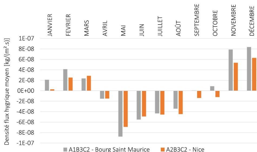
Figure 5.33 - Moyenne mensuelle de la densité de flux hygrique à travers la surface intérieure du mur bicouche béton + HB-S – Bourg Saint Maurice et Nice.
