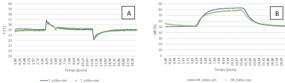
Figure 5.11 - Comparaison de la température (A) et de l'humidité relative (B) au milieu du matériau simulée et mesurée expérimentalement – C1-H.
