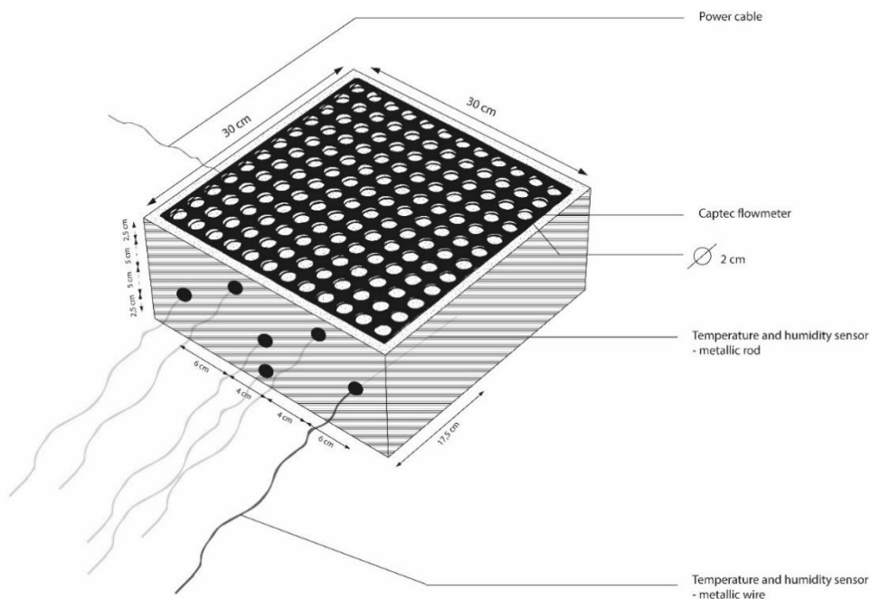
Figure 6.2 - Instrumentation pour le test du fluxmètre perforé en cuivre.
