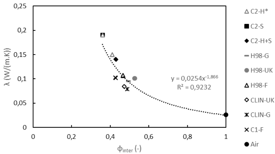
Figure 3.16 - Comparaison de la conductivité thermique et la porosité intergranulaire des bétons.
