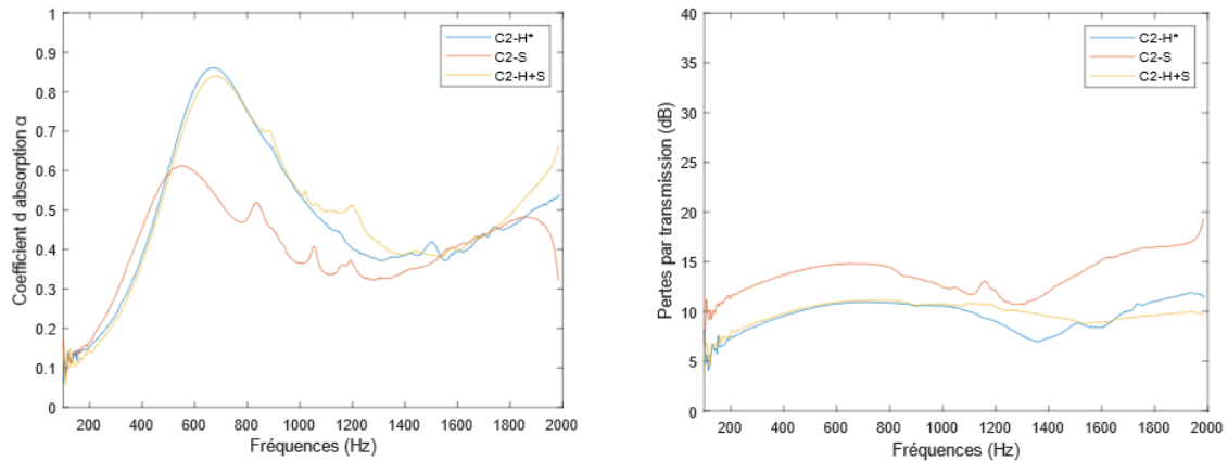
Figure 3.10 - Coefficient d'absorption acoustique et pertes par transmission des bétons C2-H*, C2-S et C2-H+S.
