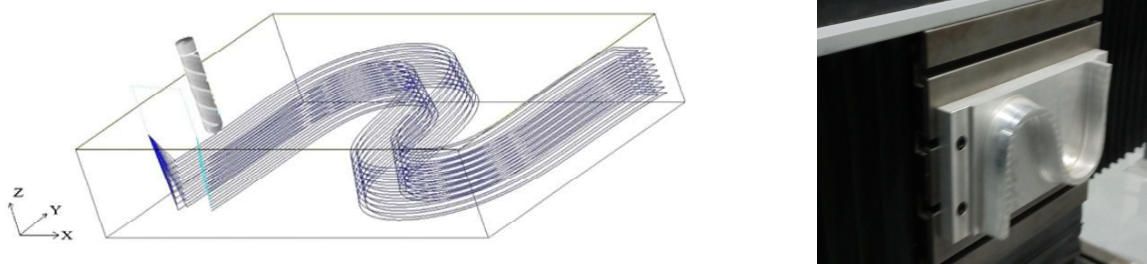
FIGURE 2.6 – Trajectoire d'usinage proposée dans Zhu et al. [2011] et pièce réalisée par l'Université de Tianjin
