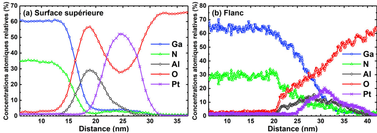
Figure 3-23 : profils de concentrations des différents atomes d'intérêt effectués à l'aide d'une imagerie STEM-EDS (a) sur le haut de la méso et (b) sur le flanc à l'interface avec une zone GaN.
