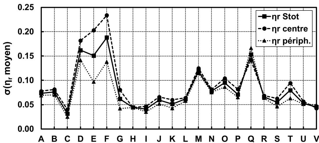
Figure D-4 : écart-type pour l'efficacité relative \eta_r moyenne sur les N mésas scannées par échantillon (Stot : toute la surface supérieure de la méso).
