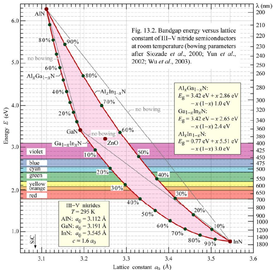
Figure 1-11 : dépendance entre énergie de gap et paramètre a de la maille cristalline, pour des alliages entre du GaN et de l'InN (InGaN) ou de l'AlN (AlGaIn) [15].
