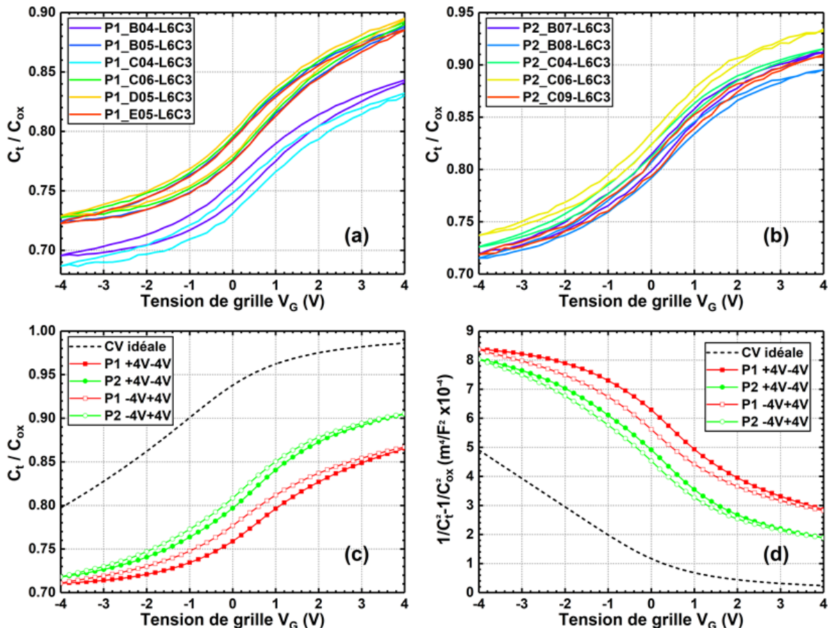
Figure 4-13 : exemples d'hystérésis C-V pour les condensateurs L6C3 sur (a) P1 et (b) P2 ; moyennes de l'ensemble des mesures C-V normalisées (c) tracées en C_t/C_{ox} et (d) tracées en 1/C_t^2 - 1/C_{ox}^2 en fonction de V_G .
