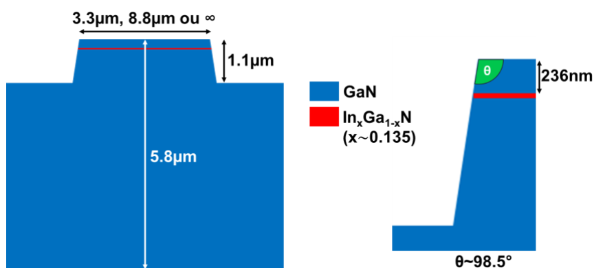
Figure 5-15 : vue en coup schématique des structures simulées.
