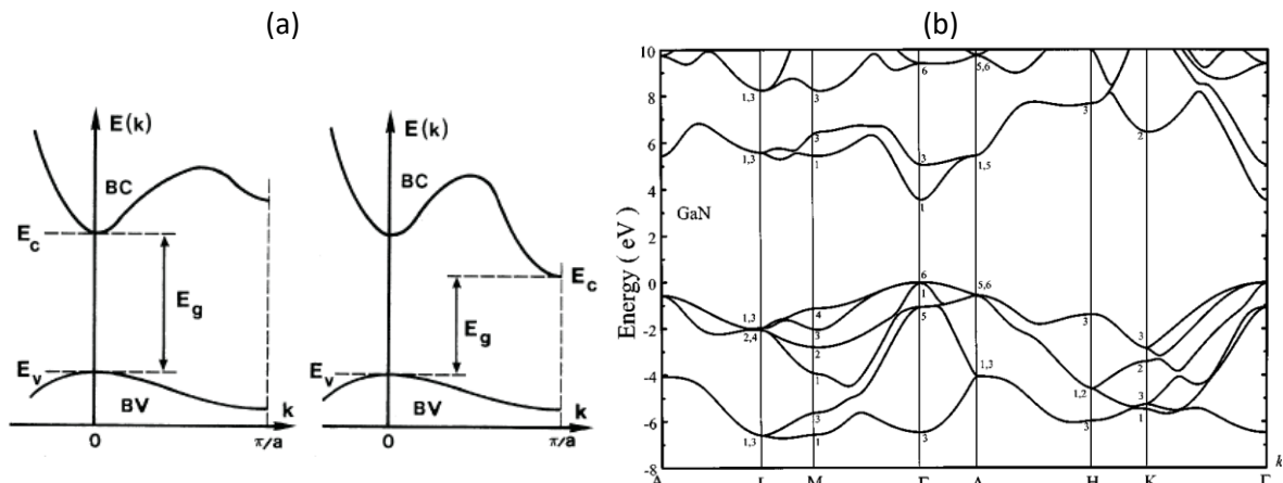
Figure 1-5 : (a) courbes de dispersion E(k) pour les électrons dans un semiconducteur à gap direct (à gauche) et à gap indirect (à droite) [12] et (b) structure des bandes électroniques du GaN wurtzite selon les directions de hautes symétries de la première zone de Brillouin dans l'espace réciproque [13].
