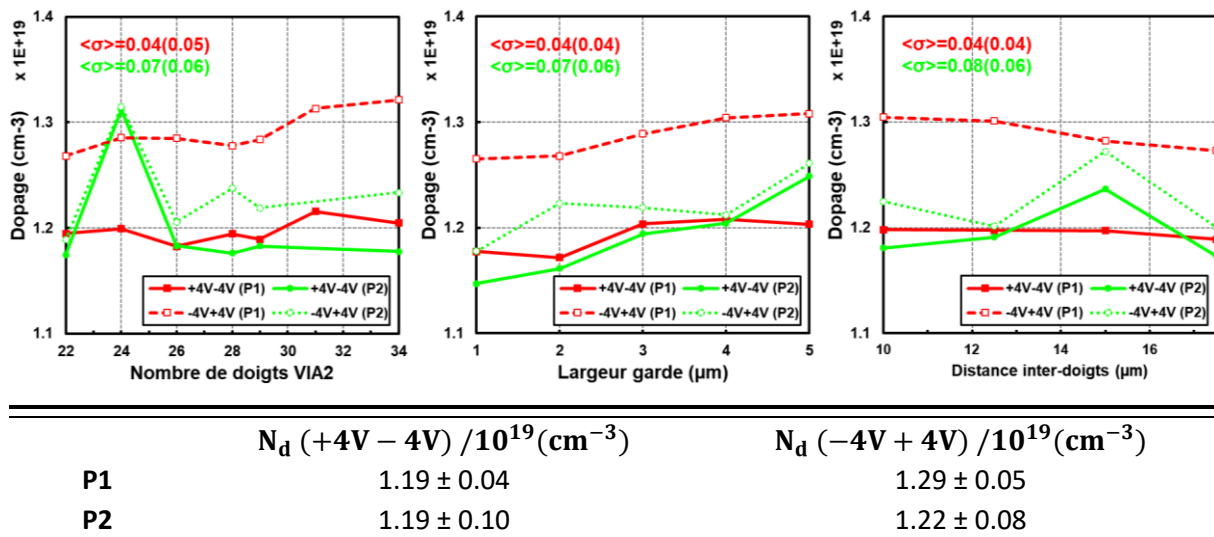
Figure 4-15 : moyenne du dopage effectif N_d en fonction des différents paramètres des peignes interdigités ; le tableau donne la moyenne du dopage sur l'ensemble des mesures C-V fonctionnelles des plaques P1 et P2.
