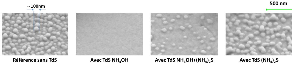
Figure 3-15 : clichés MEB après un dépôt ALD-Al 2 O 3 d'environ 28nm sur des surfaces InGaN (50 cycles H 2 O/TMA, puis 250 cycles PEALD TMA/plasma O 2 , à 250°C), pendant la fabrication de condensateurs MIS, et plus précisément, juste après une étape de gravure ICP au cours de laquelle l'InGaN est surgravé.
