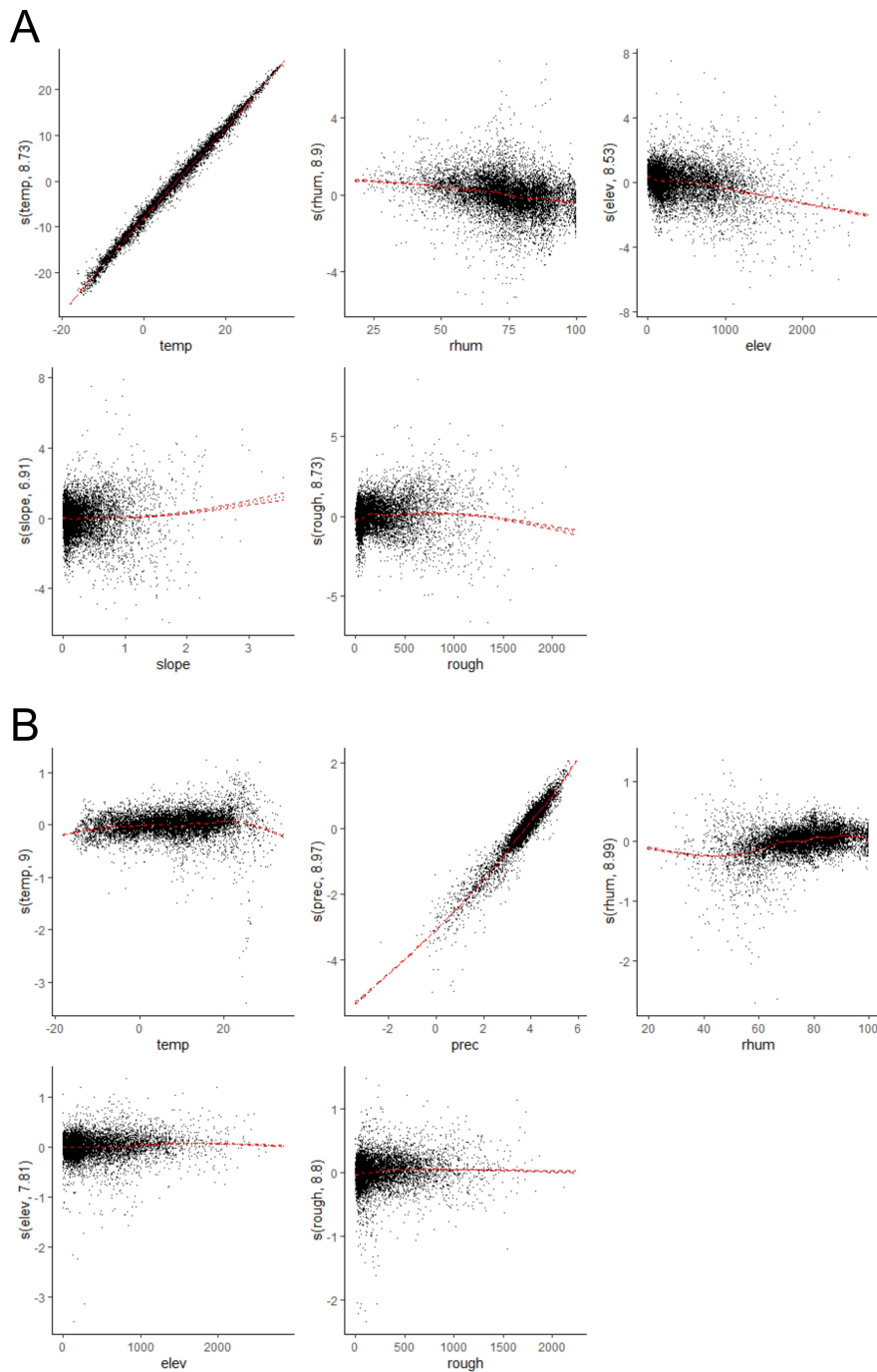
Figure II.1.5: Courbes de régression des modèles GAM sélectionnés pour la température (A) et la précipitation (B) issues des simulations à l'équilibre.
