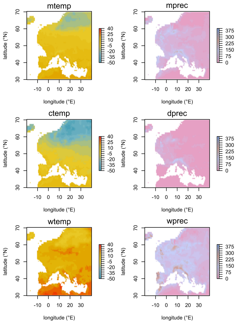
Figure II.1.1: Les six climatologies retenues pour modéliser le climat dans ce travail. Exemple du modèle HadCM3 à l'équilibre à 30 ka BP.
