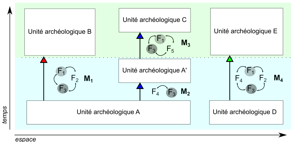
Figure I.1.9: Illustration du concept de mécanismes pour un exemple fictif. Le schéma présente trois trajectoires culturelles régionales ( flèches de couleur ) au sein d'un contexte environnemental marqué par une période froide ( fond bleu ciel ) et une période plus douce ( fond vert clair ). Chaque évolution au sein d'une trajectoire est impulsée par un mécanisme ( M ), composé de différents facteurs ( F ) en interaction ( flèches courbes ). Les facteurs grisés représentent des facteurs fréquemment en jeu dans les changements culturels observés.
