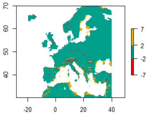
Figure II.1.9: Comparaison de deux méthodes de descente d'échelle avec les données à haute résolution du CRU. Exemple de la température du mois le plus chaud issues des simulations transitoires moyennées sur 30 ans. A. Température du mois le plus chaud à une résolution de 0.16° selon interpolation bilinéaire ou modélisation GAM et température du mois le plus chaud du CRU. B. Différence entre les données CRU et l'interpolation bilinéaire du GCM. C. Différence entre les données CRU et le modèle GAM.
