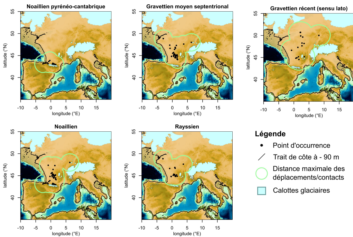
Figure III.1.2: Définition de l'aire de calibration M pour chaque unité archéologique étudiée, à partir des traits de côte à -90 m (Siddall et al., 2003), de l'extension maximale des calottes glaciaires au LGM (Ehlers et Gibbard, 2004) et de la distance maximale d'approvisionnement en matières premières siliceuses (cf. Tableau III.1.2).
