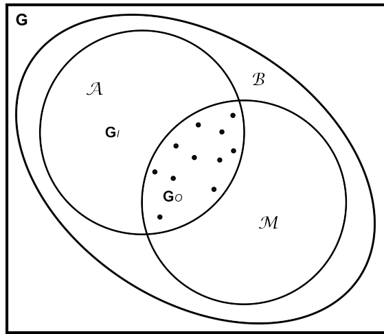
Figure I.2.4: Diagramme de BAM illustrant les facteurs influençant la distribution macro-géographique d'une espèce dans le cas de l'hypothèse du bruit Eltonien (d'après Soberón et Peterson, 2005, 2012, modifié). Les cercles représentent les différents facteurs et les points noirs représentent la distribution géographique de l'espèce. G : espace géographique ; A : variables scénopoétiques ; B : interactions biotiques ; M : zones géographiques accessibles à l'espèce ; G_O : aire de distribution occupée ; G_I : aire de distribution potentiellement envahissable.
