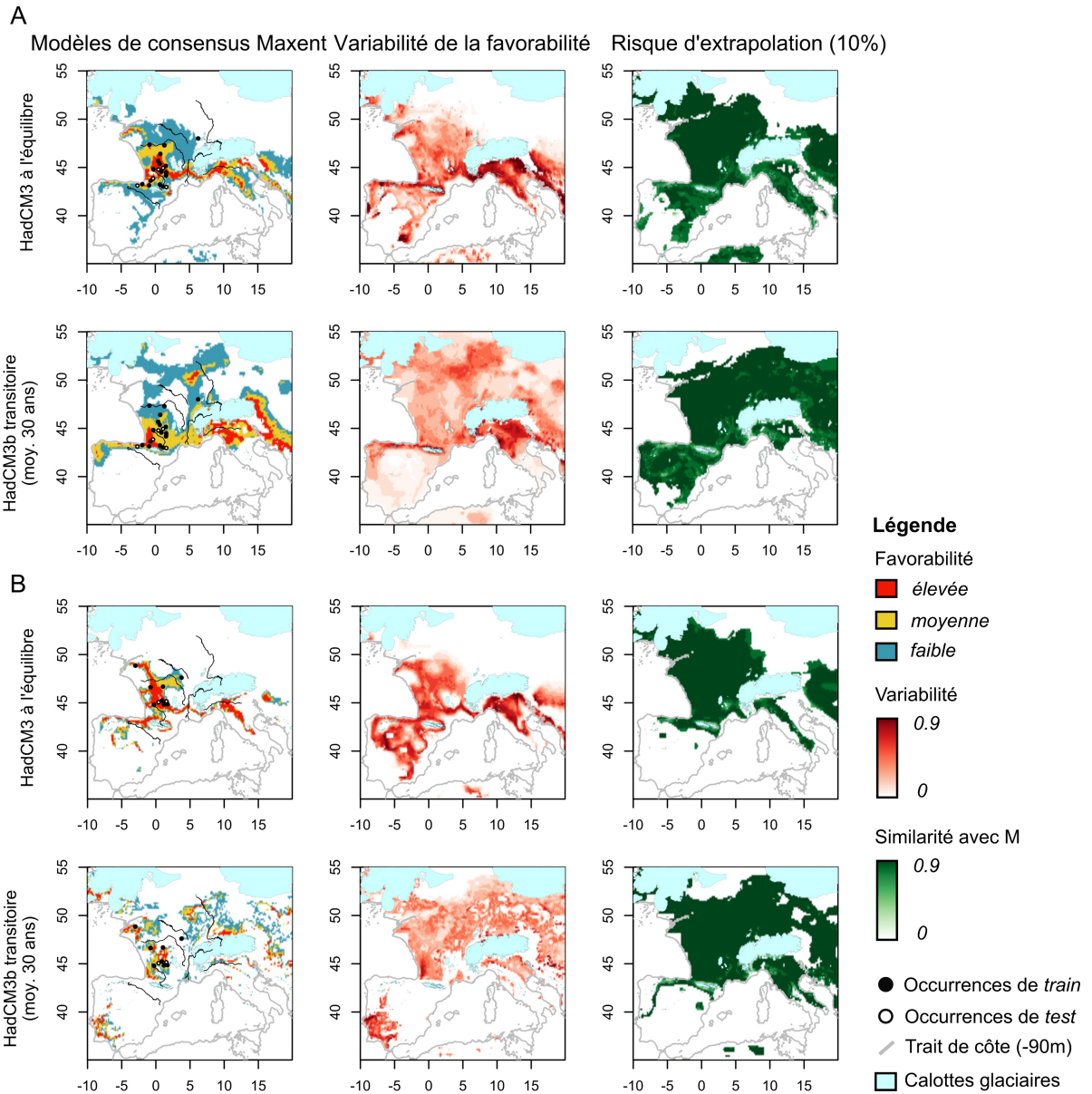
Figure III.2.11: Modèles de consensus de niches Maxent pour les unités archéologiques du scénario 2 à 30 ka. A. Noaillien. B. Rayssien.
