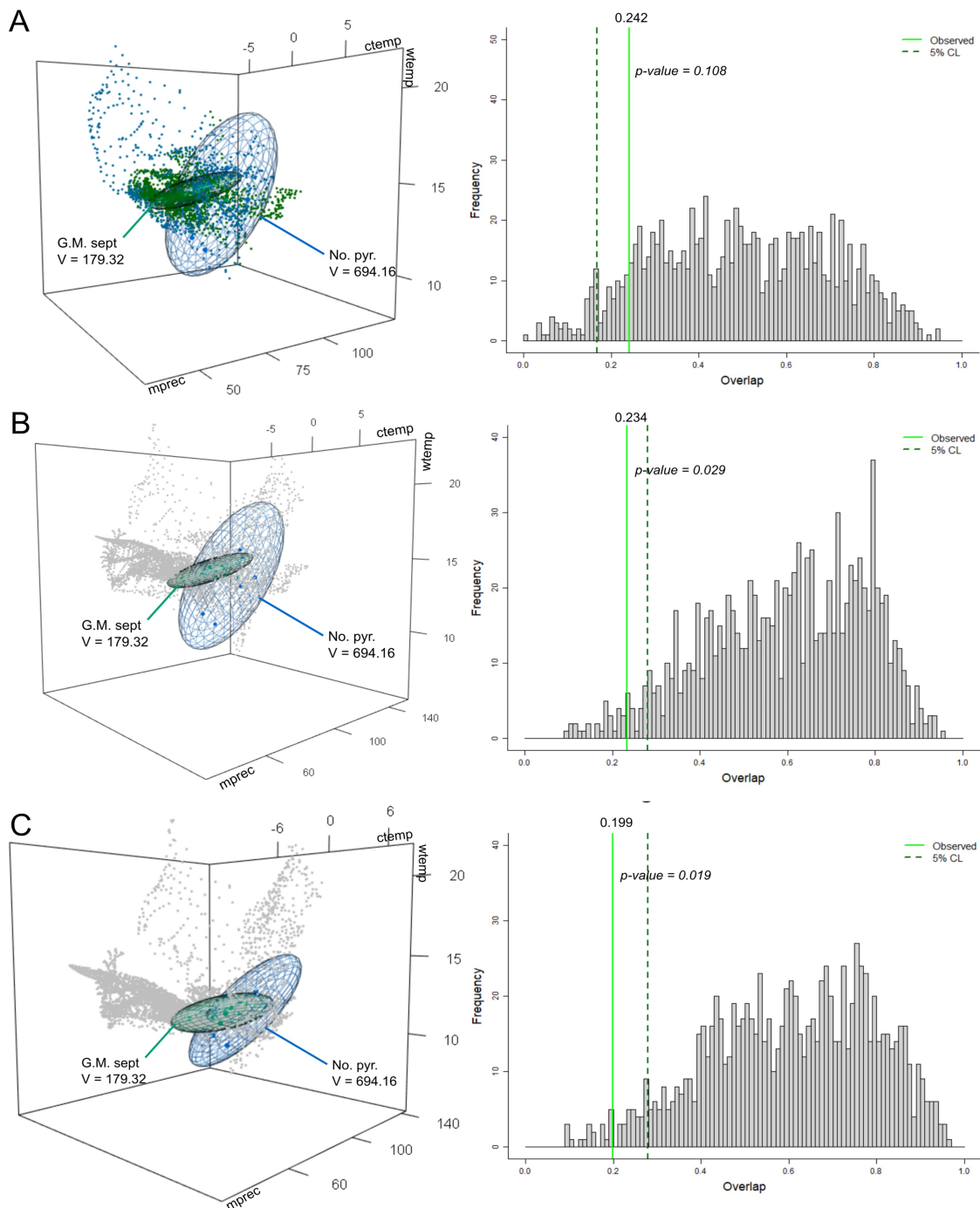
Figure III.2.7 : Recherche des facteurs de variabilité entre les modèles d'ellipsoïdes issus de l'article et ceux présentés dans cette thèse. Exemple des modèles issus des simulations à l'équilibre. A. Cas n°1 : utilisation des variables ctemp , wtemp , mprec à 30 ka. B. Cas n°2 : utilisation des variables ctemp , wtemp et mprec avec l'aire de calibration de l'article à 30 ka. C. Cas n°3 : utilisation des variables ctemp , wtemp et mprec avec l'aire de calibration de l'article à 32 ka.
