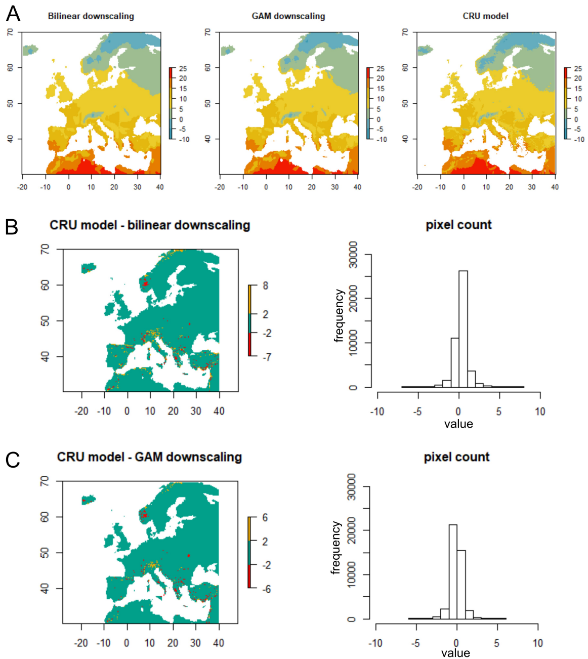
Figure II.1.6: Comparaison de deux méthodes de descente d'échelle avec les données à haute résolution du CRU. Exemple de la température moyenne annuelle issues des simulations à l'équilibre. A. Température moyenne annuelle à une résolution de 0.16° selon interpolation bilinéaire ou modélisation GAM et température moyenne annuelle du CRU. B. Différence entre les données CRU et l'interpolation bilinéaire du GCM. C. Différence entre les données CRU et le modèle GAM.
