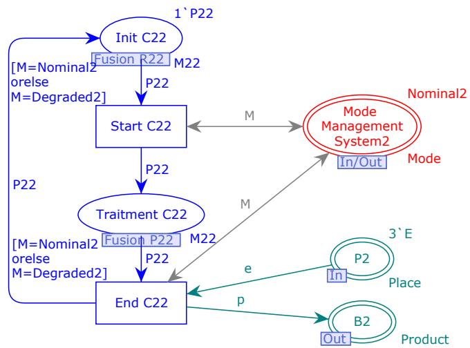
(e) Sous-page C22
