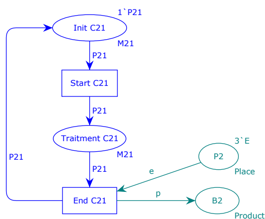
Figure 4.7 – Modèle de C21
