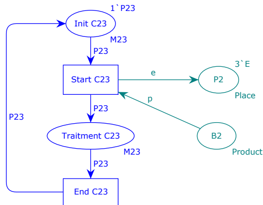
Figure 4.9 – Modèle de C23
