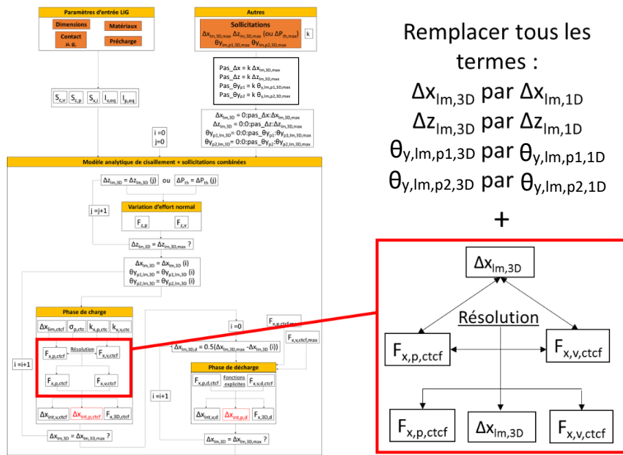
Figure 4-26 : Intégration de la correction de type Morping dans la méthode de résolution des modèles analytiques de CTCF et CTCF,TH.
