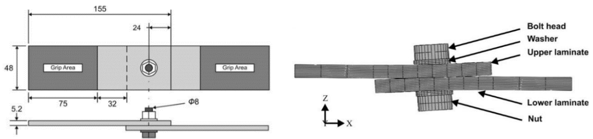
Figure 1-33 : Modélisation numérique d'une liaison sollicitée en cisaillement. Specimen (gauche) et modèle numérique (droite) [GRA, 2010].
