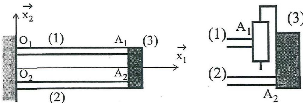
Figure 1-27 : Modèle analytique de bilame soumis à une variation de température \Delta T [BOU, 1989].
