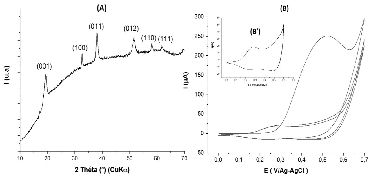
Figure 81 : A) Diffractogramme X de \beta\text{-Co(OH)}_2 , B) Courbes de voltammétrie cyclique de \beta\text{-Co(OH)}_2/\text{PGE} (20 \mu\text{g} ) (3 premiers cycles) dans NaOH 0,1 M, \nu = 10 \text{ mV s}^{-1} , B') 3 ème cycle entre 0-0,6 V/Ag-AgCl.
