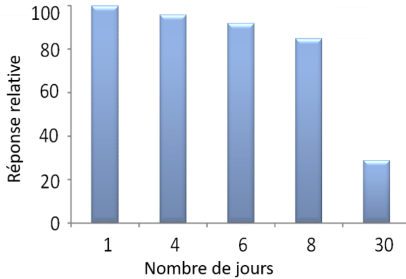
Figure 103 : Réponse relative des biocapteurs \text{Co}_3\text{Mn}/\text{GOx}/\text{Carragénane} en fonction du temps de stockage à 6 °C.
