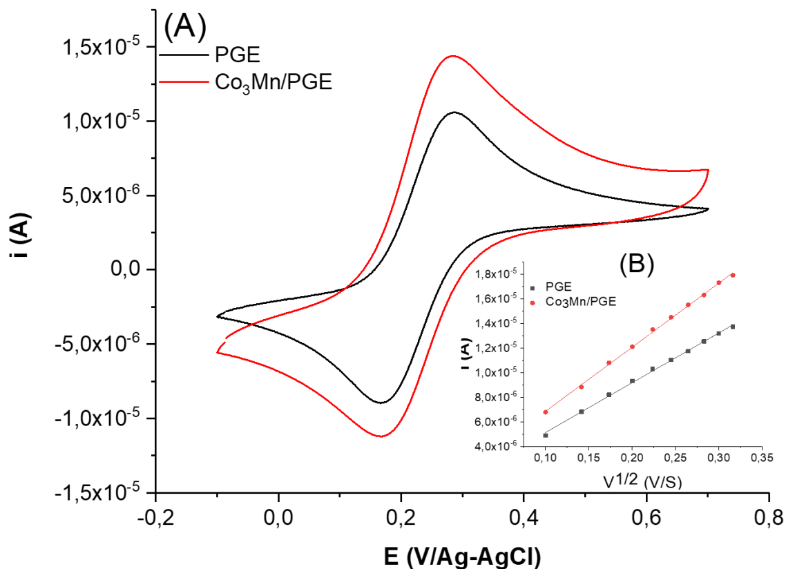
Figure 79 : Courbes de voltammétrie cyclique de 1 mM K_4FeCN_6 dans 0,1 M KCl sur PGE nue et électrode modifiée Co_3Mn/PGE ( \nu = 50 \text{ mV.s}^{-1} ) (A). La variation de I_{p_a} en fonction de \nu^{1/2} pour les deux électrodes (B).
