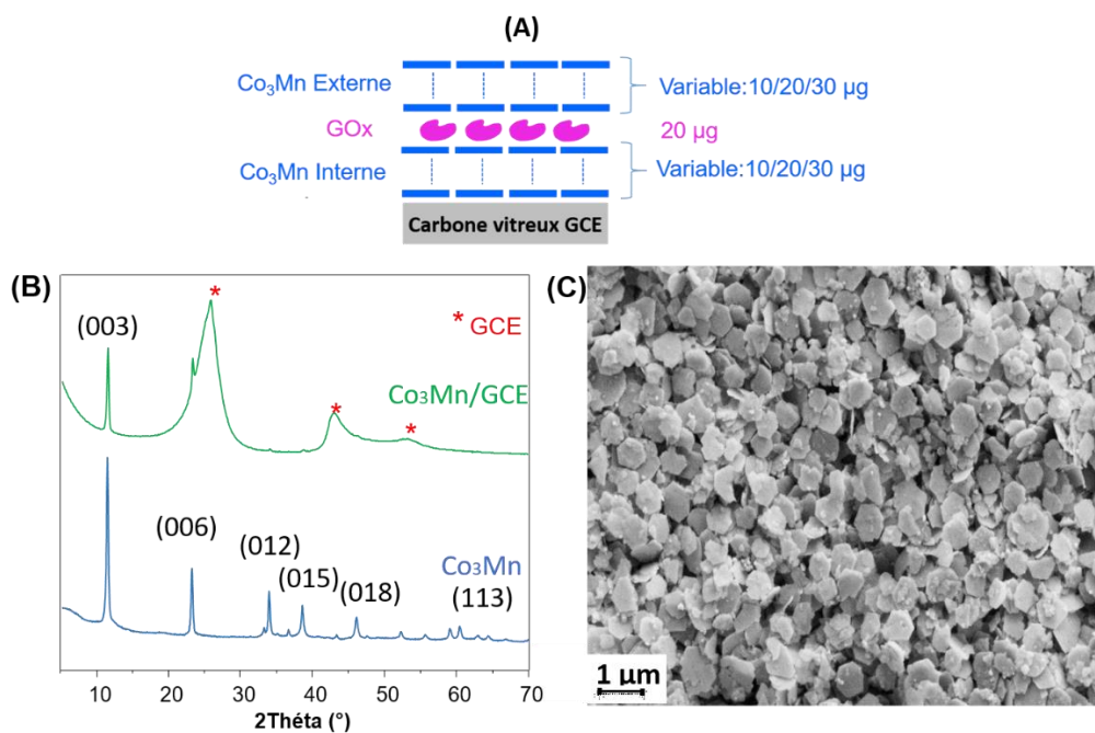
Figure 100 : (A) Configuration multicouche des biocapteurs Co_3Mn/GOx/Co_3Mn , (B) Diffractogramme X de Co_3Mn et Co_3Mn/GCE et (C) Images MEB de Co_3Mn/GCE .
