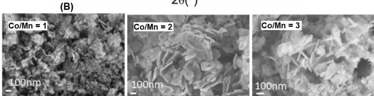
Figure 29 : Diffractogrammes X (A) et image MEB (B) des phases HDL \text{Co}_R\text{Mn} ( R=1, 2, 3 ) d'après [89].
