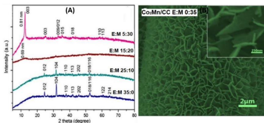
Figure 38 : Diffractogramme X de CoMn-HDL/CC coprécipités dans différents mélanges eau/méthanol (E:M) (A) et cliché MEB de Co 2 Mn/CC (B) d'après [100].
