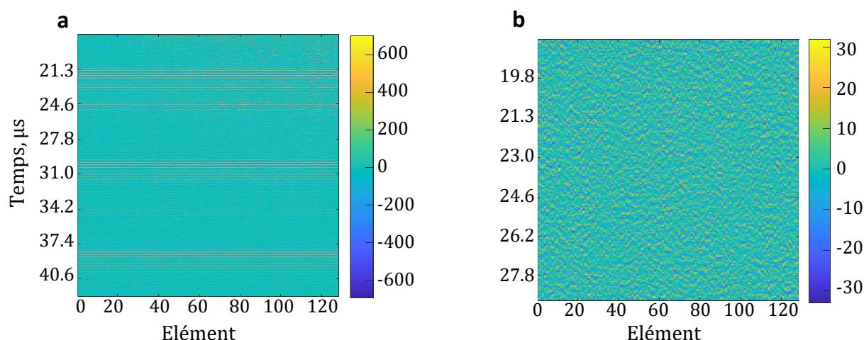
Figure 2.3 – Bruit de mesure sur les signaux radiofréquences expérimentaux.
