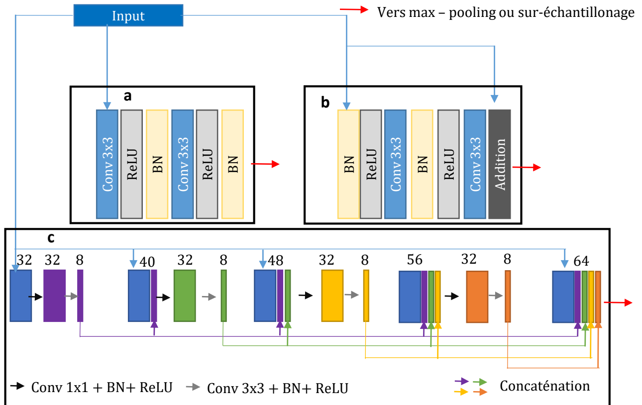
Figure 5.22 – Les différents types de blocs utilisés pour construire les réseaux de neurone. BN pour batch normalization, conv pour convolution. (a) : bloc U-Net. (b) : bloc Resunet, la donnée d'entrée du bloc est ajoutée à la sortie du bloc. (c) : bloc FD U-Net pour un taux d'agrandissement de 4 et une donnée d'entrée à 32 canaux. Les chiffres indiqués représentent le nombre de canaux après chaque opération.
