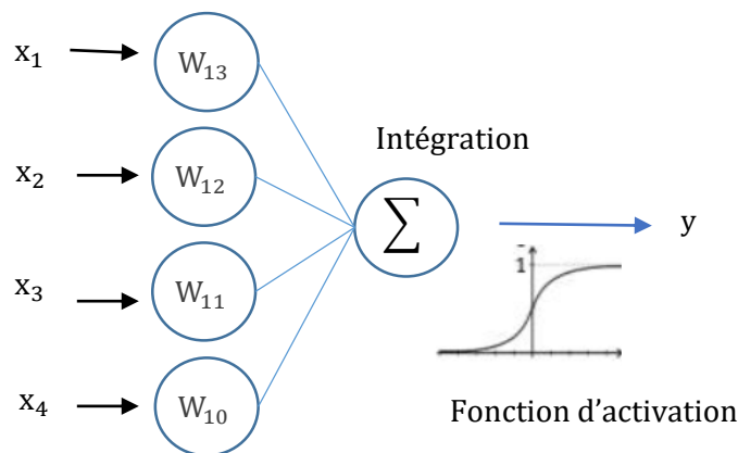
Figure 5.3 – Représentation d'un neurone artificiel, modèle du perceptron.
