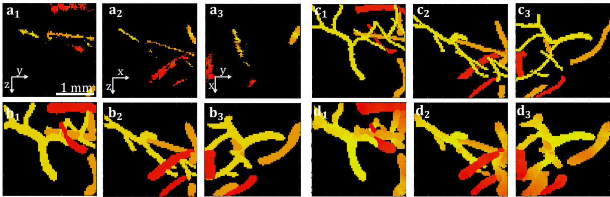
Figure 6.5 – Estimation de la saturation en oxygène ( SO_2 ) des pixels appartenant aux projections d'intensité maximale de :
