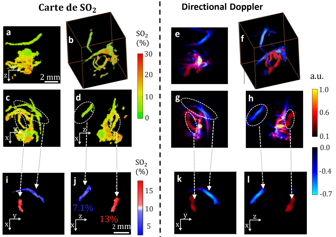
Figure 4.12 – SO_2 et analyse de flux conjointe.
