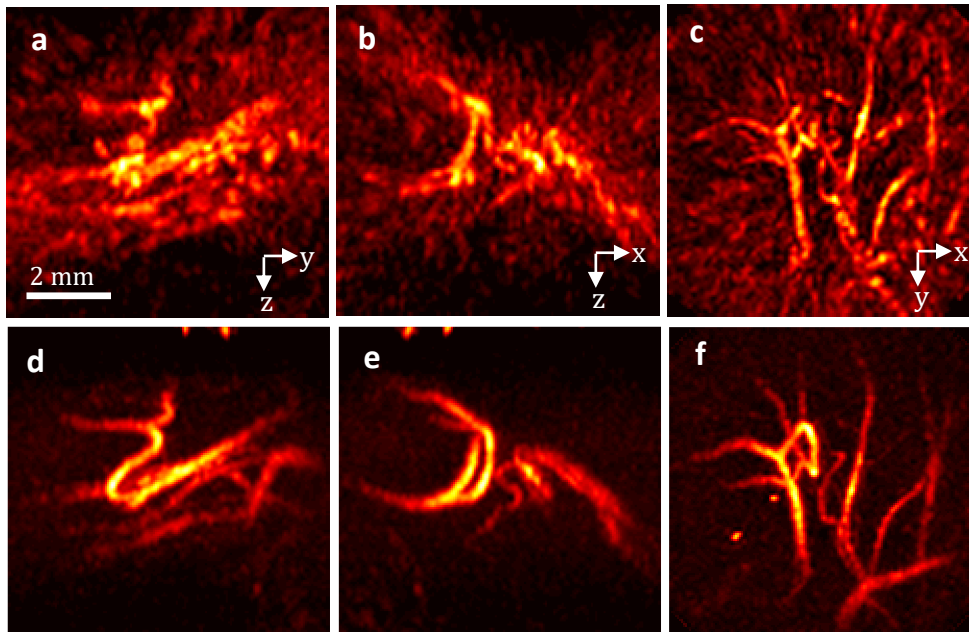
Figure 3.10 – Intensités maximales projetées dans les plans YZ (a,d) XZ (b,e) et XY (c,f) de l'image moyenne (première ligne) et de l'image de fluctuation (seconde ligne) d'un embryon de poulet.
