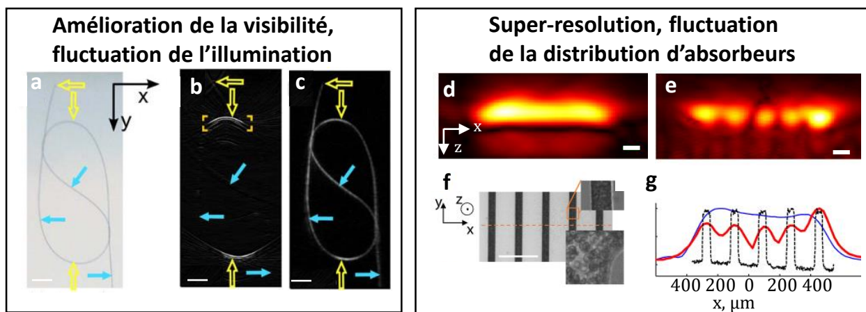
Figure 3.1 – (a-c) : imagerie photoacoustique (PA) de fluctuation pour la correction des artefacts de visibilité par fluctuation de l'illumination [40]. Une série d'images PA 2D d'un phantom (photographie en a) est obtenue. Entre chaque image, le motif de speckle subdiffraction acoustique composant l'illumination change de manière aléatoire. En (b), la moyenne de 50 images : les artefacts de visibilité (flèches bleues) sont présents. En (c), image de fluctuation : les artefacts sont corrigés.
