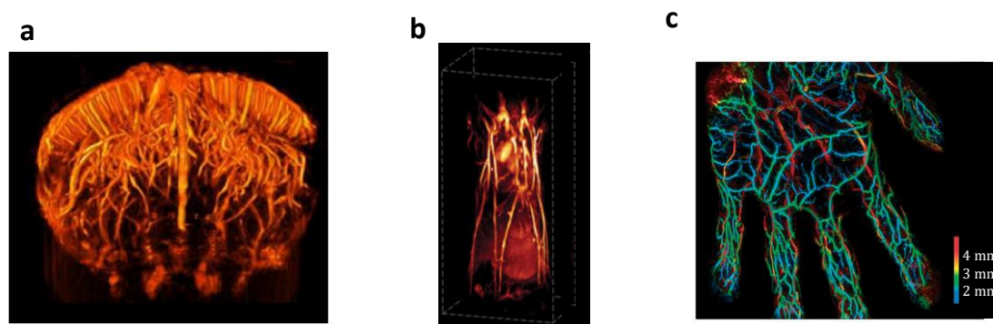
Figure 1.16 – (a) : Image Doppler ultra-rapide d'un cerveau de souris [29]. (b) : Image photoacoustique corps entier d'une souris [27]. (c) : Projection de l'intensité maximale dans le plan XY de l'image photoacoustique 3D d'une main humaine, la couleur encode la profondeur [86].
