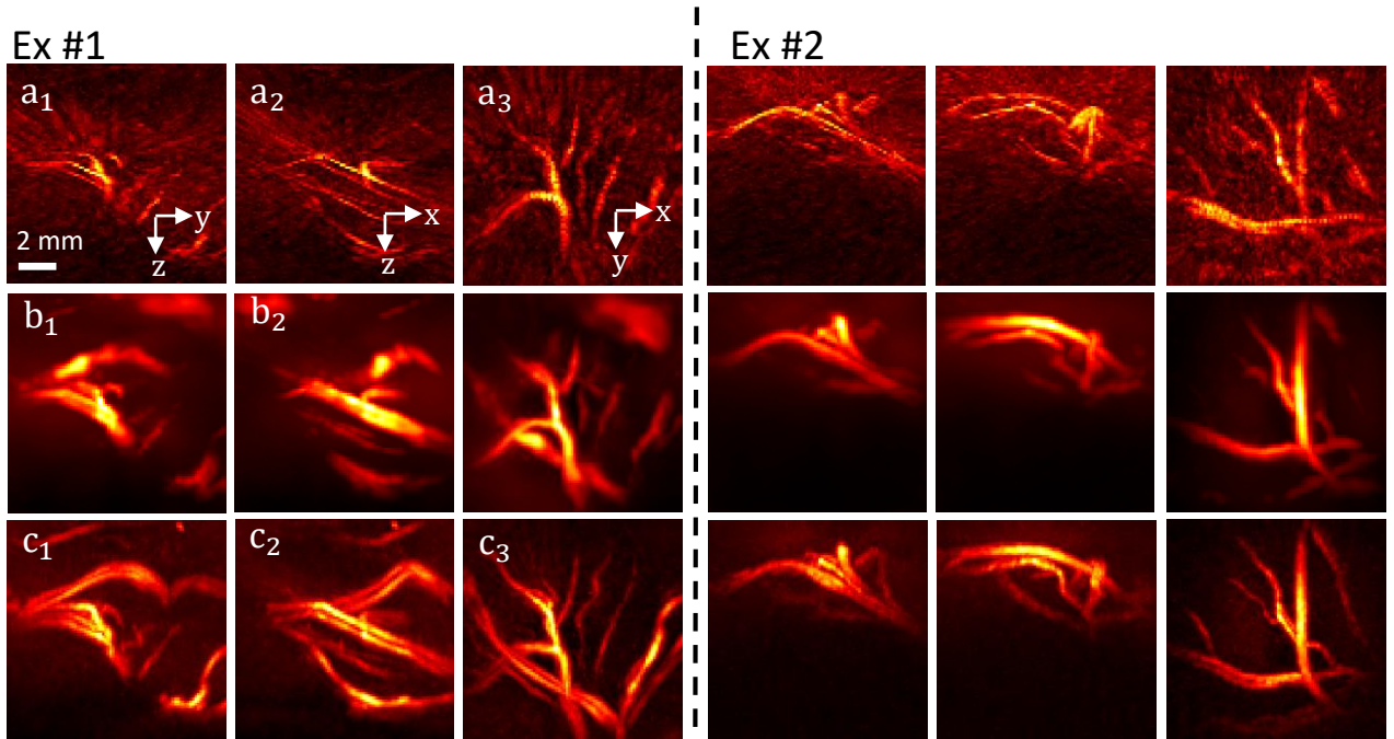
Figure 6.10 – Résultats expérimentaux de l'approche réseau de neurones avec l'image de fluctuation 3D comme ground truth. Deux exemples du test set sont présentés. La première ligne correspond à l'image conventionnelle, la seconde à l'image prédite par le réseau, et la troisième à l'image de fluctuation. Les indices 1, 2 et 3 correspondent respectivement à l'intensité maximale projetée dans le plan YZ, XZ et XY.
