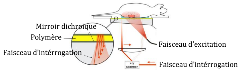
Figure 1.20 – L'épaisseur du capteur, un film fin en polymère, varie lors du passage de l'onde photoacoustique générée par le faisceau d'excitation. Ces variations sont mesurées en focalisant un faisceau d'interrogation en un point du capteur et en enregistrant la modulation de l'intensité du faisceau réfléchi. En balayant point par point le faisceau focalisé sur la surface du capteur, on synthétise un capteur multiélément. Modifié de [50].
