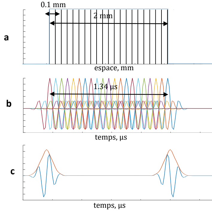
Figure 3.4 – Convolution 1D entre un objet de taille 2 mm et une point spread function (PSF) de longueur caractéristique 0.185 μm. (a) : représentation de l'objet en bleu, position des particules en noir. (b) : les signaux générés par chaque particule sont représentés en différentes couleurs. (c) : somme de ces signaux, correspondant à l'opération de convolution entre la PSF et l'objet, en bleu avec la PSF réelle et en orange avec la PSF complexe, le module du résultat de l'opération de convolution est dans ce deuxième cas représenté.
