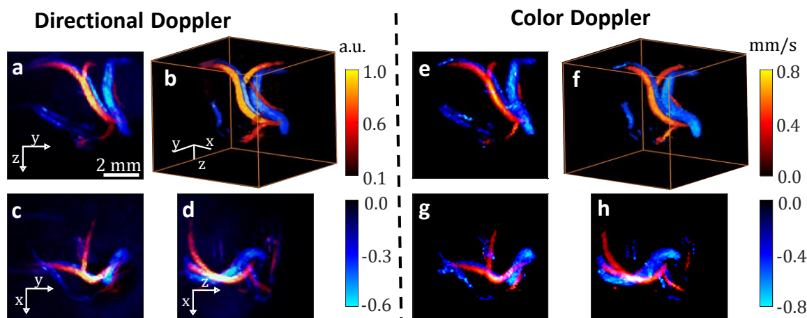
Figure 4.10 – Analyses de flux.
