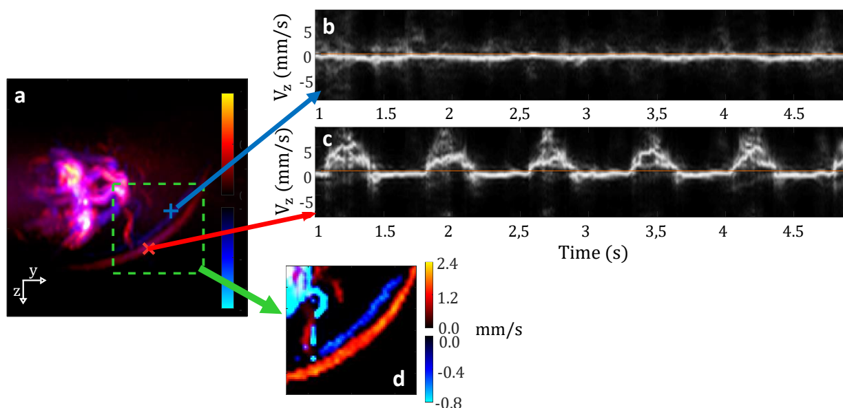
Figure 4.11 – Analyse de flux, pulsatilité.
