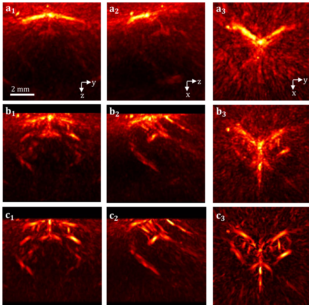
Figure 3.15 – Intensités maximales projetées dans les plans YZ, XZ et XY (indices 1, 2 et 3) pour (a) l'image moyenne, (b) l'image de fluctuation et (c) l'image de fluctuation après application d'un filtre de Frangi.
