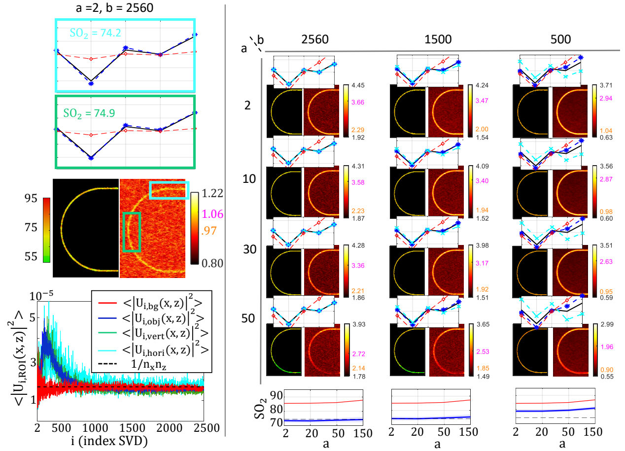
Figure D.1 – Étude de l'impact des bornes a et b sur un objet de type boucle. Cas avec bruit et variation de la fluence selon \Phi_{k,\lambda} . Les courbes représentent les coefficients d'absorption théorique en noir, et ceux estimés à partir des images de fluctuation sans correction du bruit (rouge), sans correction de l'effet de la décomposition en valeurs singulières sur l'estimation du bruit (cyan) et en corrigeant cet effet (bleu). Les nombres en magenta et orange sur la barre de couleur des images de fluctuation correspondent respectivement à la valeur moyenne des pixels au centre de l'objet et dans une zone de bruit.
