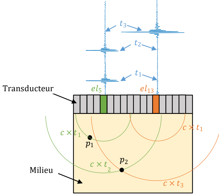
Figure 1.8 – Représentation sphérique du beamforming en imagerie photoacoustique dans le cas de l'imagerie 2D. Un milieu composé de deux absorbants est imagé, et les signaux de deux des transducteurs constituant la sonde d'imagerie (en vert, el_5 et en orange, el_{13} ) sont présentés. La particule p_1 est située sur le cercle de rayon c \times t_1 ayant pour centre el_5 , un signal est donc enregistré par el_5 au temps t_1 . Aucune particule n'est située sur le cercle de même rayon de centre el_{13} , aucun signal n'est donc enregistré à ce même temps t_1 . Même situation pour t_2 avec la seconde particule. A t_3 , les deux particules sont situées sur le cercle de rayon c \times t_3 de centre el_{13} : un signal de plus grande amplitude, correspondant à la somme des contributions de chacune de des particules, est visible.
