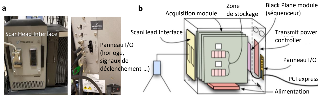
Figure 2.2 – Photographies de l'échographe "High Frequency Vantage 256 system, Verasonics" en (a) et schéma correspondant en (b). Sur la photographie de la Scan Head Interface, l'un des deux connecteurs est relié à une sonde d'imagerie.
