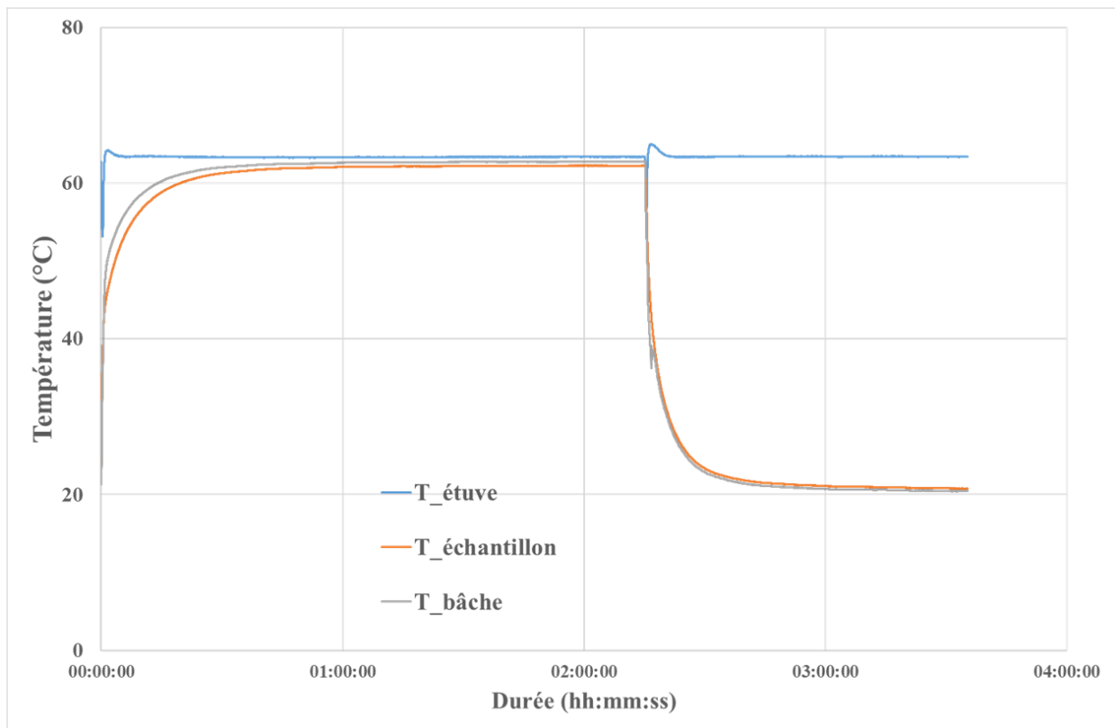
Figure 3.5 : Profils de température enregistrés au niveau de l'étuve, de la bache et d'un échantillon lors d'un cycle d'imprégnation sous vide et en étuve.
