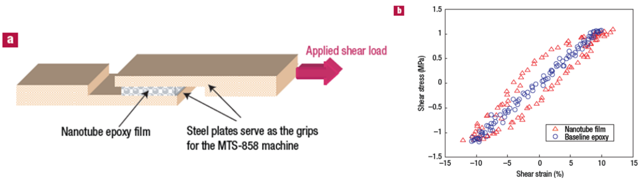
Figure 1.41 : (a) Schéma de principe d'un essai de vibration par cisaillement ; (b) Profils contrainte – déformation de cisaillement de résines de référence et nano- structurée, avec mise en évidence d'une boucle d'hystérésis caractéristique du cas de la résine nano-structurée [70].
