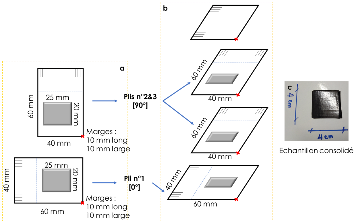
Figure 3.15 : Trois tapis de nanotubes transférés sur des plis de pré-impregné en vue de la consolidation des 4 plis du composite. (a) Plis à 0° et à 90°, avec tapis de VACNTs, (b) Schéma de drapage, (c) Exemple de l'échantillon L consolidé.
