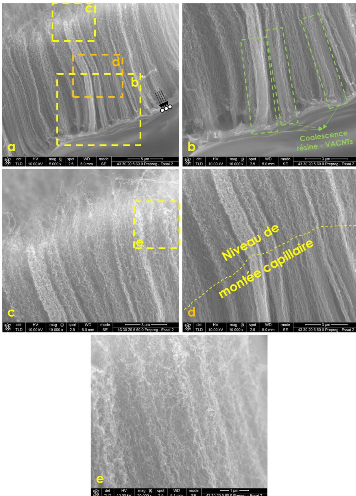
Figure 2.26 : (a) Une forêt de VACNTs partiellement imprégnée par la résine ; (b) Grossissement : certaines zones de coalescence sont visibles aux têtes de VACNTs ; (c) Grossissement : Morphologie tortueuse des pieds de VACNTs secs ; (d) Zone de transition entre la zone imprégnée et la zone sèche, (e) Zone de grossissement de 20 000.
