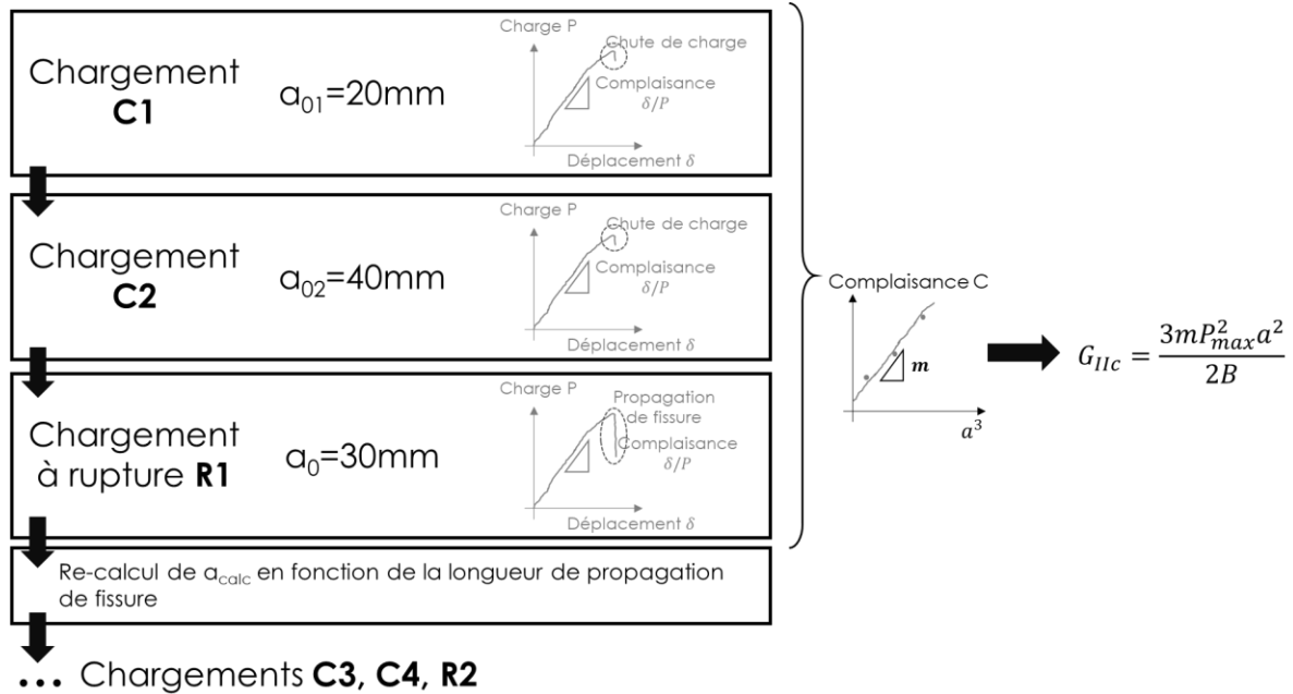
Figure 4.15 : Essais ENF - Description des étapes de chargement mécanique et d'exploitation des données pour déterminer le G_{IIc} .
