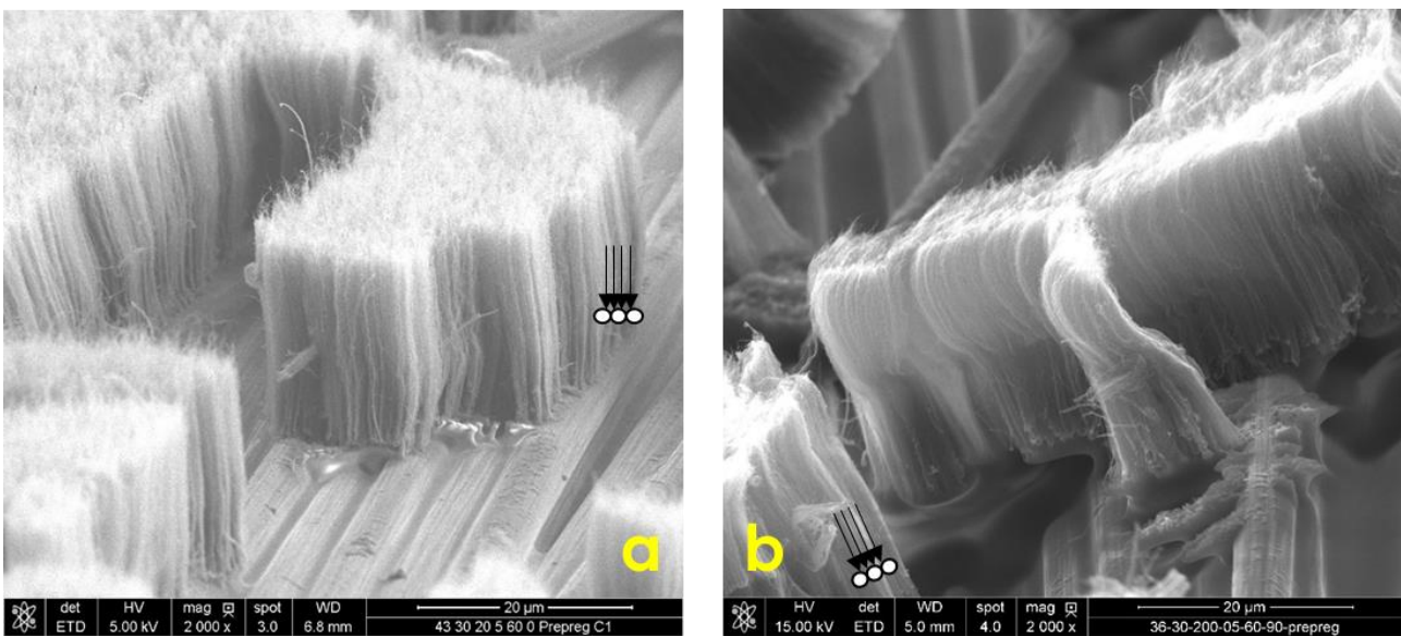
Figure 2.25 : (a) VACNTs verticaux et alignés après transfert à 20kPa de pression (VACNTs-30µm/M55J-M18)/(T60°C/P20kPa/D5mn) ; (b) VACNTs légèrement flambés après transfert à 200kPa de pression (VACNTs-30µm/M55J-M18)/(T60°C/P200kPa/D5mn).
