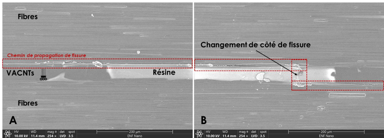
Figure 4.24 : Échantillon ENF nano-structuré – Vue d’une face latérale de l’éprouvette après propagation de fissure et au niveau de la zone nano-renforcée - Observations MEB du chemin de la propagation de fissure.
