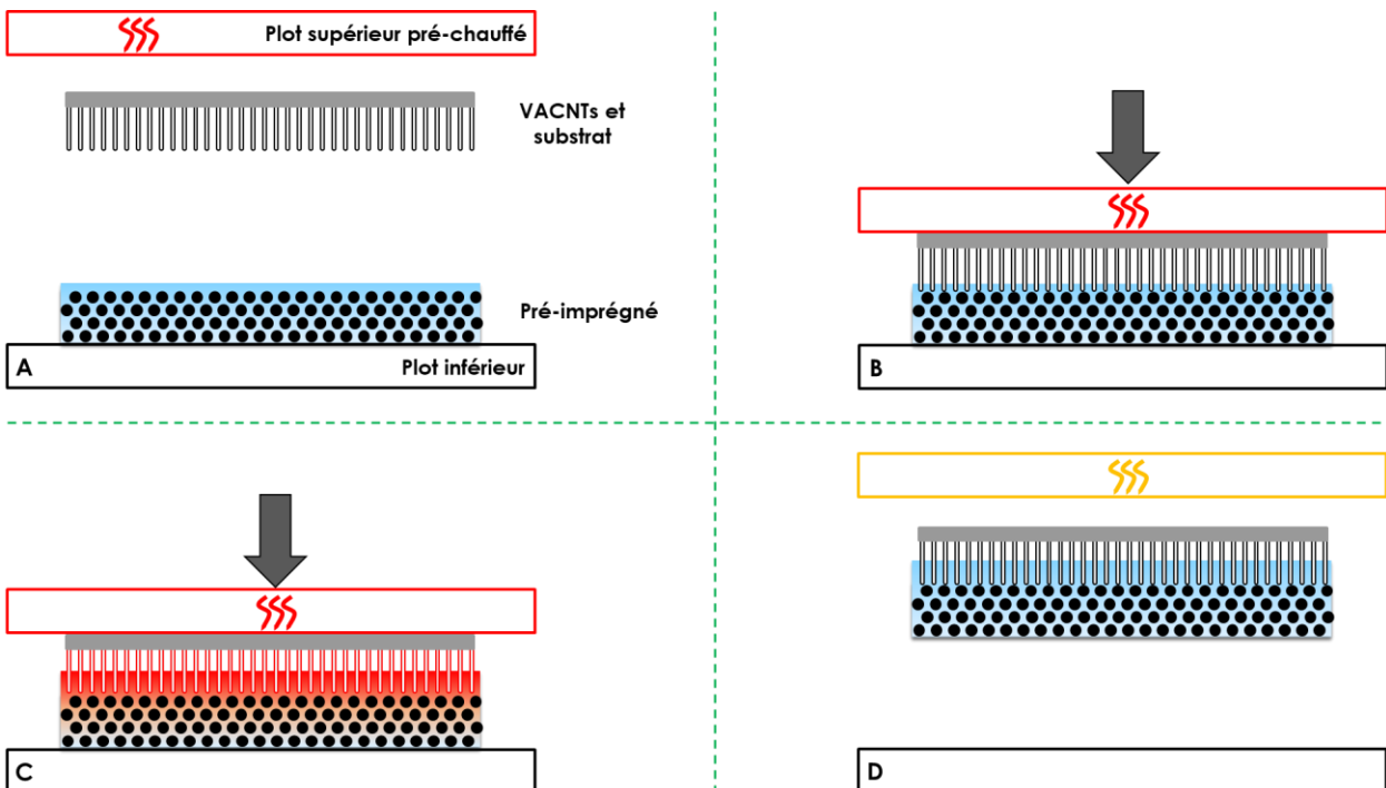
Figure 2.7 : Schéma de principe du procédé d’imprégnation de la résine dans les VACNTs par montée capillaire.
