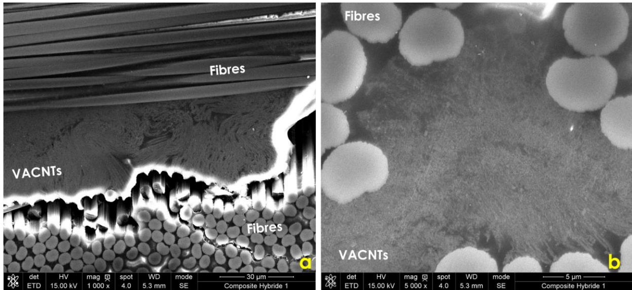
Figure 3.23 : Échantillon K consolidé - Fort flambement de VACNTs entre deux plis de pré-imprégné après consolidation, en autoclave et sous 7bars en continu (images MEB).
