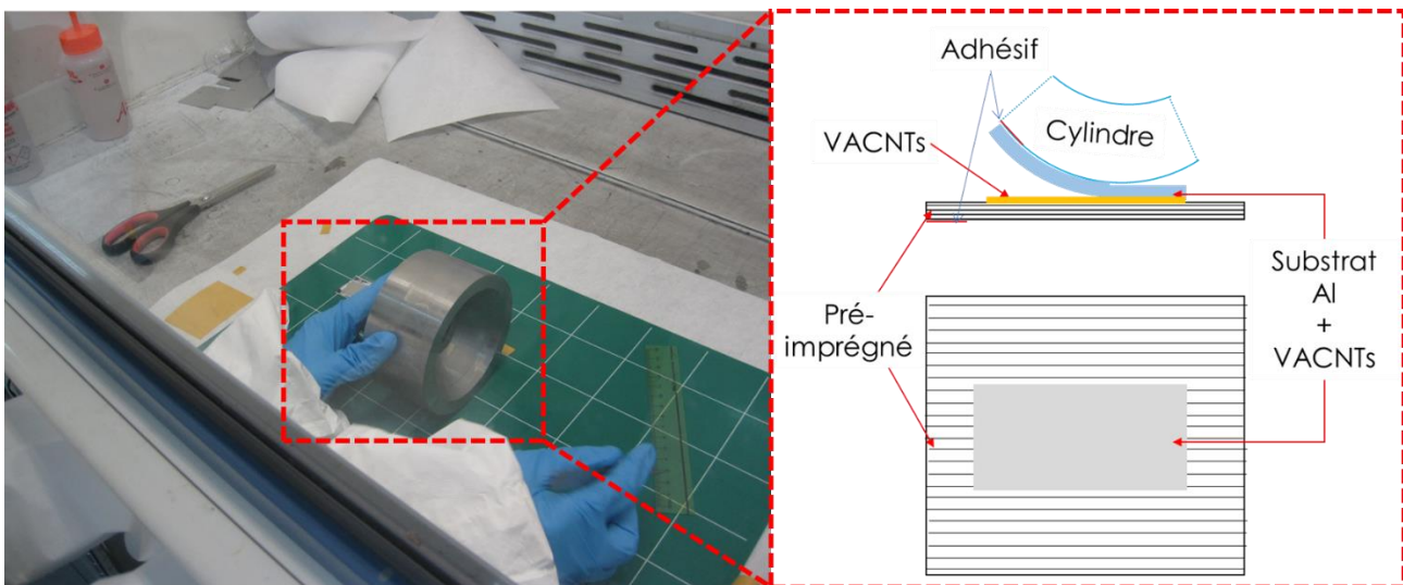
Figure 2.12 : Séparation du substrat de croissance en Al par un cylindre en acier à une température comprise entre 15°C et 20°C.
