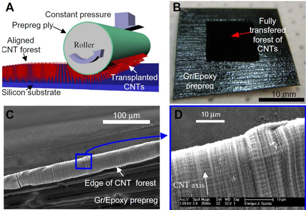
Figure 1.30 : Description et résultat d'un procédé de séparation basé sur l'utilisation d'un cylindre métallique : (A) Illustration du procédé « transfer-printing » ; (B) Forêt de VACNTs transférée à la surface du pré-imprégné ; (C) et (D) Images MEB montrant l'alignement des VACNTs après le transfert [5].
