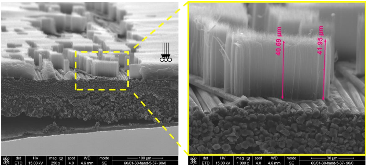
Figure 2.24 : Structure alignée verticale des nanotubes de carbone transférés à la surface du pré-imprégné. (VACNTs-30µm/M55J-M18)/(T37°C/pression-doigt/D5mn).
