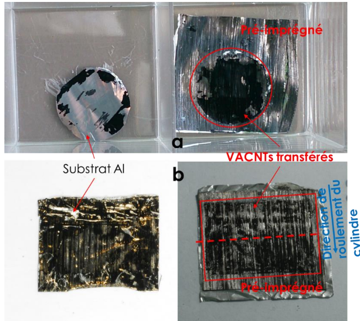
Figure 2.13 : Séparation par cylindre entre 15°C et 20°C. Les zones en noir foncé indiquent la présence des VACNTs. (a) Résultat de transfert pour la configuration plots cylindriques (VACNTs-32 \mu m/NC66-1808NA)/(T50°C/P398kPa/D20mm) ; (b) Résultat de transfert pour la configuration plots rectangulaires (VACNTs-32 \mu m/M55J-M18)/(T60°C/P20kPa/D20mm).
