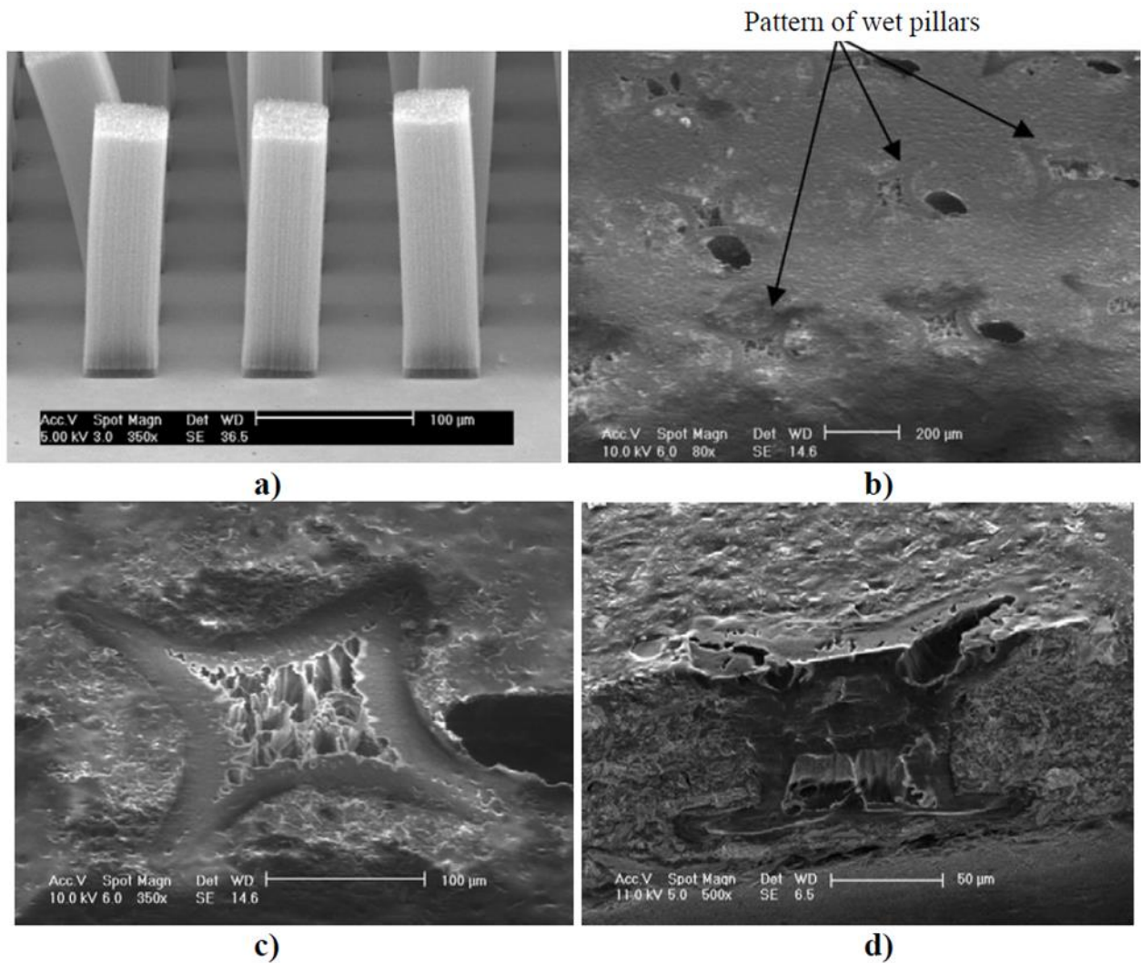
Figure 1.17 : Méthode n°2 - Photos MEB de piliers de VACNTs avant et après transfert: (a) piliers de VACNTs secs de hauteur 100μm et sur leur substrat de croissance ; (b) zone imprégnée et apparition de pores dus à la coalescence locale ; (c-d) Grossissements d'une zone totalement imprégnée par la résine et mise en évidence d'une coalescence locale des VACNTs ainsi que de porosités [49].
