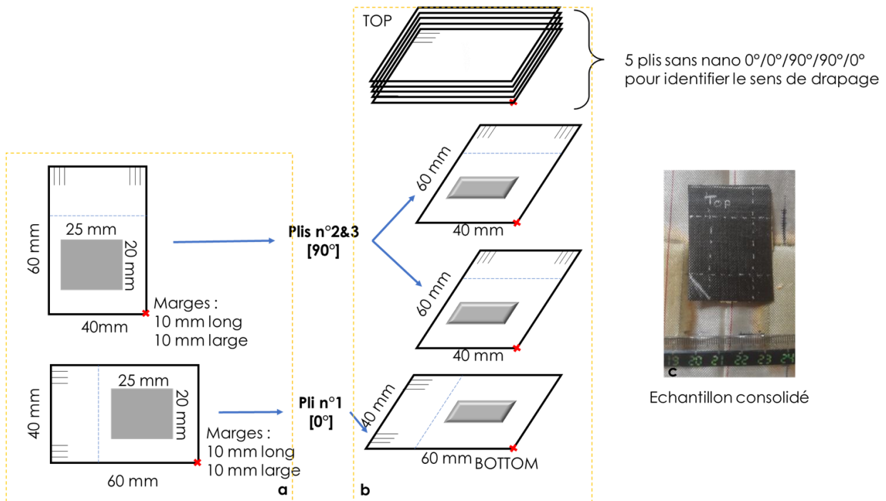
Figure 3.16 : Trois tapis de nanotubes transférés dans les plis de pré-impregné pour la consolidation des 8 plis du composite. (a) Plis à 0° et à 90°, avec tapis de VACNTs, (b) Schéma de drapage, (c) Exemple de l'échantillon M consolidé.
