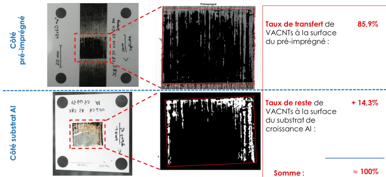
Figure 2.17 : Validation de la méthode de détermination du taux de transfert par analyse d'images : Cas d'un échantillon (VACNTs-J2-33/M55J-M18)/(T60°C/P200kPa/D15mm). La somme du taux de transfert et le taux de reste vaut approximativement 100%.
