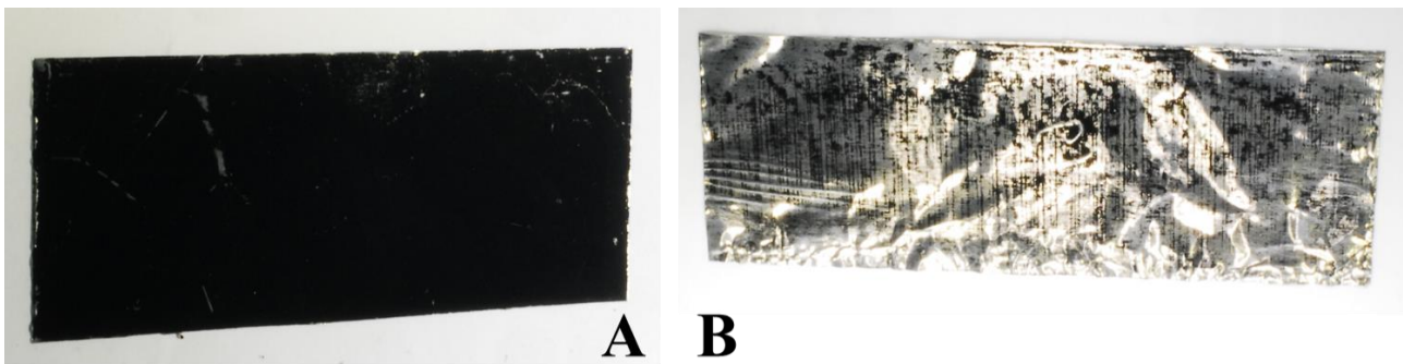
Figure 3.29 : Cas d'un substrat pour le transfert d'un échantillon de compression (Comp-pli19) - (A) Tapis de VACNTs sur son substrat d'alliage d'aluminium avant imprégnation, de dimensions 35 x 90 mm 2 (B) Substrat du même tapis de VACNTs après le transfert.
