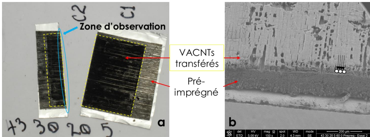
Figure 2.23 : (a) VACNTs transférés à la surface du pré-imprégné – taux de transfert 85% ; (b) MEB en vue de section, certaines fibres ne sont pas couvertes de VACNTs (VACNTs-30µm/M55J-M18)/(T60°C/P20kPa/D5mn).
