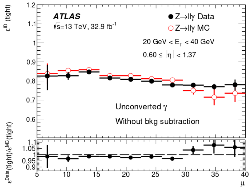
Figure 4.5: Efficacité d'identification des photons non-convertis en fonction du nombre d'interactions des protons par croisement de paquet \mu , dans la région de pseudo-rapacité 0.60 \leq |\eta| \leq 1.37 [107].
