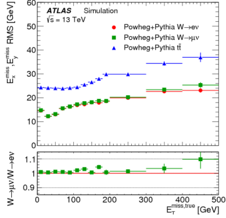
Figure 3.18: Resolution de l'énergie transverse manquante, calculée comme le RMS, en fonction de la vraie énergie transverse manquante pour les événements W \rightarrow e\nu , W \rightarrow \mu\nu et t\bar{t} issus de simulation Monte Carlo. [120]
