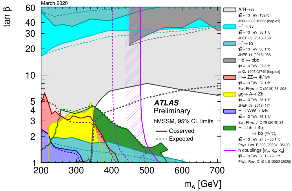
Figure 2.6: Région exclue, en fonction de m_A ( m_h dans notre modèle) et de \tan\beta dans le modèle hMSSM, par des recherches directes de résonance de boson de Higgs lourd et des mesures des taux de désintégration de bosons de Higgs. Les limites à 95% sont indiquées en ligne pleine pour les données et les limites attendues du secteur de Higgs dans le Modèle Standard sont indiquées en ligne pointillées. [58]
