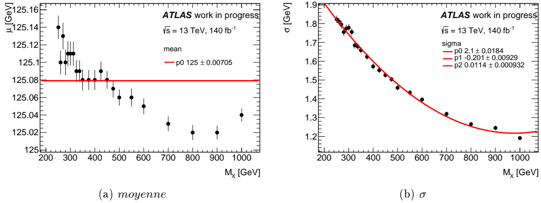
Figure 5.27: Distribution de la moyenne de la fonction DSCB modélisant la masse invariante m_{\gamma\gamma} en fonction de la masse de la résonance (à gauche), l’ajustement (en rouge) est fait avec une fonction constante. Distribution de \sigma de la fonction DSCB en fonction de la masse de la résonance (à droite) l’ajustement (en rouge) est fait avec un polynôme d’ordre 2
