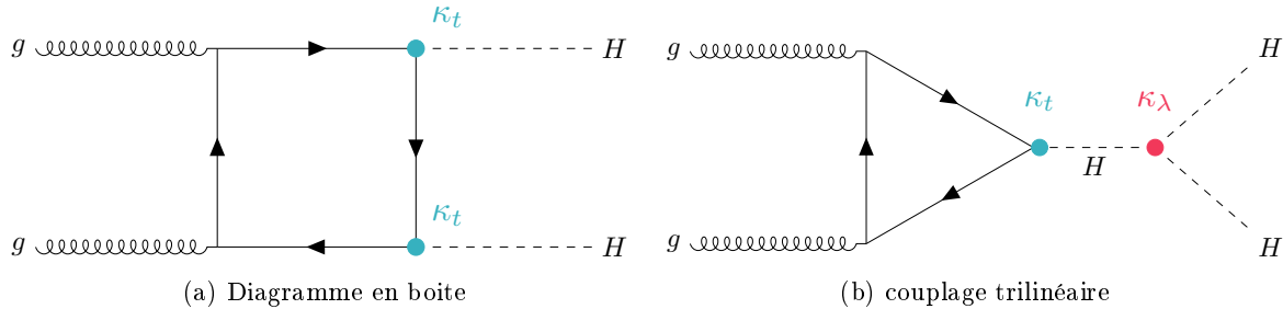
Figure 1.11: Diagrammes de Feynman dominant dans la production issue de la fusion gluon-gluon. Dans le Modèle Standard, la production du couplage trilineaire (à droite) est plus faible que la production que par le diagramme en « boîte » (à gauche). La contribution totale du MS sera la somme des deux en prenant en compte les interférences.
