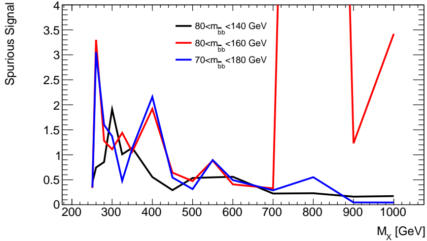
Figure 5.24: Comparaison du signal parasite avec une fonction exponentielle \times exponentielle pour les trois fenêtre de sélections pour la distribution m_{\bar{b}b}
