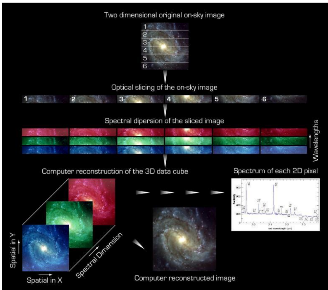
FIGURE 3.1 – Principes de base de la spectroscopie à intégrale de champ. Ici, l'image est découpée en six bandes, dont la lumière est dispersée. Ces bandes sont ensuite recollées pour former un cube de données à trois dimensions. Figure issue du manuel de SINFONI 1 .
