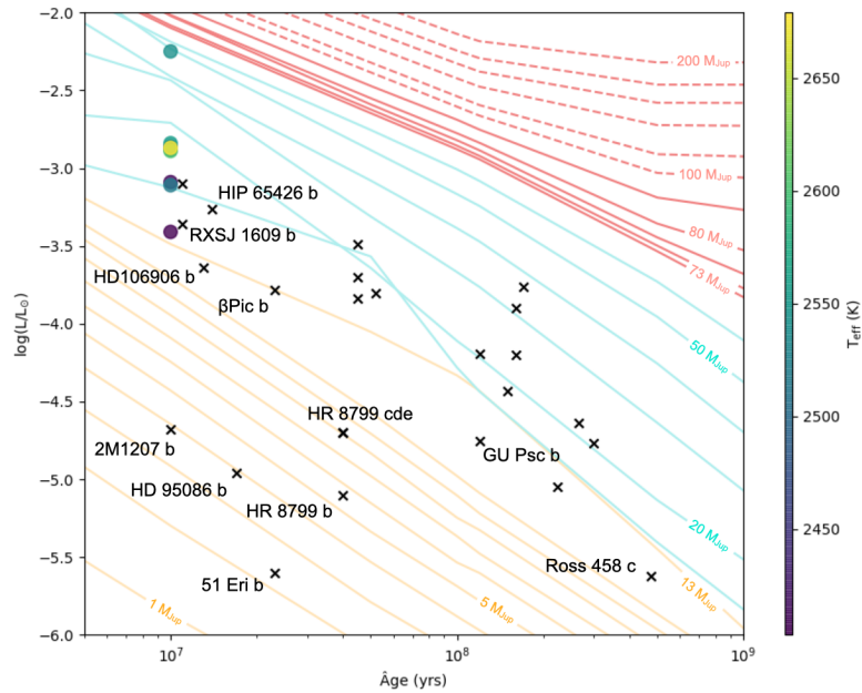
FIGURE 2.10 – Relation luminosité-âge. Les isochrones en masse sont représentées et ont été calculées avec les modèles évolutifs COND03 (Baraffe et al., 2003) pour les traits pleins et de Baraffe et al. (2015) pour les traits en pointillés. Les séparations entre les modèles jaunes-bleus et bleus-rouges marquent les limites de fusion du deuthérium ( M \sim 13 M_{\text{Jup}} ) et de l'hydrogène ( M \sim 73 M_{\text{Jup}} ), respectivement. Les exoplanètes imagées sont représentées par des croix et l'échantillon de naines brunes présenté ici est représenté par des points (leur T_{\text{eff}} est donnée par leur code couleur).
