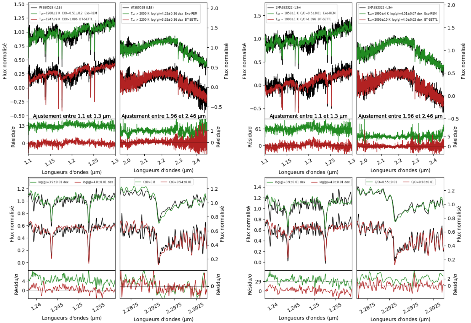
FIGURE 4.21 – Suite de la Figure 4.19. Deux ajustements sont présentés ici, l'un (à gauche), centré sur les absorptions du K I et du Na I (1.1-1.3 μm) et l'autre (à droite), centré sur les absorptions du CO (2.0-2.5 μm).
