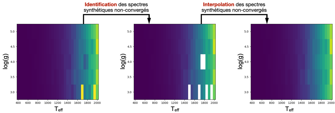
FIGURE 2.7 – Illustration du tri et de l'interpolation des grilles de modèle. La valeur représentée ici est le flux intégré des spectres synthétiques Exo-REM pour des spectres de métallicité [M/H]=0.0 et C/O=0.15 . À gauche : La grille présente des inhomogénéités en flux intégré. Au centre : Les spectres déviants sont identifiés et supprimés de la grille. À droite : Les spectres déviants et les trous dans la grille sont interpolés.
