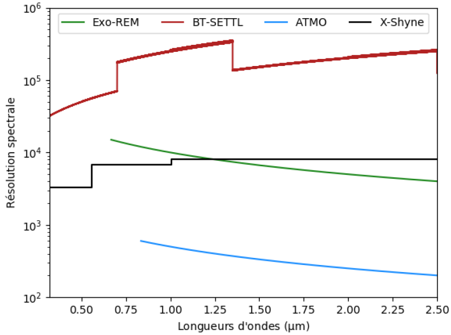
FIGURE 4.15 – Résolution spectrale des différentes grilles de spectres synthétiques en fonction de la longueur d'onde. La résolution des spectres X-Shooter utilisée est représentée en noir.
