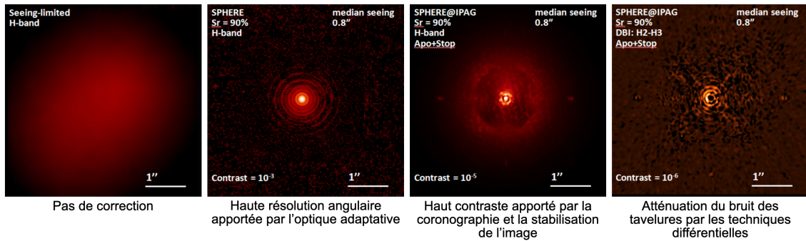
FIGURE 1.3 – Application des techniques de haute résolution angulaire, de haut contraste et de soustraction des résidus stellaires à des données d'imagerie. Figure issue de Chauvin 2018 .
