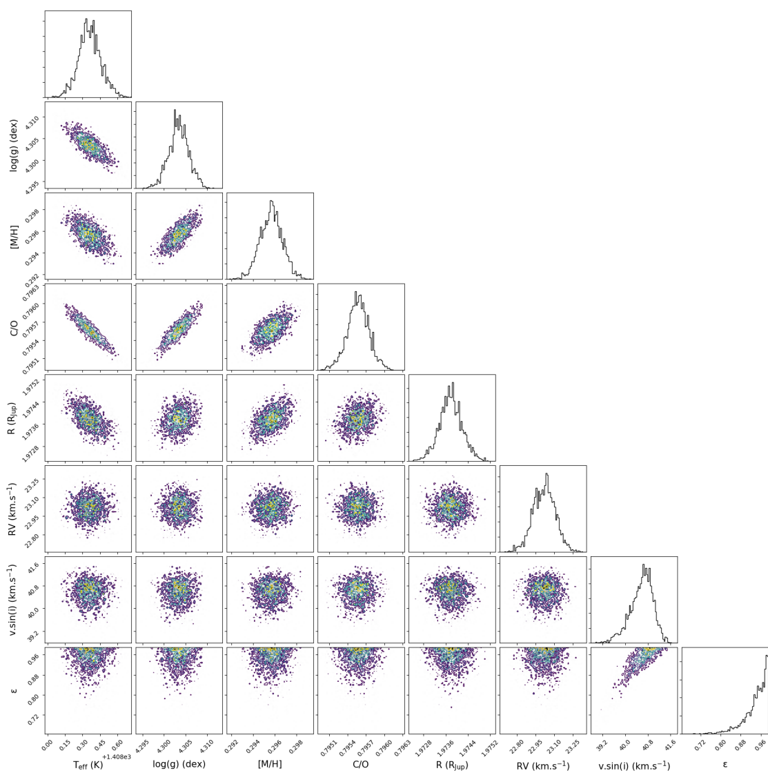
FIGURE 4.17 – Exemple de distributions postérieures pour tous les paramètres obtenus avec les modèles Exo-REM. La source sélectionnée pour cet exemple est 2MASS0723.
