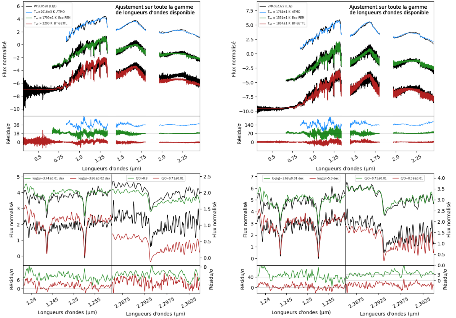
FIGURE 4.19 – Comparaison des ajustements avec les modèles ATMO (bleu), Exo-REM (vert) et BT-SETTL (rouge) sur la L1 \beta WISE0528 (à gauche) et la L3 \gamma 2MASS 2322 (à droite), en utilisant l'ensemble de la couverture spectrale de X-Shooter. Des zooms, centrés sur le doublet du K I ( \sim 1.25 \mu\text{m} ) et sur l'absorption du CO ( \sim 2.3 \mu\text{m} ), sont présentés (en bas) pour montrer la difficulté qu'ont les modèles à reproduire l'ensemble de l'information spectrale.
