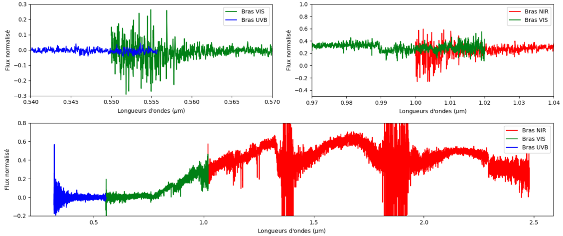
FIGURE 2.6 – Illustration de l'assemblage des spectres des différents bras (en bas) en utilisant le chevauchement local entre deux bras successifs (en haut).
