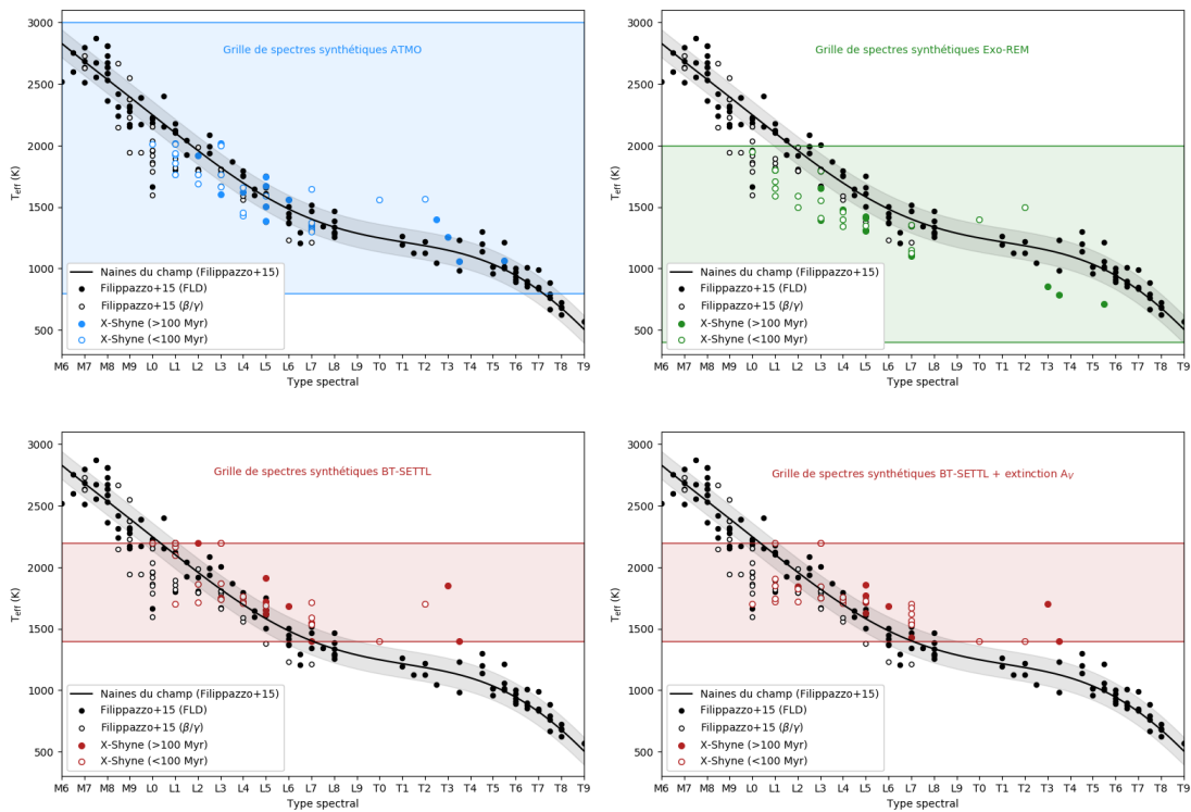
FIGURE 4.23 – Relation entre la T_{\text{eff}} et le type spectral. Les valeurs calculées par Filippazzo et al. (2015) sont représentées par les points noirs (pleins pour les objets du champ et vides pour les objets jeunes). La ligne noire correspond à la séquence des naines du champ ajustée par un polynôme de degré 6. Les T_{\text{eff}} estimées pour les objets de X-Shyne par ForMoSA sont représentées par des points bleus (grille ATMO), verts (grille Exo-REM) et rouges (grille BT-SETTL). La fenêtre en bas à droite montre la T_{\text{eff}} ajustée avec la grille BT-SETTL et l'ajout d'un paramètre libre d'extinction A_V . Les rectangles de couleur marquent les limites en T_{\text{eff}} des grilles.
