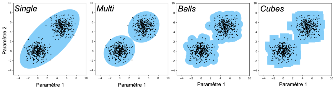
FIGURE 2.8 – Différentes méthodes de détermination du volume de prior.
