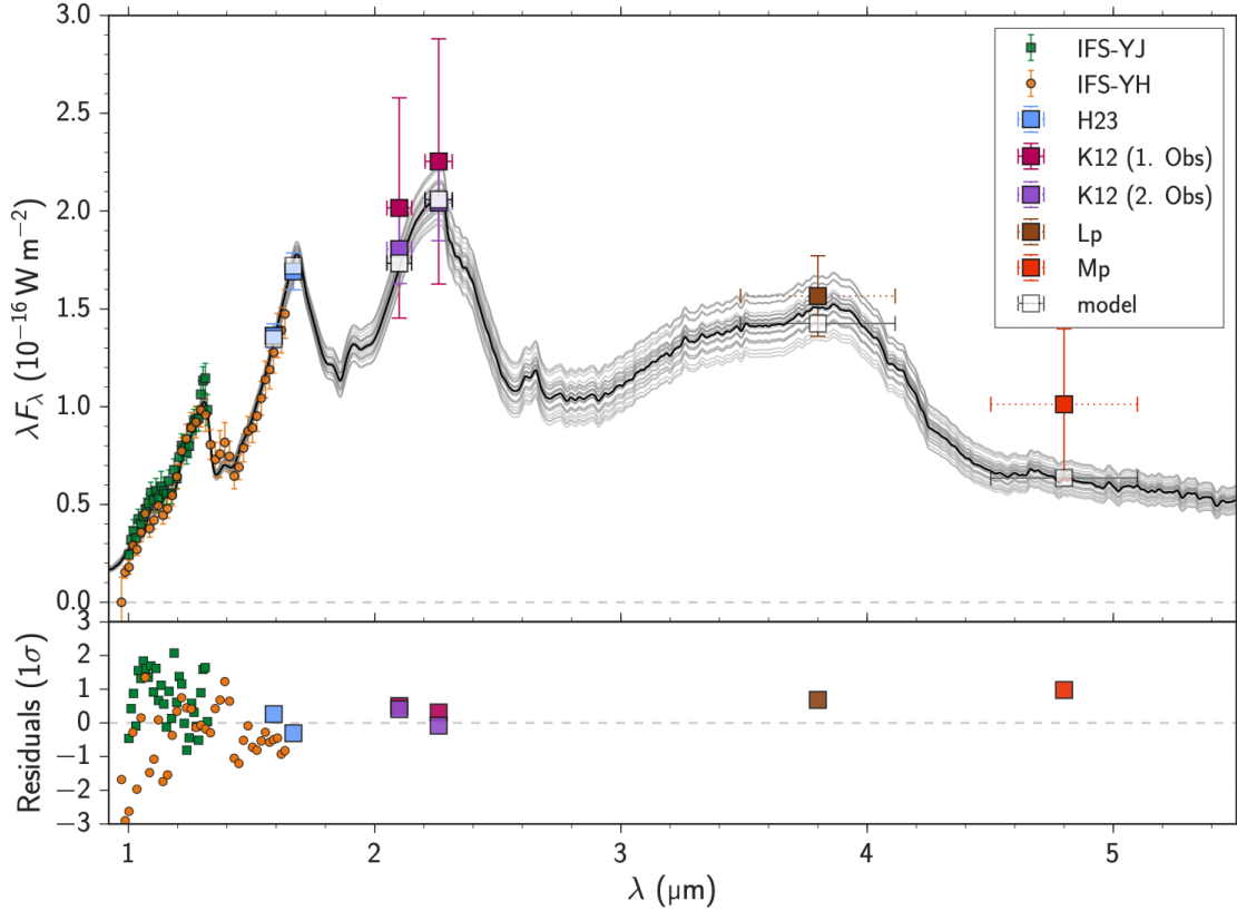
FIGURE 3.3 – Données spectroscopiques et photométriques recueillies avant les données SINFONI. Ces données ont été comparées aux spectres synthétiques de la grille BT-SETTL avec un code de MCMC pour caractériser son atmosphère. Figure issue de Cheetham et al. (2019).
