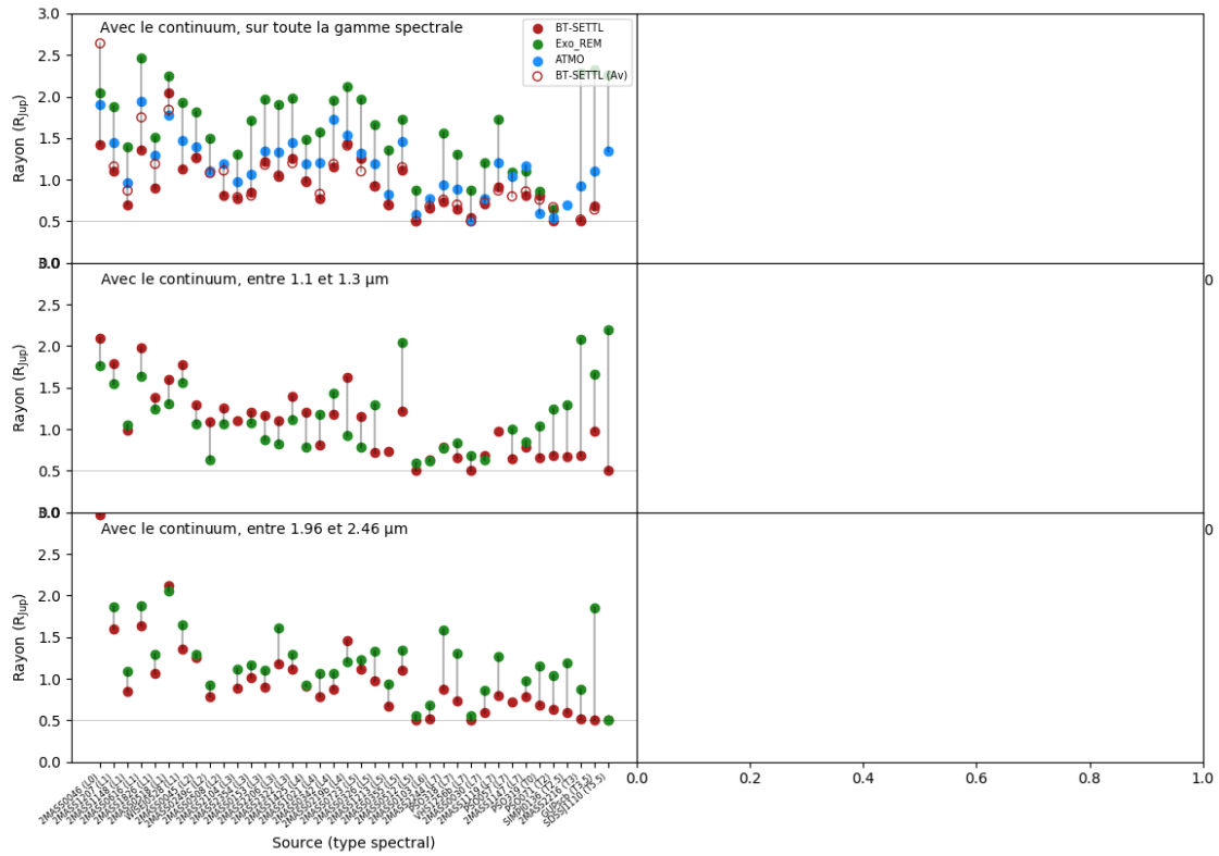
FIGURE B.5 – Suite de la Figure B.1 pour le rayon. Notons qu'ici la configuration sans le continuum n'a pas été testée.
