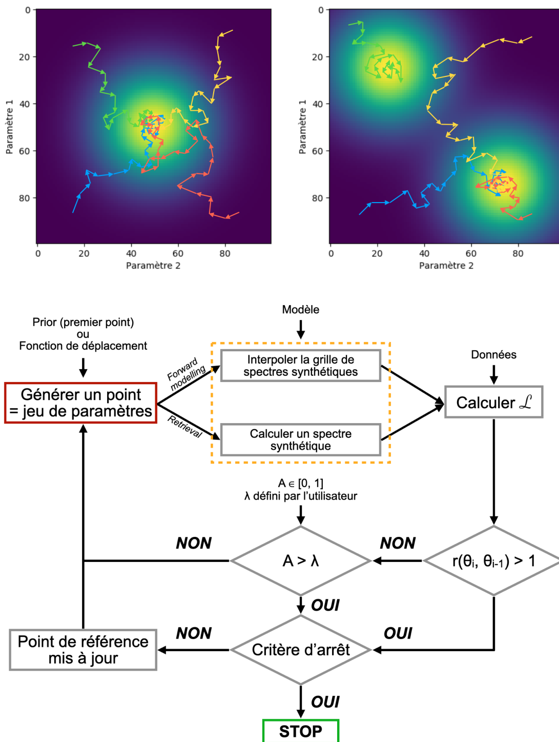
FIGURE 1.9 – En bas : Algorithme du MCMC. Le critère d'arrêt est choisi par l'utilisateur. Il peut s'agir, par exemple, d'un nombre d'itérations maximal ou d'un écart de vraisemblance minimum à atteindre entre deux itérations. En haut : Illustration des chaînes de Markov sur un espace de paramètres mono-modal (à gauche) et bi-modal (à droite). Ici, quatre chaînes sont représentées mais une application pratique peut en compter des centaines.
