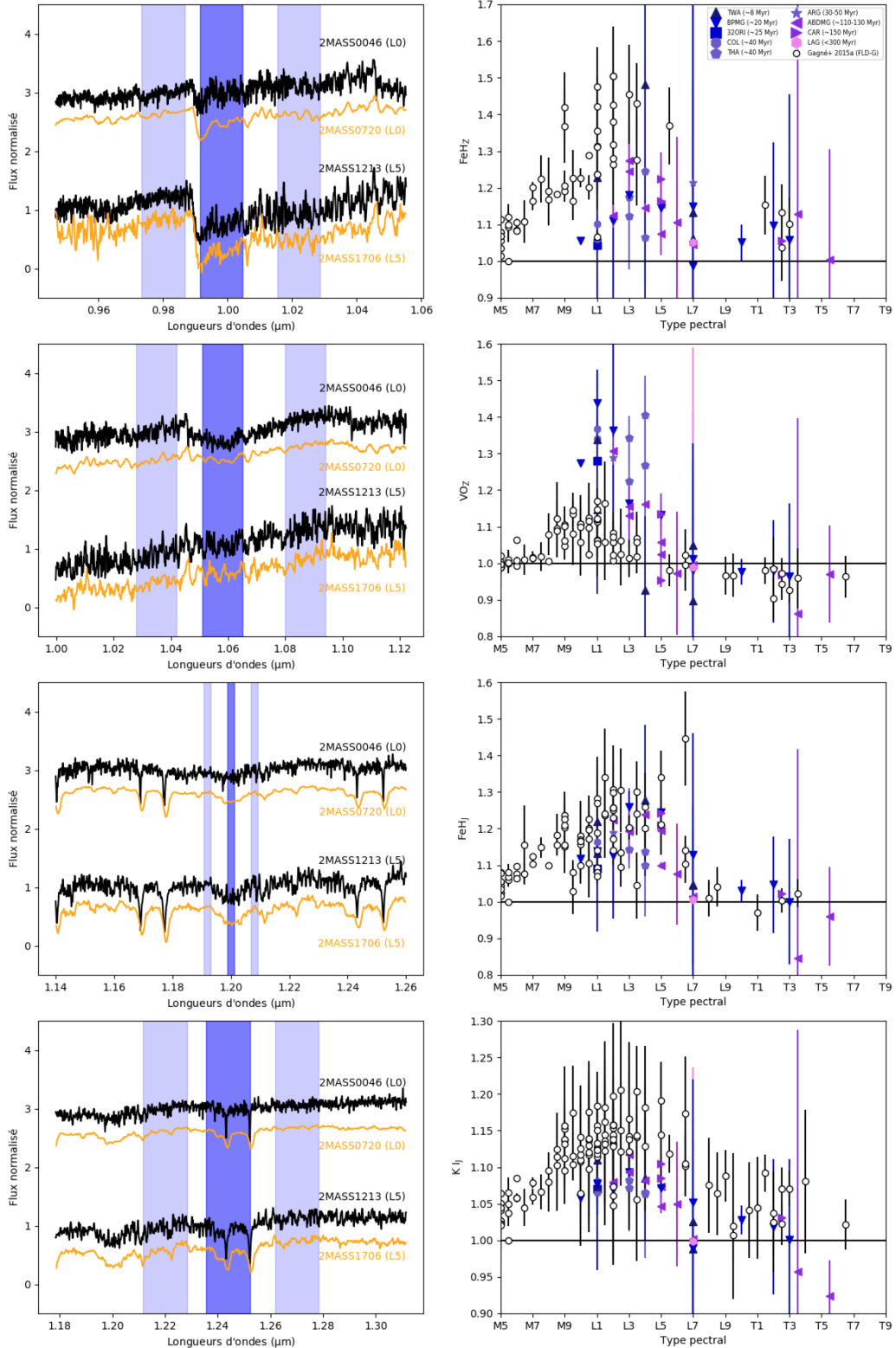
FIGURE 4.9 – À gauche : Fenêtres spectrales de la bande d'absorption moléculaire (bleu foncé) et du continuum (bleu clair) utilisées pour le calcul des indices de gravité. Des exemples de spectres X-Shyne sont donnés (en noir), ainsi que des spectres d'objets du champ (en orange) issus de la Montreal Spectral Library ( R \sim 750 ). À droite : Comparaison des indices de gravité calculés pour les objets de X-Shyne et de la Montreal Spectral Library. La ligne noire horizontale marque une valeur d'indice à 1, signifiant une absence de détection. De haut en bas : Indices FeH_z , VO_z , FeH_j et K_{ij} .
