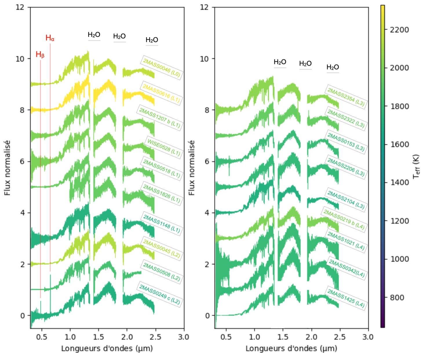
FIGURE 4.4 – Présentation des spectres X-Shyne (L0-L4).
