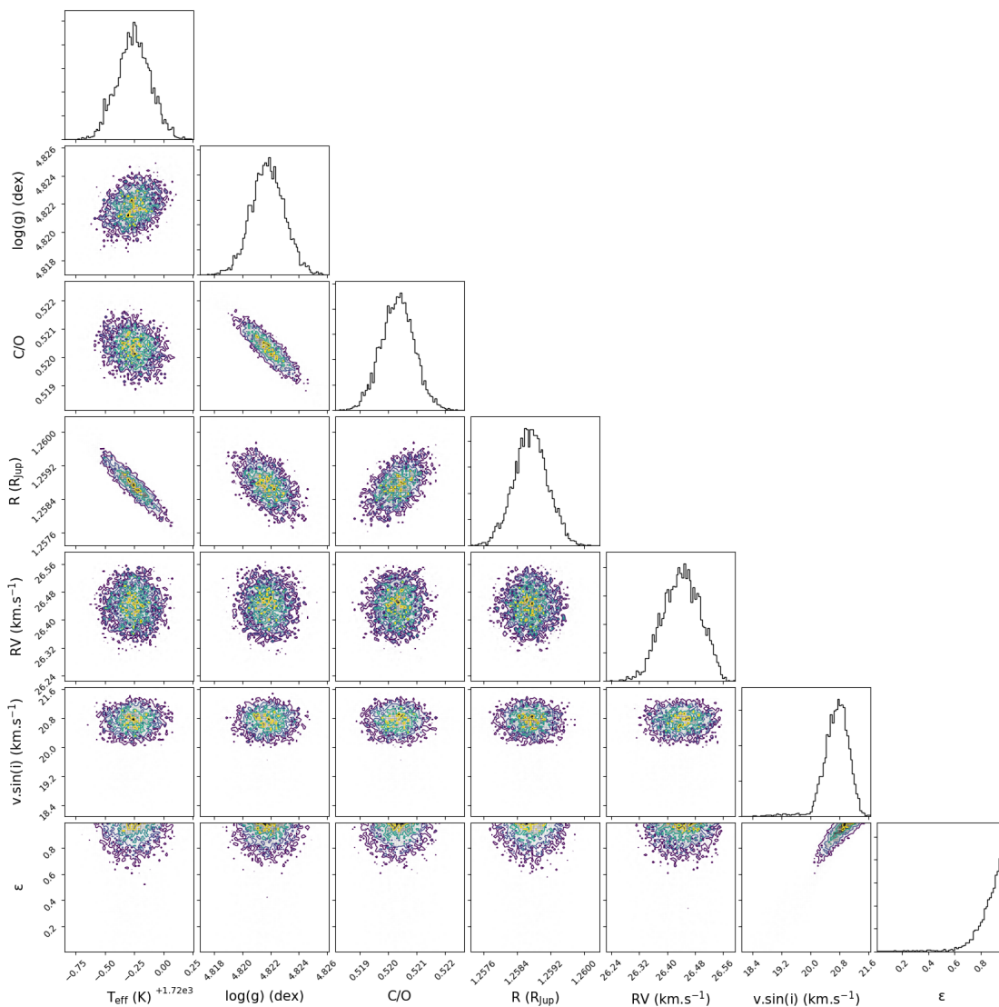
FIGURE 4.16 – Exemple de distributions postérieures pour tous les paramètres obtenus avec les modèles BT-SETTL. La source sélectionnée pour cet exemple est 2MASS0723.
