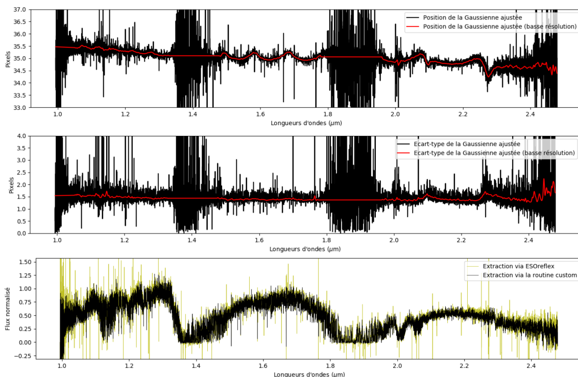
FIGURE 2.5 – En haut : Illustration des variations à basse résolution de la position des lois Gaussiennes utilisées pour extraire le flux de la trace. Au milieu : Illustration des variations à basse résolution de l'écart-type. En bas : Comparaison entre le spectre extrait par ESoreflex et celui extrait par cette routine.
