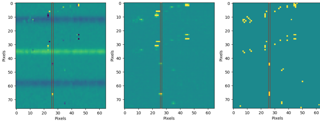
FIGURE 2.3 – Exemple d'identification des mauvais pixels dans une portion de la trace 2D fournie par ESOflex. À gauche : La trace de départ. Au centre : La carte de variation pixel à pixel. À droite : La carte de mauvais pixels. La colonne rouge servira d'exemple pour la Figure 2.4.
