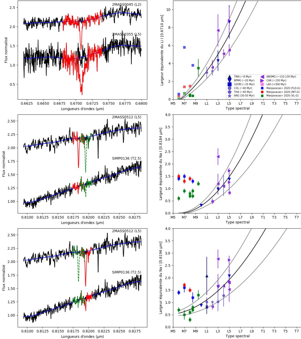
FIGURE 4.12 – Suite de la Figure 4.11. Les largeurs équivalentes reportées dans les figures de droite sont issues de Manjavacas et al. (2020) . Les coefficients des ajustements de Legendre (lignes noires et grises à droite) sont donnés dans la Table 4.5. De haut en bas : Largeurs équivalentes des raies du Li I à 0.6710 \mu\text{m} , Na I à 0.8184 \mu\text{m} , Na I à 0.8196 \mu\text{m} .
