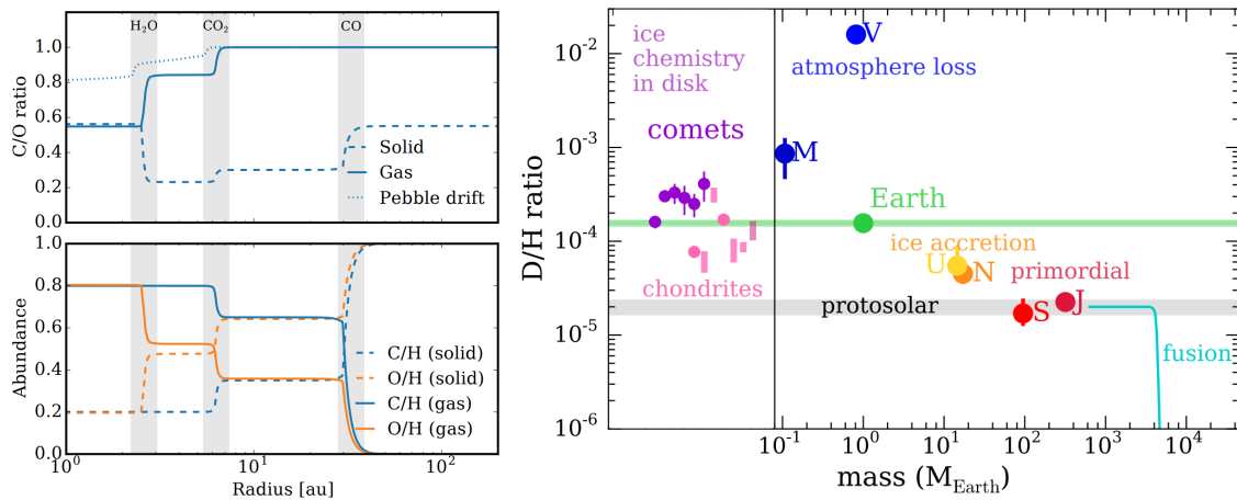
FIGURE 1.12 – En haut à gauche : Variation radiale du rapport C/O des gaz et des solides dans le disque. Les lignes des glaces de l'eau, du \text{CO}_2 et du \text{CO} sont illustrées en gris. La ligne pointillée illustre l'augmentation du C/O due à la migration des galets. En bas à gauche : Abondances de carbone et de l'oxygène comparées aux valeurs solaires. Figure tirée de Madhusudhan (2019). À droite : Rapport D/H des objets du système solaire en fonction de leur masse. On voit que Saturne et Jupiter présentent une abondance de deutérium solaire, tandis que les autres objets sont enrichis en deutérium. Figure tirée de Morley et al. (2019)
