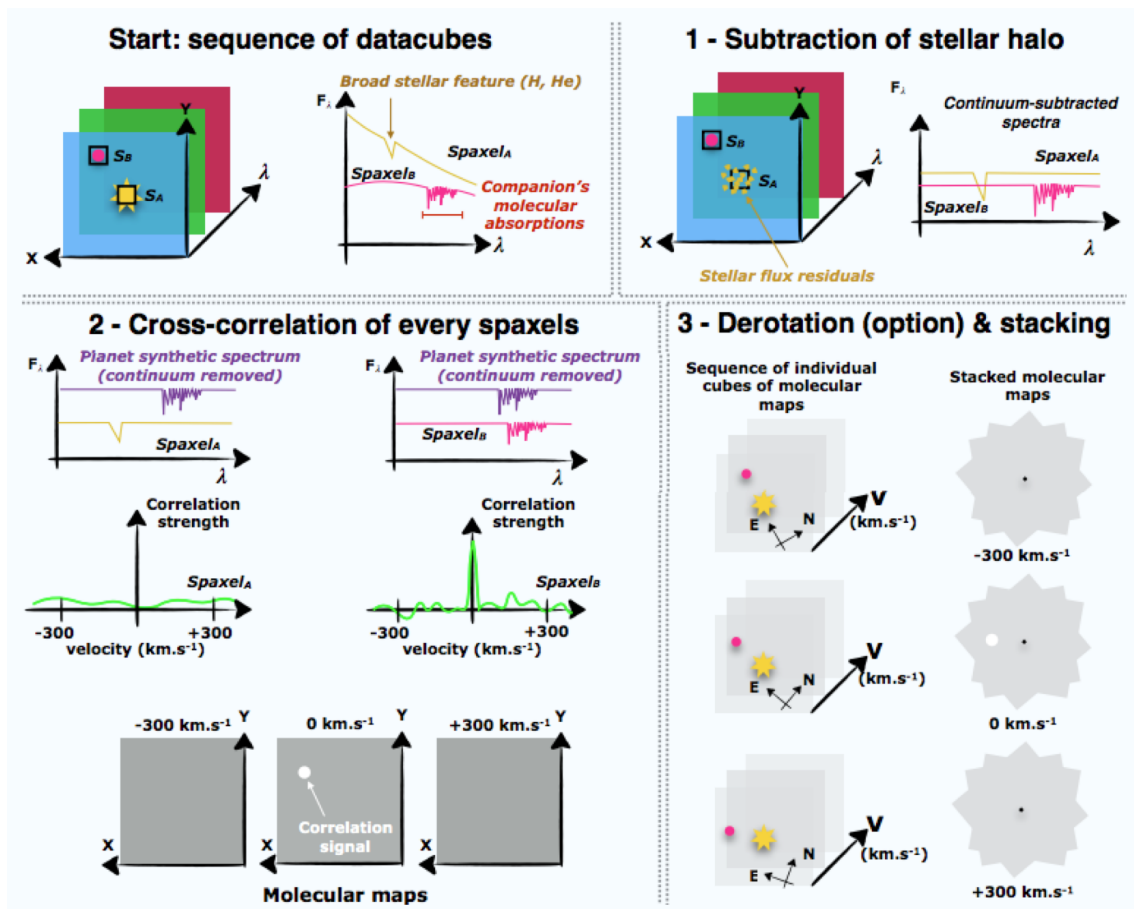
FIGURE 3.2 – Algorithme du molecular mapping. Ici, un système planétaire est observé avec l'étoile primaire (en jaune) et un compagnon (en rose) dans le champ. Le halo de la primaire est soustrait, pour permettre la corrélation croisée de chaque spaxel avec un spectre synthétique.
