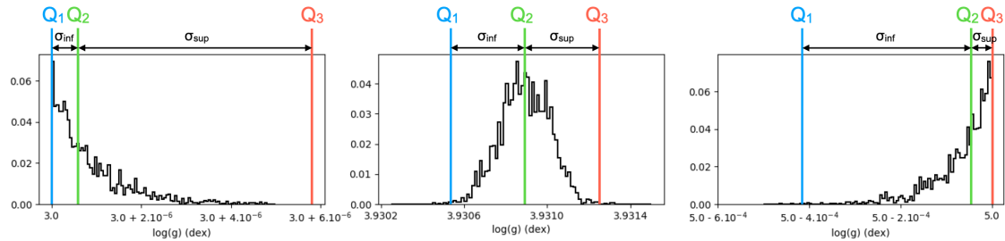
FIGURE 4.18 – Exemples de distributions postérieures de la gravité de surface obtenues avec la grille Exo-REM. Les quantiles à 0.15%, 0.5% et 99.85% calculés pour ces distributions sont représentés par les lignes verticales bleues, vertes et rouges respectivement.
