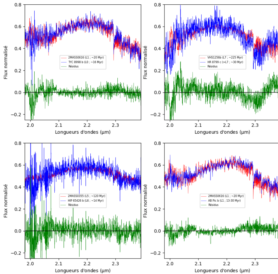
FIGURE 4.14 – Comparaison entre les spectres en bande K de TYC 8998 b (en haut à gauche), HR 8799 c (en haut à droite), HIP 65426 b (en bas à gauche) et AB Pic b (en bas à droite) et le spectre de X-Shyne qui minimise le \chi^2 . La courbe verte représente les résidus entre ces deux spectres.
