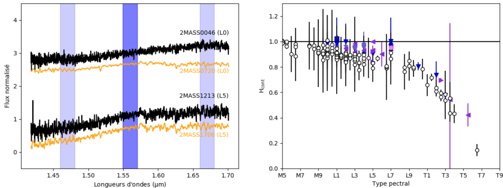
FIGURE 4.10 – Suite de la Figure 4.9 pour l'indice H_{cont} . La ligne noire horizontale marque une valeur d'indice à 1, signifiant, cette fois, que la pente côté bleu est parfaitement droite, et ainsi, que la forme de la bande H est triangulaire.
