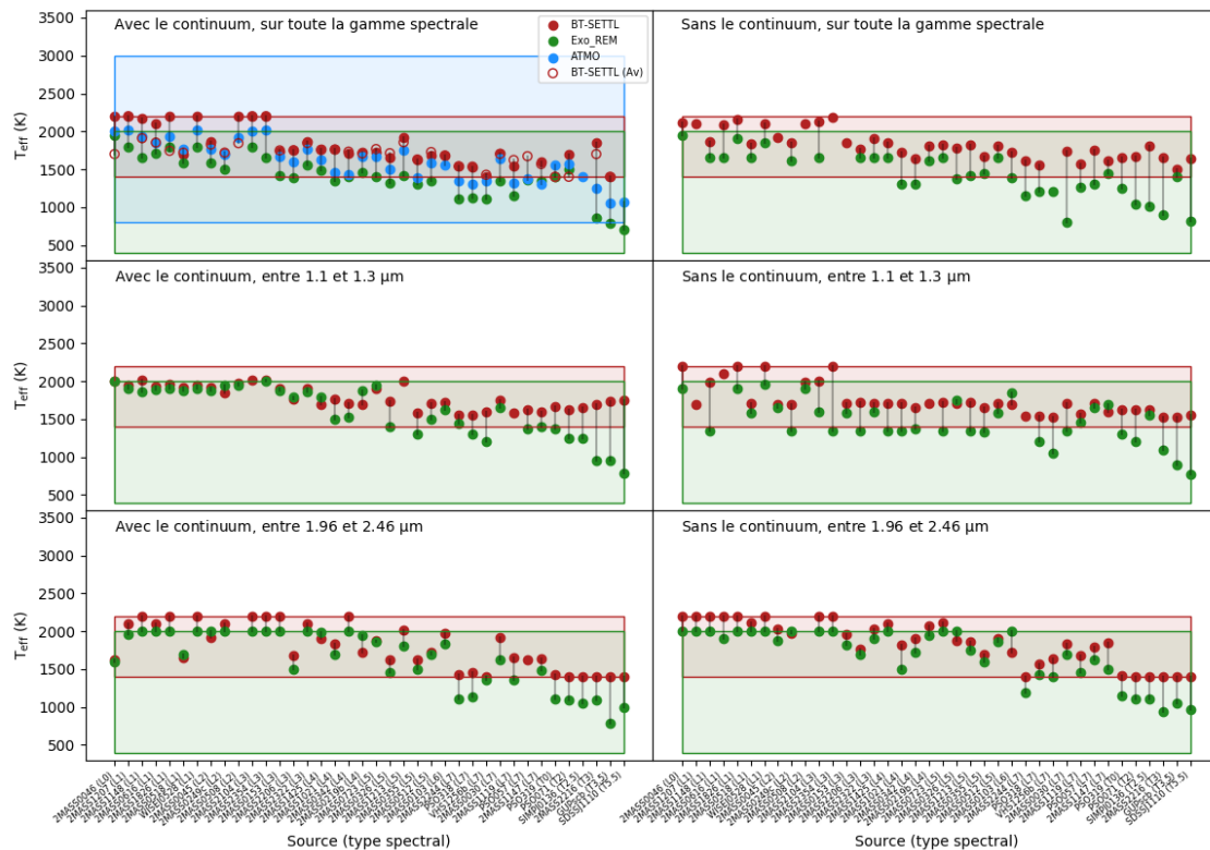
FIGURE B.1 – Estimation de la T_{\text{eff}} pour chaque source de la librairie X-Shyne. Six configurations d'ajustement sont testées ici. À gauche : Avec le pseudo-continuum. À droite : Sans le pseudo-continuum. De haut en bas : Sur toute la couverture spectrale, entre 1.1 et 1.3 \mu\text{m} , sur la bande K. Trois grilles de spectres synthétiques ont été utilisées : ATMO (en bleu), Exo-REM (en vert), BT-SETTL (en rouge). Les rectangles de couleur représentent les limites de ces grilles.
