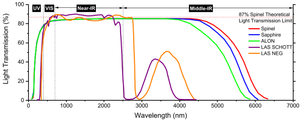
Figure I-38. Transmission de spinelles transparentes usuelles et de verres silicates [46]
