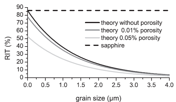
Figure I-23. Influence de la microstructure sur le facteur RIT d'Al 2 O 3 en fonction de la taille des grains (pores de 100 µm) [52]
