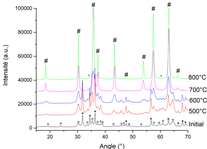
Figure II-38. Diffractogrammes des poudres à l'issue du pré-traitement appliqué sous air à la température indiquée pour 2h (initial en noir, 500°C en rouge, 600°C en bleu, 700°C en magenta et 800°C en vert) (# ZnGa_2O_4 ICDD 00-038-1240, ' pics secondaires dus aux raies L_\alpha du W et K_\beta du Cu, * ZnO ICDD 00-036-1451 et ° Ga_2O_3 ICDD 00-043-1012)
