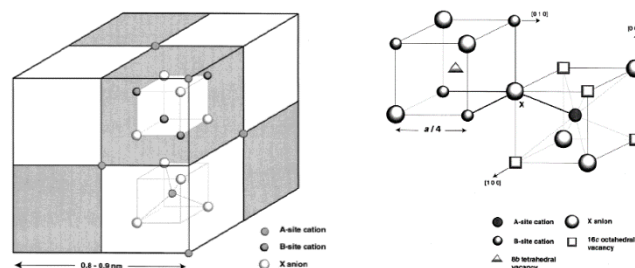
Figure I-36. Structure générale des spinelles [87]
