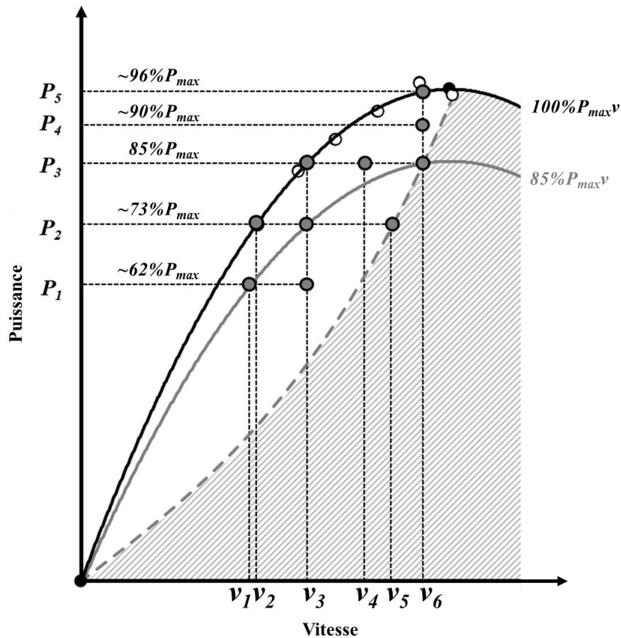
Figure 35. Relation puissance-vitesse individuelle typique représentant 100 % (courbe noire) et 85 % (courbe grise) de puissance relative à la condition de vitesse ( \%P_{\max}v ). Les points gris représentent les 10 conditions force-vitesse-puissance dans lesquelles les tests de squat jumps répétés jusqu'à l'épuisement étaient réalisés.
