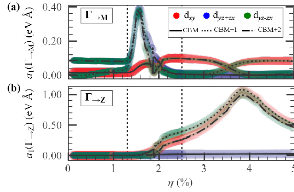
FIGURE 4.13 – Évolution du coefficient linéaire a_1 en fonction de la contrainte biaxiale \eta , avec une projection sur les orbitales d_{xy} , d_{yz+zx} et d_{yz-zx} , et le long de (a) la direction \Gamma \rightarrow M et \Gamma \rightarrow Z . Les résultats obtenus pour la direction \Gamma \rightarrow M sont identiques à ceux de la direction \Gamma \rightarrow X .
