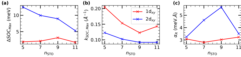
FIGURE C.9 – Variation des propriétés spin-orbite des bandes 1d_{xy} (rouge) et 2d_{xy} (bleu) en fonction de l'épaisseur de STO n_{STO} : (a) Variation de la différence d'énergie maximale entre les deux états de spin \Delta SOC_{Max} (au niveau de l'anticroisement). (b) Variation du vecteur d'onde k_{SOC,Max} pour lequel \Delta SOC_{Max} est atteint. (c) Variation du coefficient Rashba linéaire \alpha_R .
