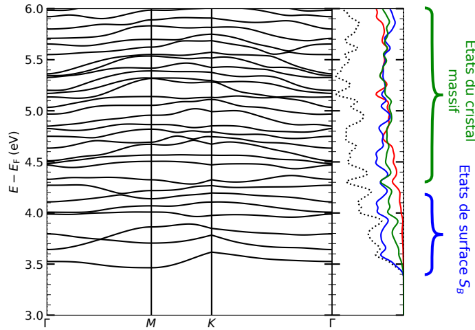
FIGURE 5.16 – Structure de bandes (gauche) et densité d'états (droit) projetés sur les plans atomiques de HfO 2 (b) pour une épaisseur de 3 monocouches. La contribution de la surface S_A est donnée en rouge, celle de la surface S_B en bleu, tandis que la contribution des autres plans est en vert.
