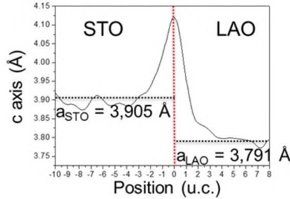
FIGURE 3.14 – Variation du paramètre de maille c dans \text{LAO}_{(8)}/\text{STO} obtenue par mesures HRSTEM. Les lignes noires correspondent aux paramètres de maille des cristaux massifs de STO ( a_{\text{STO}} = 3.905 \text{ \AA} ) ou de LAO ( a_{\text{LAO}} = 3.791 \text{ \AA} ). La ligne rouge en pointillés indique l'interface de LAO/STO. [Rubi 2020]
