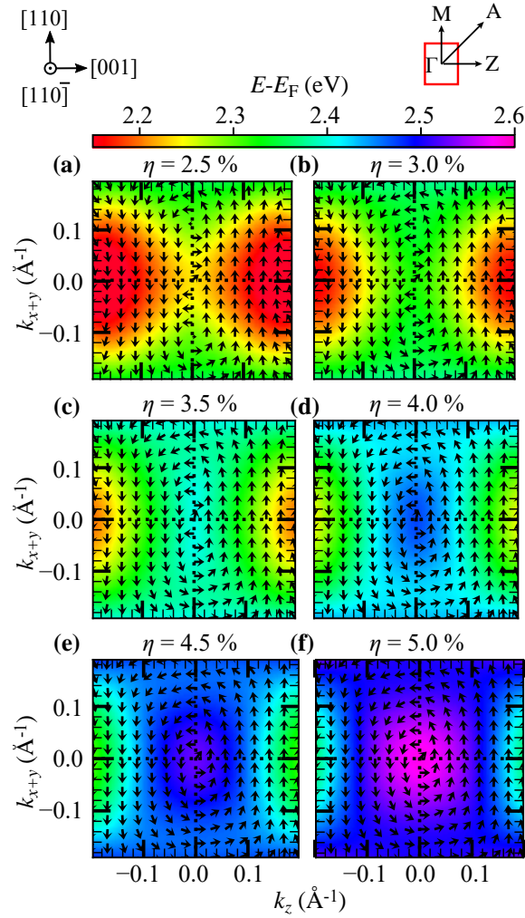
FIGURE 4.15 – Textures de spin de la bande CBM+1 en fonction de l'énergie dans le plan (\Gamma - Z - A - M) près du point \Gamma et perpendiculaire à la polarisation électrique ([1\bar{1}0]) de la phase Amm2 pour différents états de contrainte : (a) \eta = 2.5\% , (b) \eta = 3\% , (c) \eta = 3.5\% , (d) \eta = 4\% , (e) \eta = 4.5\% et (f) \eta = 5\% .
