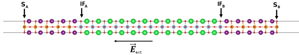
FIGURE 3.20 – Schéma représentant la géométrie symétrique utilisée dans les calculs DFT. les atomes Sr, La, Ti, Al et O sont respectivement représentés par les sphères de couleur verte, grise, bleue, orange et rouge. Les deux interfaces et les deux surfaces sont différenciées en IF A , IF B , S A et S B . La direction du champ électrique appliqué E_{ext} est indiquée.
