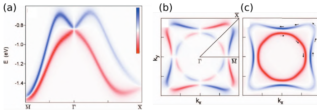
FIGURE 5.2 – (a) États électroniques de surface résolus en spin, correspondant aux états 6p de Bi sur BaTiO 3 pour un état de polarisation donné P_{\uparrow} . Projection radiale (b) et tangentielle (c) de la polarisation en spin dans la zone de Brillouin des états de surface de Bi sur BaTiO 3 pour un état de polarisation P_{\uparrow} et pour une isoénergie de -1.30 eV [Mirhosseini 2010].
