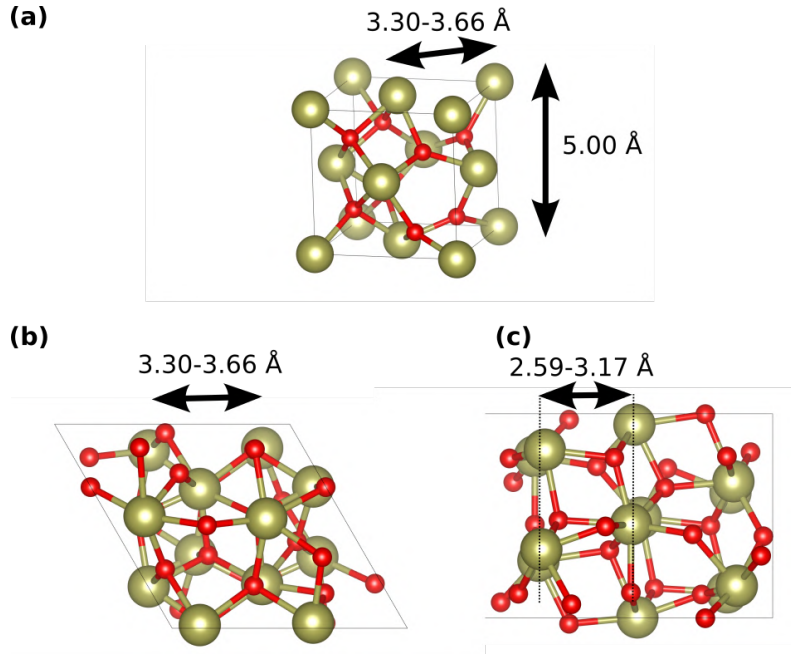
FIGURE 5.6 – Structures atomiques de (a) la cellule primitive et la cellule hexagonale vue du plan (b) (111) et (c) (01 \bar{1} ) de HfO 2 dans sa phase orthorhombique Pca2_1 .
