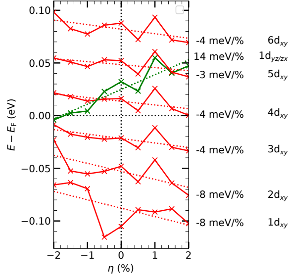
FIGURE 3.28 – Variation de la position en énergie par rapport au niveau de Fermi des bandes de conduction du système au point \Gamma en fonction de l'épaisseur de LAO, avec n_{STO} = 5 monocouches de STO. La couleur rouge correspond aux bandes de caractère d_{xy} , tandis que la couleur verte représente les bandes de caractère d_{yz} et d_{zx} .
