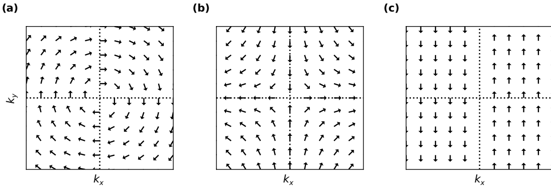
FIGURE 1.7 – Texture de spin d'un couplage spin-orbite type (a) Bychkov-Rashba, (b) Dresselhaus 2D et (c) persistant. Les flèches représentent la direction du moment magnétique suivant les axes k_x et k_y pour un état de spin.
