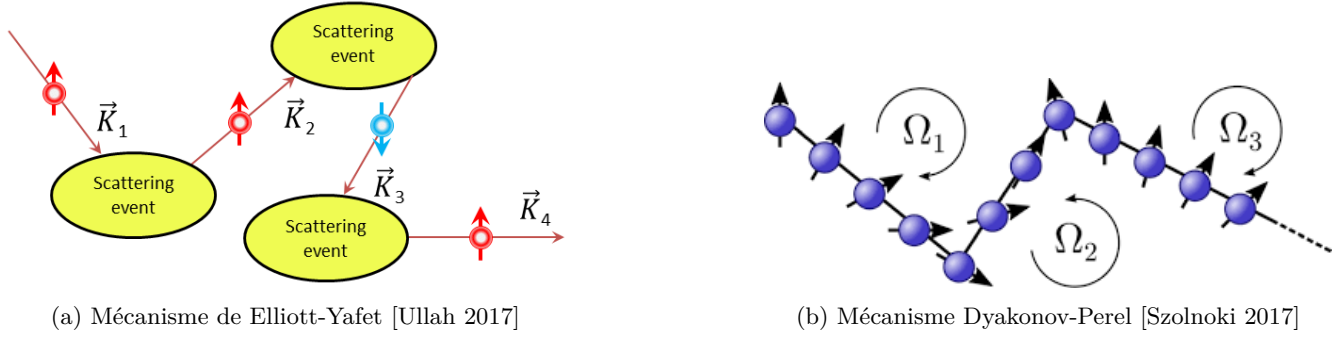
FIGURE 1.11 – (a) Mécanisme de Elliott-Yafet et (b) mécanisme Dyakonov-Perel (b).
