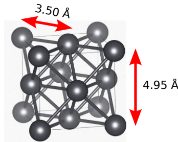
FIGURE 5.18 – Structure atomique du plomb dans sa phase cristallographique Fm – 3 m .
