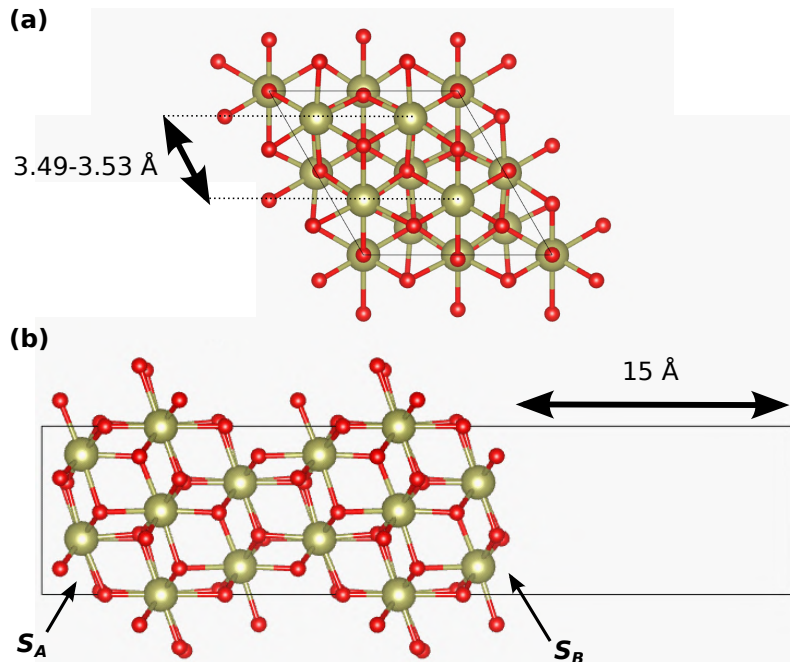
FIGURE 5.10 – Structure atomique d'une couche mince de HfO 2 dans la phase P3m (a) vu de dessus, (b) vu sur le côté.
