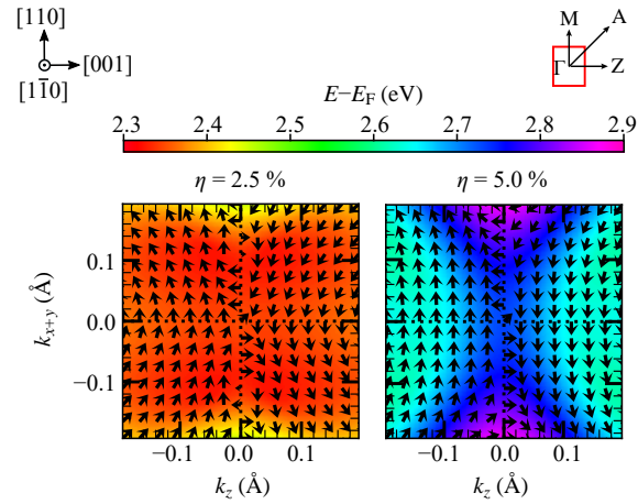
FIGURE 4.16 – Textures de spin de la bande CBM+2 en fonction de l'énergie dans le plan (\Gamma - Z - A - M) près du point \Gamma et perpendiculaire à la polarisation électrique (orientée selon l'axe [1\bar{1}0]) de la phase Amm2 pour différents états de contrainte, (a) \eta = 2.5\% , (b) \eta = 5\% .
