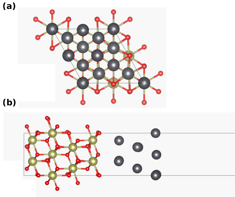
FIGURE 5.20 – Structure atomique d'une interface entre une couche mince de HfO 2 dans la phase P3m et le plomb (a) vu de dessus, (b) vu sur le côté.
