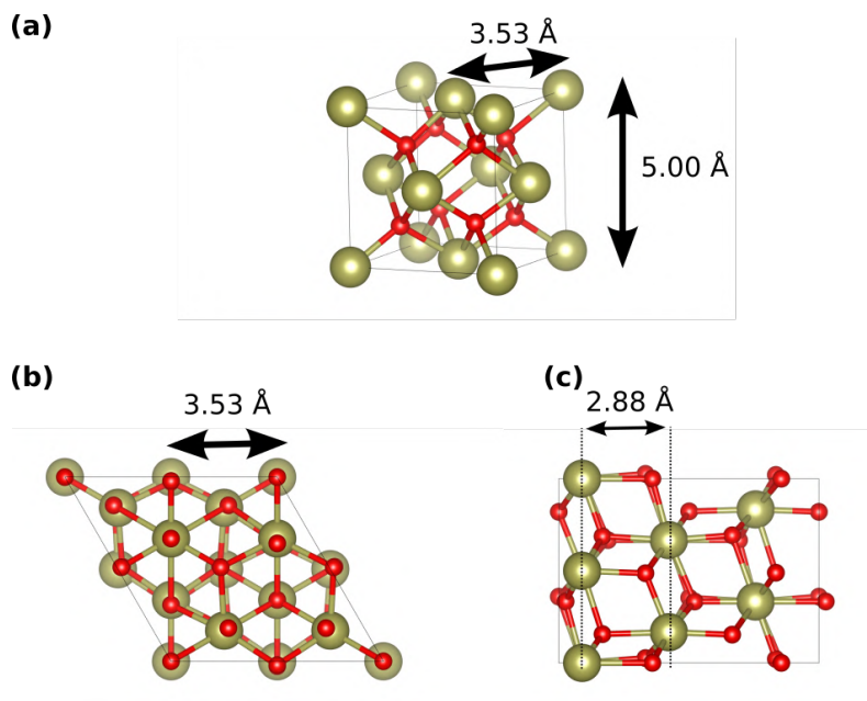
FIGURE 5.3 – Structures atomiques de (a) la cellule primitive et la cellule hexagonale vue du plan (b) (111) et (c) (01 \bar{1} ) de HfO 2 dans sa phase rhombohedrale R3m .
