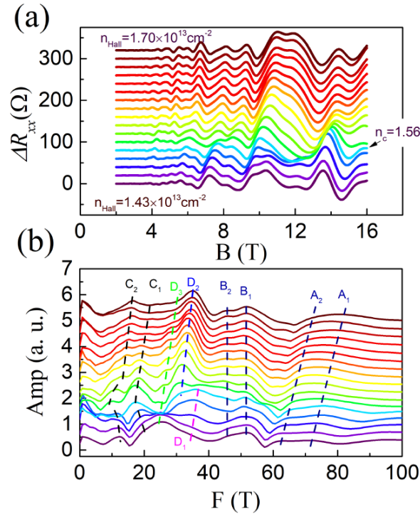
FIGURE 3.13 – (a) Variation de la résistivité longitudinale \Delta R_{xx} en fonction du champ magnétique pour différentes densités de Hall. (b) Transformé de Fourier de \Delta R_{xx} en fonction de 1/B . Les lignes en pointillés indiquent les pics de fréquence des oscillations. [Yang 2018]
