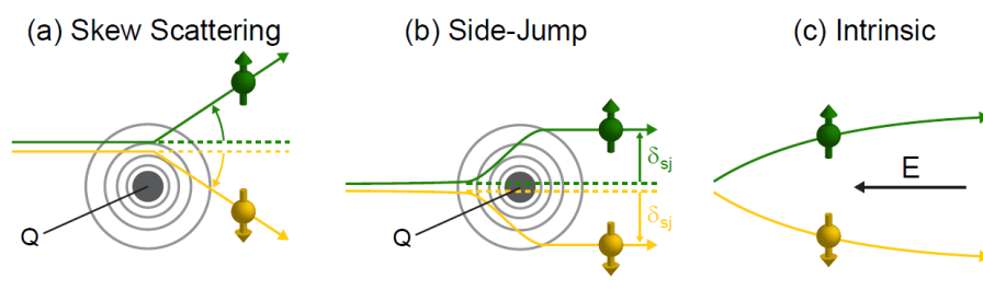
FIGURE 1.9 – Schéma de principe des trois mécanismes responsables de l'effet Hall de spin : (a) Diffusion de Mott ( skew-scattering ou Asymmetric scattering ), (b) Mécanisme dit side-jump et (c) Mécanisme intrinsèque. Image provenant de [Czeschka 2011]
