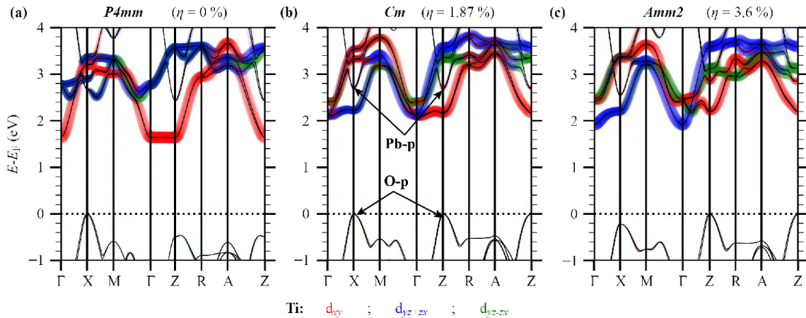
FIGURE 4.10 – Structures de bandes associées aux phases (a) tétragonale P4mm pour \eta = 0 \% , (b) monoclinique Cm pour \eta = 1.87 \% et (c) orthorhombique Amm2 pour \eta = 3.6 \% . La contribution des orbitales d des atomes de titane est donnée en couleur. Afin de faciliter la comparaison entre les structures de bandes des différentes phases cristallographiques, nous avons conservé la notation des points de haute de symétrie de la phase P4mm pour toute les phases.
