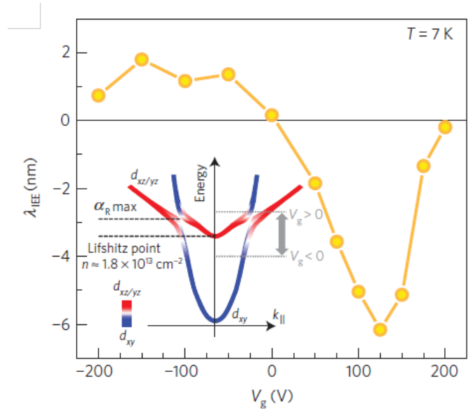
FIGURE 3.10 – Variation de la constante \lambda_{IREE} de l'effet Rashba-Edelstein inverse dans le gaz 2D d'électrons dans LAO/STO via la tension de grille. L'encart est une représentation de la structure de bandes du gaz 2D. [Lesne 2016]
