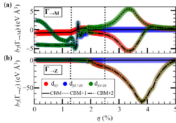
FIGURE 4.14 – Évolution du coefficient cubique b_3 en fonction de la contrainte biaxiale \eta , avec une projection sur les orbitales d_{xy} , d_{yz+zx} et d_{yz-zx} , et le long de (a) la direction \Gamma \rightarrow M et \Gamma \rightarrow Z . Les résultats obtenus pour la direction \Gamma \rightarrow M sont identiques à ceux de la direction \Gamma \rightarrow X .
