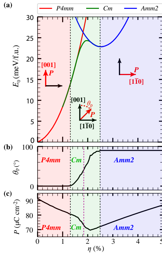
FIGURE 4.9 – (a) Energie totale de \text{PbTiO}_3 calculée pour les phases tétragonale ( P4mm ), monoclinique ( Cm ) et orthorhombique ( Amm2 ) en fonction de la contrainte \eta . Les flèches rouges représentent l'orientation de la polarisation électrique dans la base [1\bar{1}0] , [001] . (b) Angle \theta_p entre la polarisation électrique \mathbf{P} et l'axe z [001] et (c) norme de \mathbf{P} calculés pour la phase cristallographique la plus stable dans \text{PbTiO}_3 en fonction de la contrainte biaxiale \eta . La ligne en trait pointillés violette indique la valeur de la contrainte pour laquelle la polarisation électrique est alignée avec l'axe [1\bar{1}1] .
