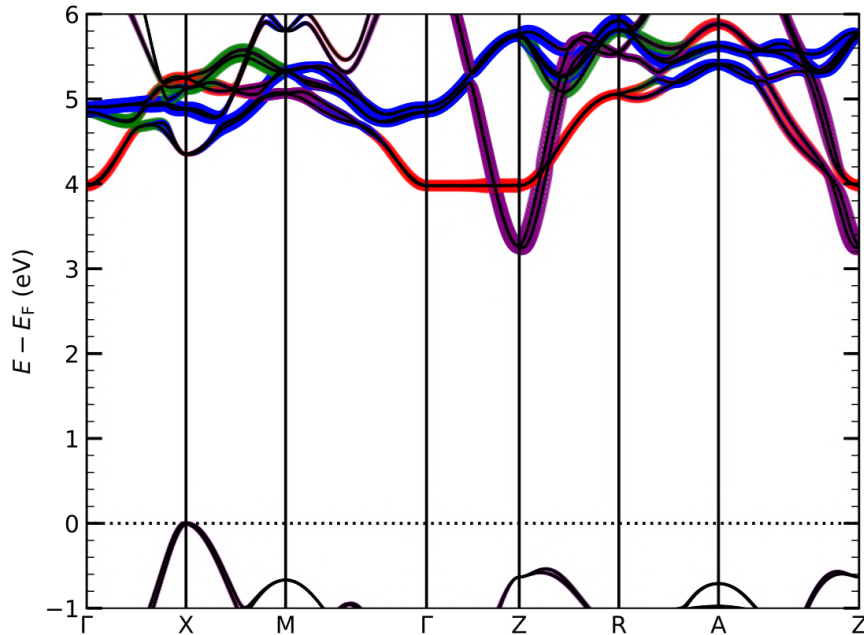
FIGURE 4.20 – Structure de bandes de la phase d'équilibre de \text{PbTiO}_3 , obtenue en déterminant les fonctions de Wannier à partir d'un calcul type GW, en utilisant l'algorithme \text{EVGW}_0 . La couleur représente respectivement les contributions des orbitales d_{xy} (rouge), d_{yz} (verte) et d_{zx} (bleue) du titane et p_z (violette) des atomes de plomb.
