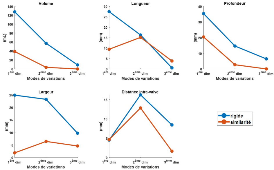
FIGURE 6.7 – Variations selon les trois premières dimensions de cinq caractéristiques de forme définies en chaque maillage entre les formes estimées à -2\sigma et à +2\sigma . Les caractéristiques sont définies dans la Figure 6.5.
