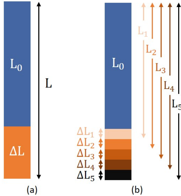
FIGURE 2.3 – Calcul de la déformation Lagrangienne (a) et de la déformation naturelle (b) illustré en 1D. Image inspirée de (Amzulescu et al., 2019).
