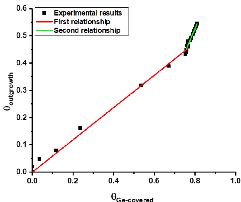
Figure 2 Fraction de l'excroissance en fonction du taux de couverture des zones de reconstruction pendant la croissance à 300K. Le résultat expérimental indiqué par les carrés noirs montre deux relations linéaires indiquées par les lignes solides rouges et vertes, respectivement.
