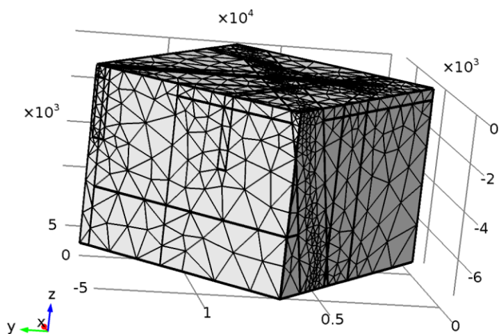
Maillage 1
