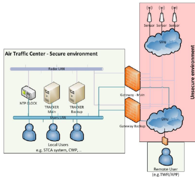
FIGURE 1.1 – Représentation schématique de l'isolation du réseau
