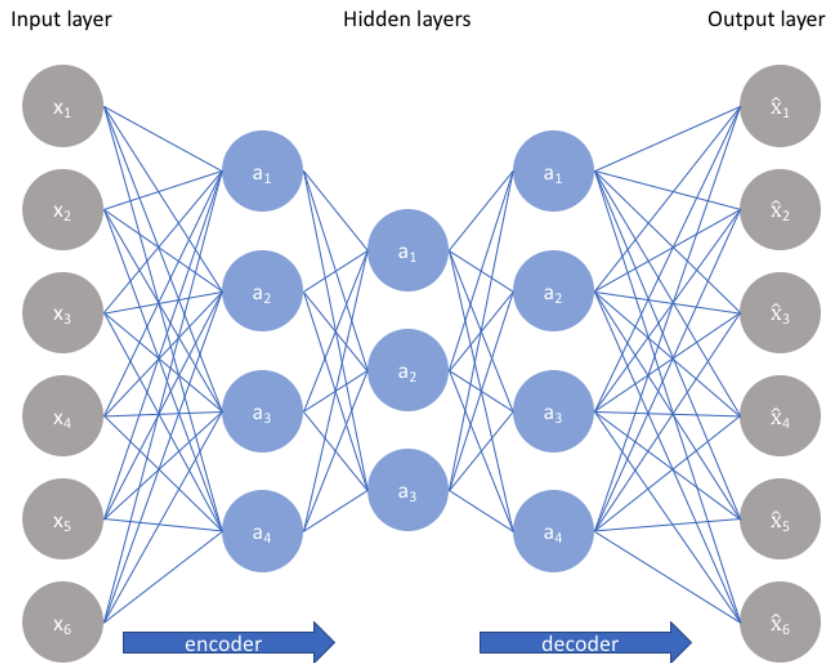
FIGURE 5.6 – Modèle d'auto-encodeur
