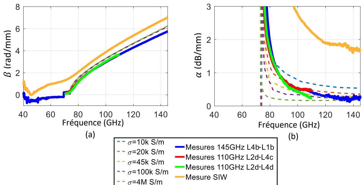
Figure II-61 : (a) Constante de propagation \beta et (b) constante d'atténuation \alpha mesurés de guides SIW classique (traits pleins oranges) et PAFSWSIW (traits pleins rouges, bleus et verts) pour une fréquence de coupure de 75 GHz. Des résultats de simulation sont tracés en traits pointillés pour différentes valeurs de conductivité verticale, de 10 kS/m à 4 MS/m.
