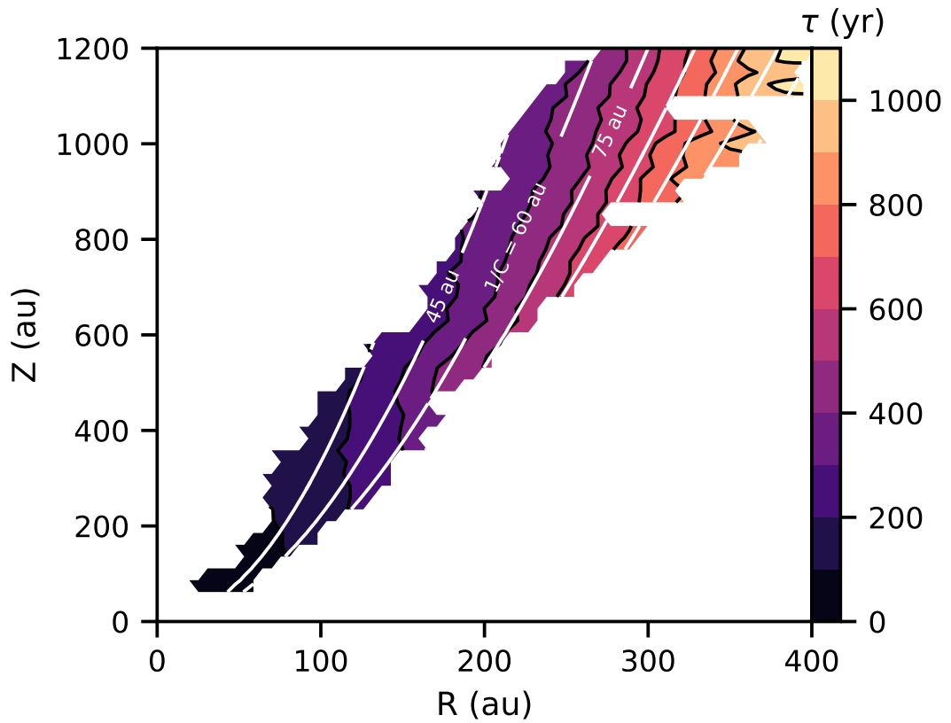
Fig. 6.1.: En couleur est représenté l'âge dynamique \tau = Z/V_Z déterminé à partir de la carte de V_Z . Les lignes blanches correspondent à des courbes paraboliques avec 1/C variant de 30 à 135 au, par sauts de 15 au.
