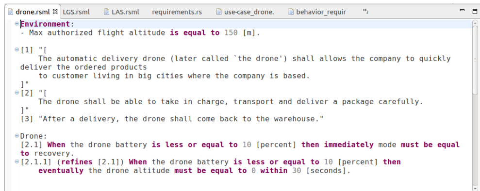
FIGURE C.5 : Exemple du DSL RSML en pratique
