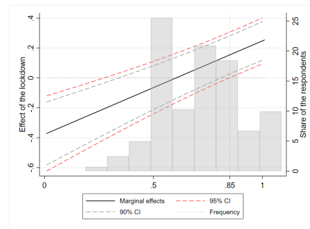
(d) Both outside (N=161)
