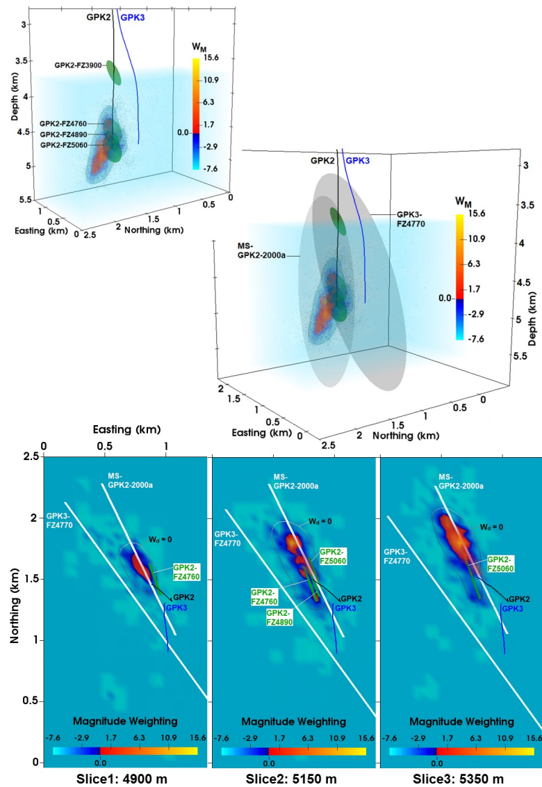
FIGURE 6.2 – PPFN appliquée au grand jeu de données du nuage sismique de GPK2 et zones de failles proches de GPK2. En haut à gauche : PPFN-Magnitude avec F = 1/2 en carte couleur, PPFN-Distance avec d = 50 m en contour au seuil de W_d = 0 et les quatre zones de failles identifiées au puits en plans verts. Au milieu à droite : le plan MS-GPK2-2000a obtenu par analyse du cluster sismique de GPK2 et la zone de faille GPK3-FZ4770, tous deux déterminés par Sausse et al. (2010), sont ajoutés et représentés par des plans gris. En bas : trois sections à différentes profondeurs, des plans de failles représentés sous forme de segments verts et blancs. Pour l'ensemble des graphes, les points noirs représentent les séismes, la courbe noire représente la trajectoire de GPK2 et la courbe bleue, celle du puits GPK3. La position, l'orientation et la taille des plans de failles sont tirés de SAUSSE et al. (2010).
