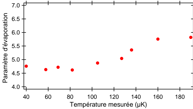
FIGURE 7.8 – Évolution du paramètre d'évaporation \eta en fonction de la température mesurée du nuage.
