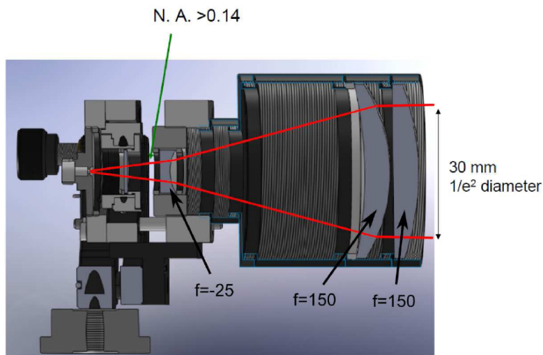
FIGURE 5.7 – Dispositif de mise en forme et de contrôle de polarisation des faisceaux du MOT 3D. La figure est extraite de [104].
