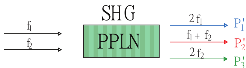
FIGURE 2.6 – Génération des fréquences de refroidissement de potassium : le processus non linéaire génère la deuxième harmonique de chaque fréquence et leur somme de fréquence.
