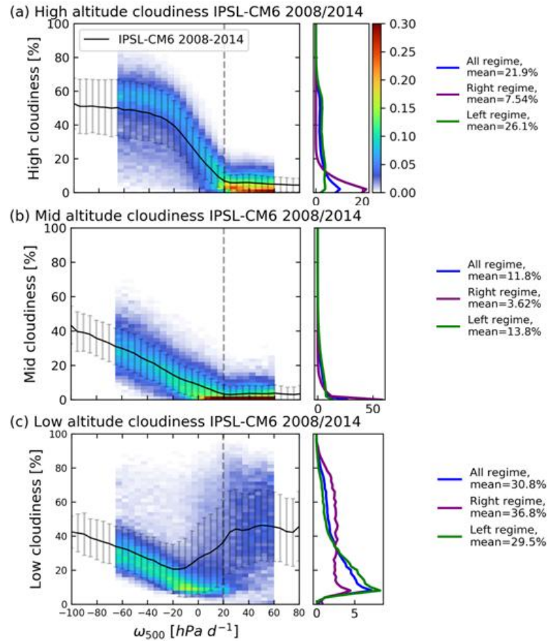
Figure 4.13 : Histogramme normalisé montrant la distribution de la couverture en nuages d'altitude (a) élevée [%], (b) moyenne [%] et (c) faible [%] et la PDF de \omega_{500} [ \text{hPa/d} ] pour le modèle IPSL-CM6. Les plages de \omega_{500} contenant moins de 1500 occurrences absolues pour CESM1 et IPSL-CM6 sont masquées (blanc). La courbe noire en pointillé représente la distribution sur la période 2008-2014 selon les simulations IPSL-CM6. Les barres d'erreur indiquent l'écart type sur 7 ans. Les PDFs de la couverture en nuages d'altitude (a) élevée, (b) moyenne et (c) faible sont situées à droite de chaque histogramme normalisé. La résolution des données est de 2^\circ \times 2^\circ \times 1 mois.
