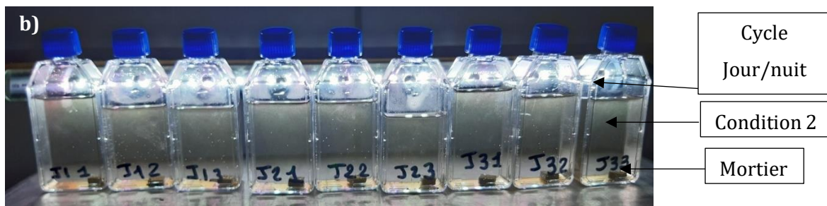
Figure 37. Dispositif expérimental de la dissolution du mortier immergé dans la condition 1 (a) et condition 2 (b).
