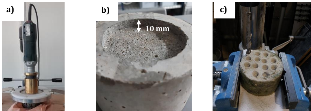
Figure 21. Grignoteuse (a) , éprouvette de mortier ( \varnothing 110 \text{ mm} \times H 50 \text{ mm} ) après grignotage à 10 mm de profondeur (b) , perceuse à colonne (c)
