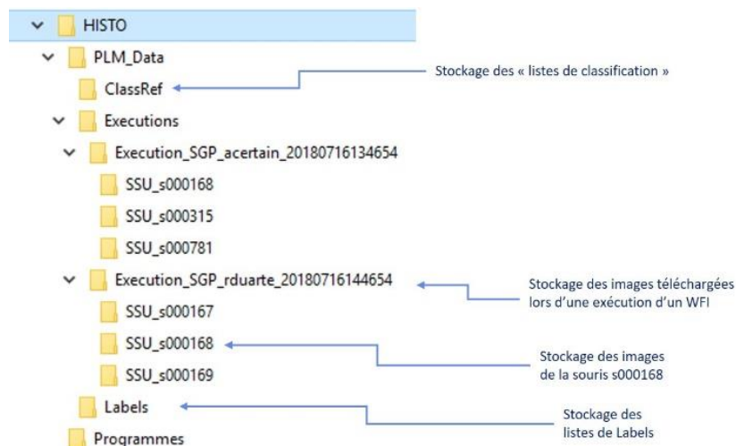
Figure 125 Arborescence prédéfinie du stockage local des fichiers échangés entre l'application Matlab et le système BMS-LM
