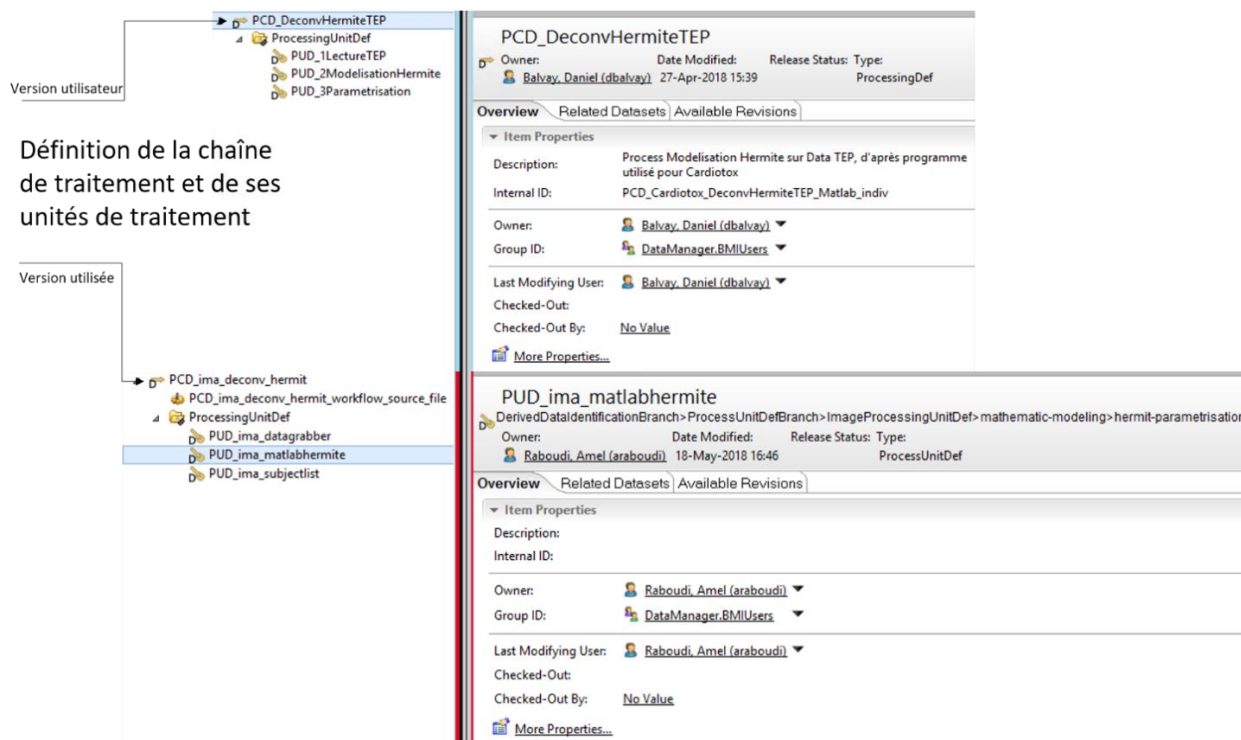
Figure 141 Les objets représentant le workflow Hermite (FTPH) dans le système BMS-LM
