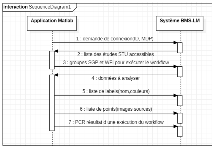
Figure 126 Diagramme de séquence des échanges entre le système BMS-LM et l'application Matlab d'apprentissage histologique
