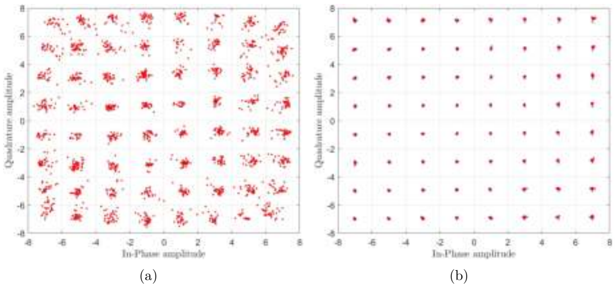
Figure 12 : Constellation des données I/Q : (a) Sans DPD; (b): Avec DPD
