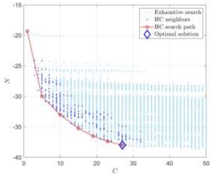
Figure 5 : Algorithme HC avec \alpha = 0.05
