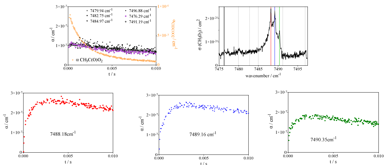
Figure 65: Spectre d'absorption du radical CH 3 O 2 mesuré dans le proche infrarouge, d'après Faragó et al. [90] (en haut à droite) et décroissances cinétiques mesurées à partir de la photolyse à 351 nm de [CH 3 CHO] = 1,66 × 10 15 / [Cl 2 ] = 4,5 × 10 15 cm -3 . Les graphiques en bas montrent les décroissances mesurées sur les trois raies du spectre. Le graphique en haut à gauche montre toutes les décroissances mesurées aux longueurs d'onde indiquées par des lignes verticales dans le spectre (le signal mesuré à 7476,29 cm -1 est utilisé dans Figure 67 comme exemple). La décroissance de CH 3 C(O)O 2 est donnée à titre indicatif sous forme de cercles orange dans le même graphique (axe y à gauche).
