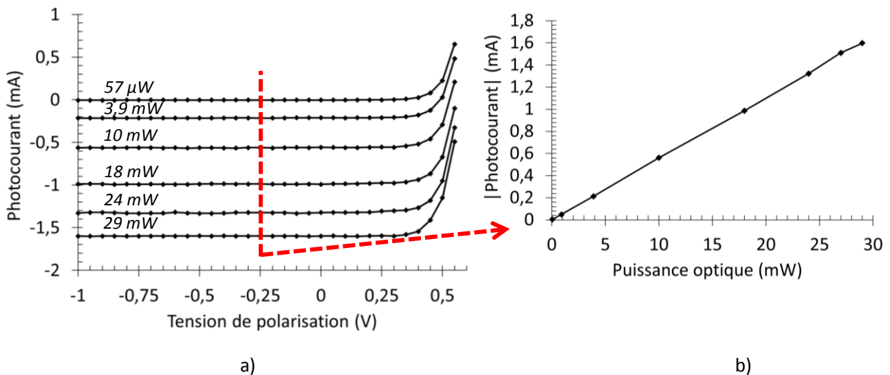
Figure 54: Mesure du photocourant généré par une photodiode de diamètre 10 \mu m en fonction de sa tension de polarisation pour des puissances optiques de 0,06 mW à 29,20 mW en sortie de fibre optique.
