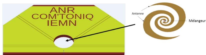
Figure 90: PCB hôte pour mélangeur subharmonique en RO3003.
