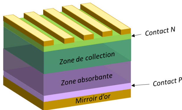
Figure 25: Photodiode résonante en cavité.
