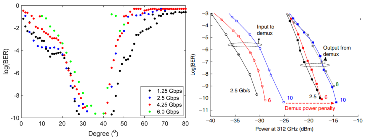
Figure 105 : Mesure du BER à différents angles à 300 GHz pour différents débits (gauche) et mesures en transmission dans le guide (droite).
