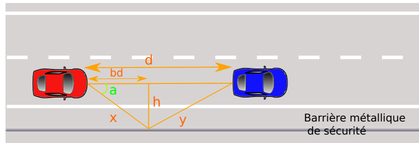
FIGURE 6.17 – Exemple d’une erreur systématique : pour un certain angle a propre au radar à côté d’une glissière de sécurité le véhicule qui précède sera vu à une distance bd inférieure à la distance réelle d
