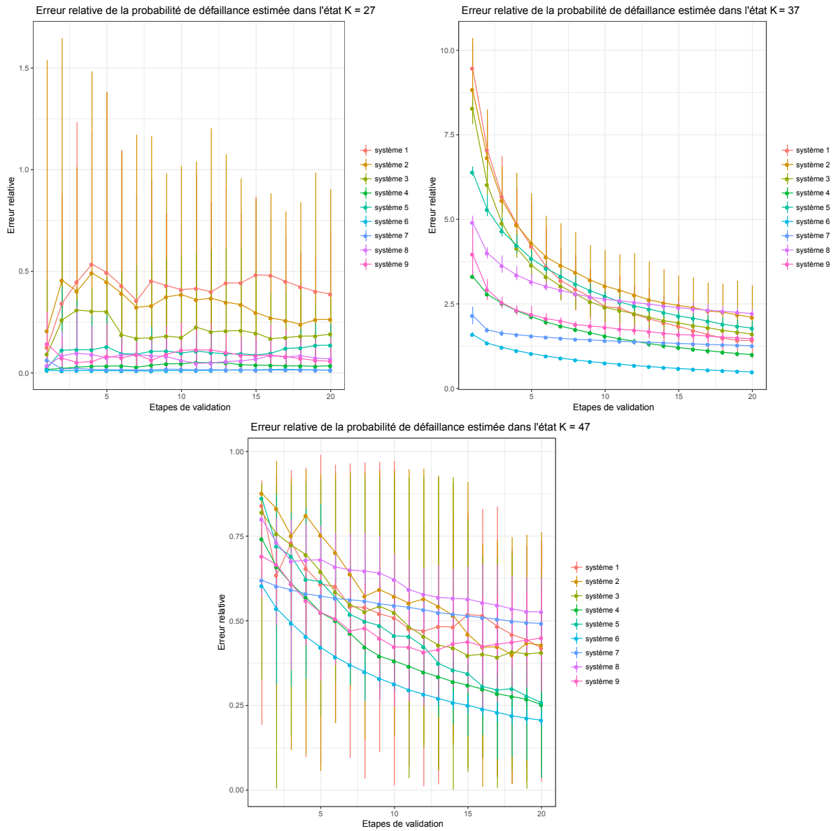
FIGURE 8.10 – Erreur relative de la probabilité de défaillance avant une une heure de roulage estimée pour les mêmes niveaux de connaissance 27,37 et 47 avec différents systèmes.
