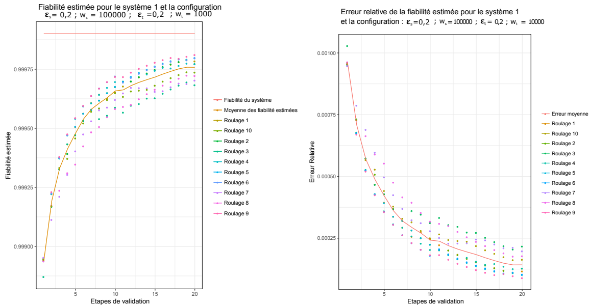
FIGURE 8.4 – Evolution de la fiabilité estimée sur 10 séquences de validation différentes dans le cas où la fiabilité a priori est plus faible que la fiabilité du système
