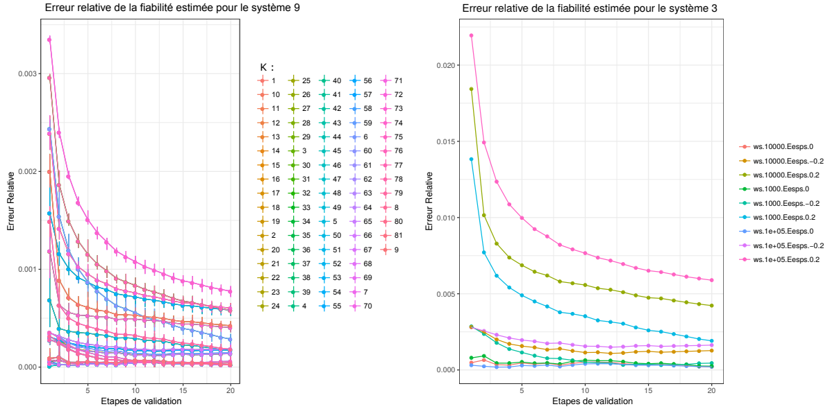
FIGURE 8.8 – Evolution de la fiabilité estimée d'un second système pour 81 niveaux de connaissances différents puis en omettant les variations de w_t et \epsilon_t
