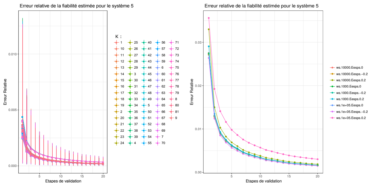
FIGURE 8.12 – Evolution de l'erreur relative de la fiabilité estimée pour le système à cinq cas d'usage dans tous les états de connaissance
