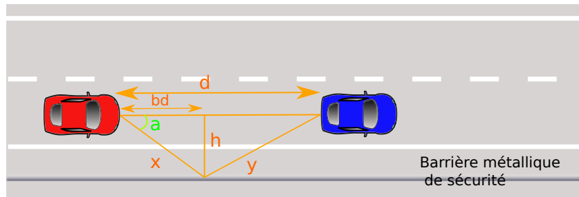
FIGURE 6.17 – Exemple d’une erreur systématique : pour un certain angle a propre au radar à côté d’une glissière de sécurité le véhicule qui précède sera vu à une distance bd inférieure à la distance réelle d
