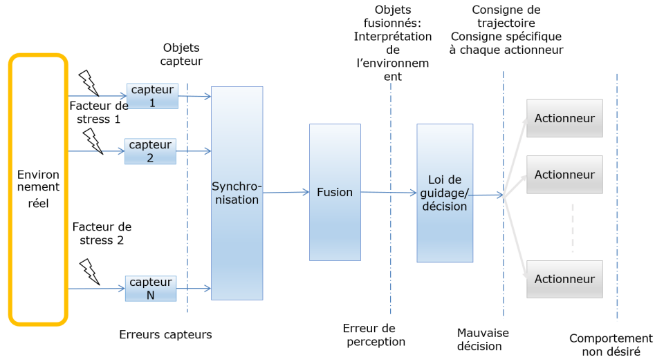
FIGURE 2.2 – Système de perception et de décision
