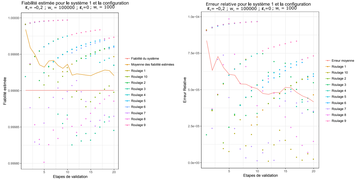
FIGURE 8.6 – Evolution de la fiabilité estimée sur 10 séquences de validation différentes dans le cas où la fiabilité a priori est plus grande que la fiabilité du système
