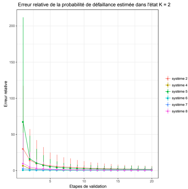
FIGURE 8.13 – Evolution de l’erreur relative de la probabilité de défaillance dans l’état de connaissance K2 pour tous les systèmes
