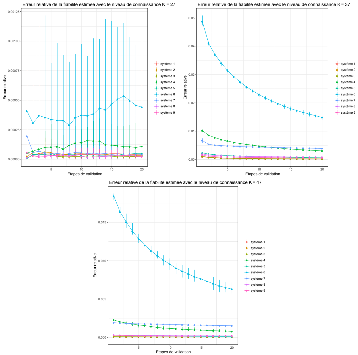
FIGURE 8.9 – Erreur relative de la fiabilité estimée pour les niveaux de connaissance 27,37 et 47 avec différents systèmes
