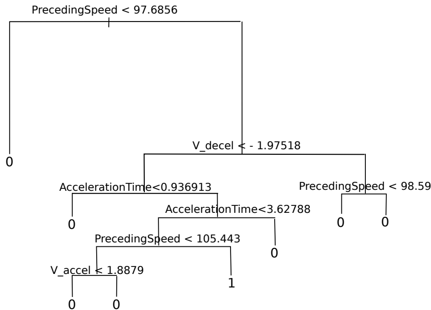
FIGURE 6.8 – Exemple de diagramme CART obtenu lors de l’analyse du cas d’usage suivi de véhicule pour l’indicateur "durée avant de retourner à une distance sécuritaire", 1 indique les feuilles comportant des défaillances, 0 les zones sans défaillance
