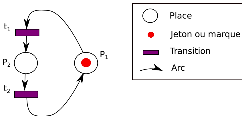
FIGURE 3.2 – Exemple de réseaux de Pétri
