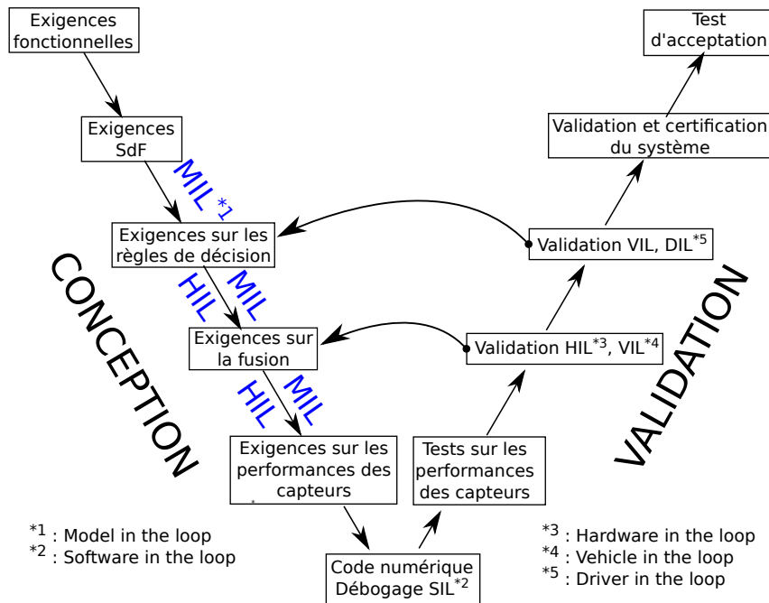
FIGURE 2.4 – Cycle en V du système de perception et de décision des ADAS et AD
