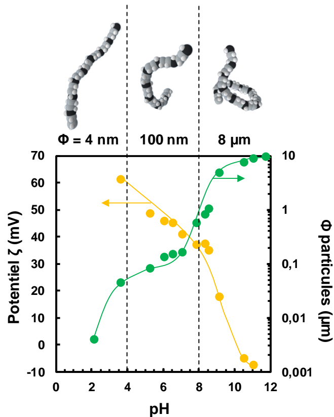
Figure 2.23 : Potentiel zêta (●) et diamètre des particules (●) en fonction du pH pour des dispersions à 0,1 %m de LPEI dans l'eau. La gamme de pH est séparée en 3 zones distinctes correspondant à la conformation de la chaîne de LPEI.
