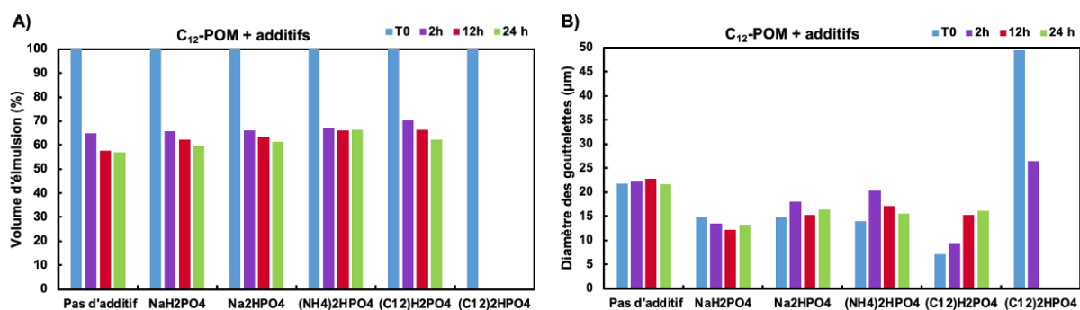
Figure 4.8 : A) Évolution du volume des émulsions E/H et B) diamètre moyen des gouttelettes pour les combinaisons de C_{12} -POM + additifs. 0,75 mL de toluène, 2,25 mL d'eau, 100 mg de NPs, 2 équivalents d'additif par rapport au C_{12} -POM. Émulsification à l'Ultraturrax à 11500 rpm pendant 1 min.
