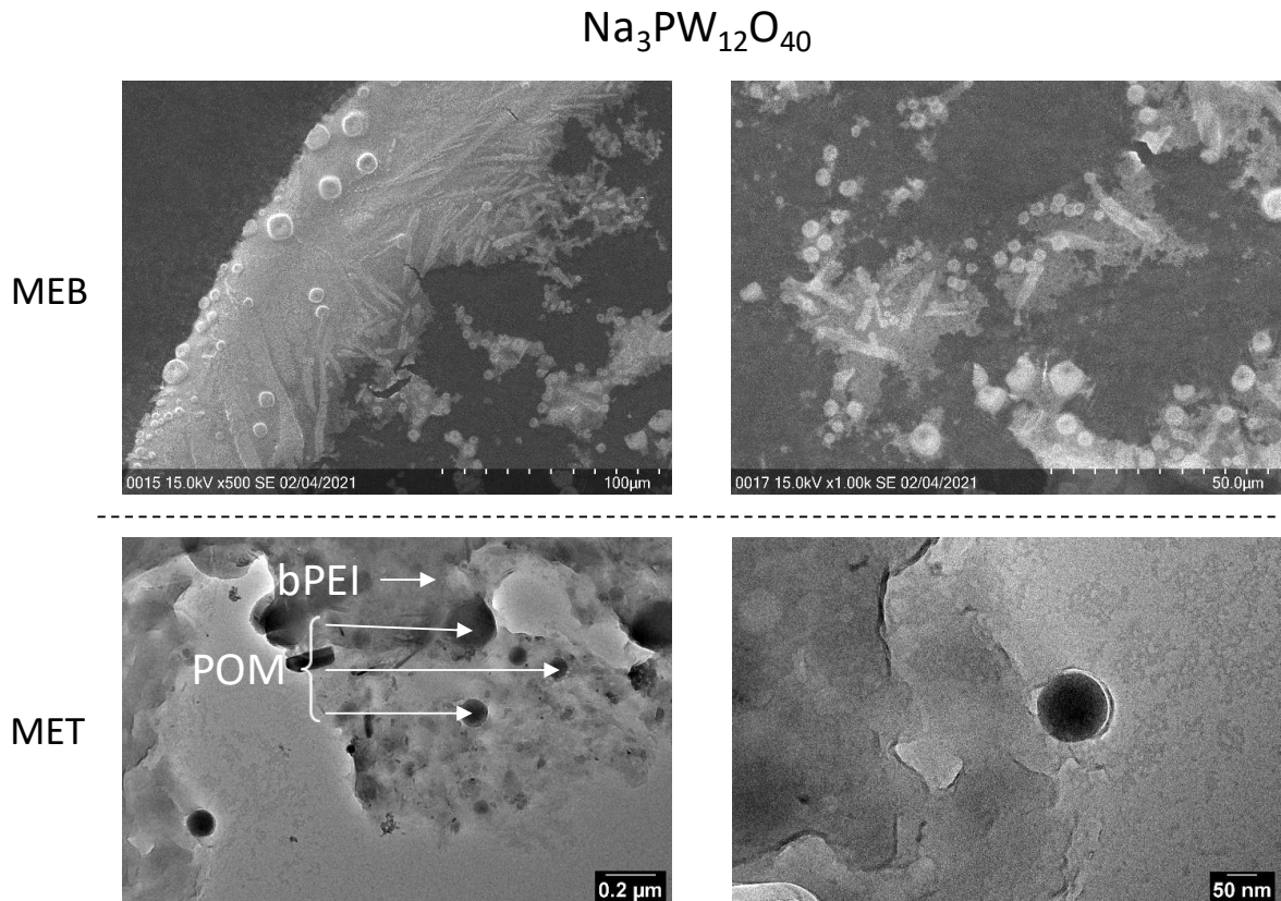
Figure 4.19 : Images MEB et MET des particules auto-assemblées de PEI-POM synthétisées à partir d'un mélange de BPEI (50 μM) et de \text{Na}_3\text{PW}_{12}\text{O}_{40} (50 μM).
