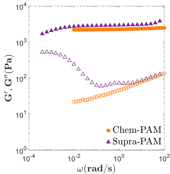
Figure 15. Propriétés rhéologiques dynamiques des gels chimique (orange) et supramoléculaire (violet) réticulé à 0,1 mol%. Module élastique ( G' , symbole plein) et module visqueux ( G'' , symbole vide) en fonction de la fréquence angulaire mesurés sur l'état de préparation (25 °C, \gamma = 1\% ).
