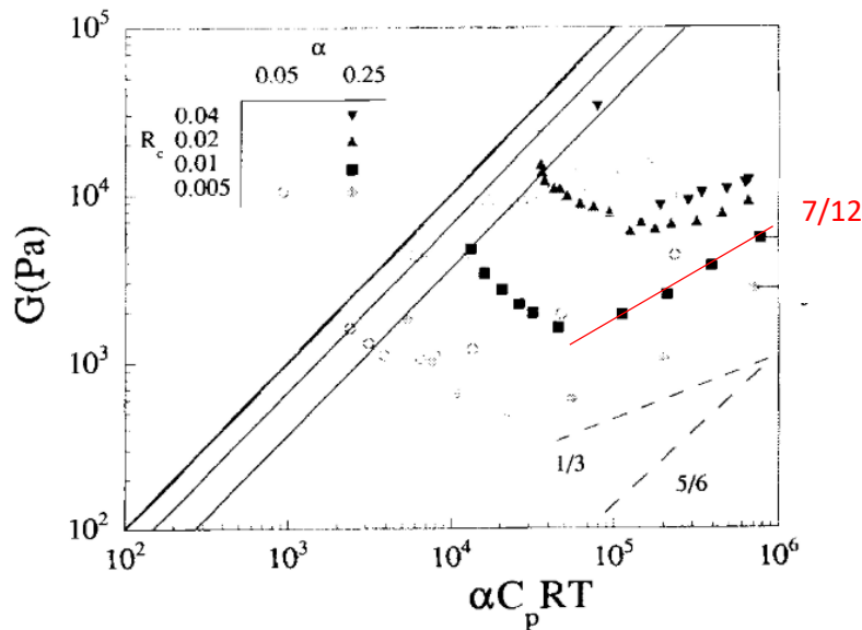
Figure 18. Module élastique d'un gel polyelectrolyte de polyacide acrylique (7 wt% de polymère) en fonction du gonflement en eau pure pour différents taux d'ionisation \alpha et différents taux de réticulation R_c à 20 °C. D'après Nisato et al. 76
