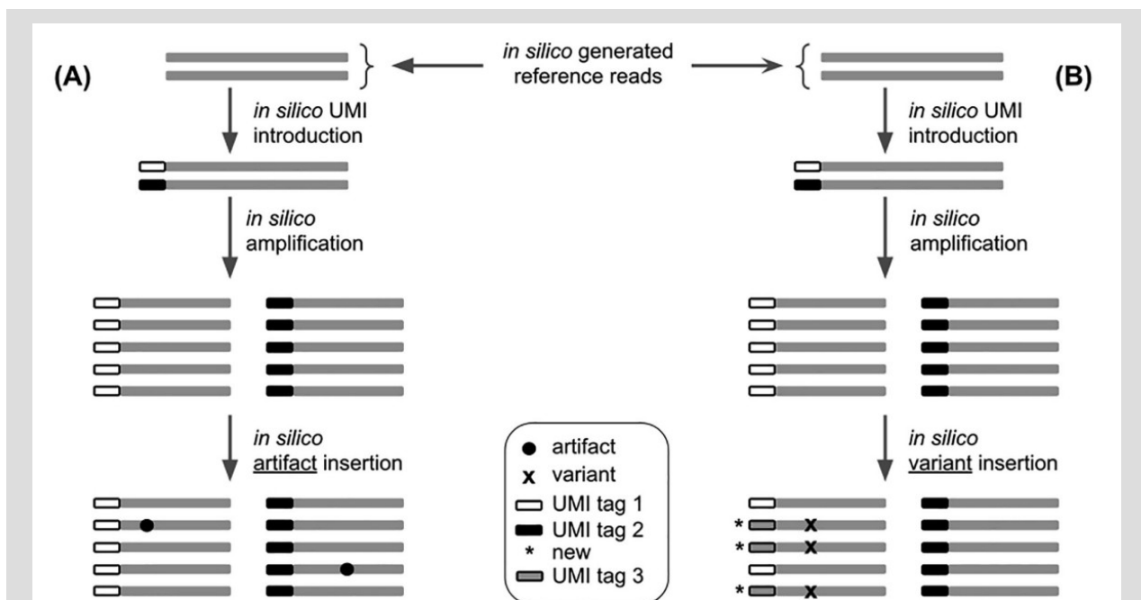
Figure 66: UMI-Gen - Introduction du bruit de fond de séquençage et des vrais positifs.
