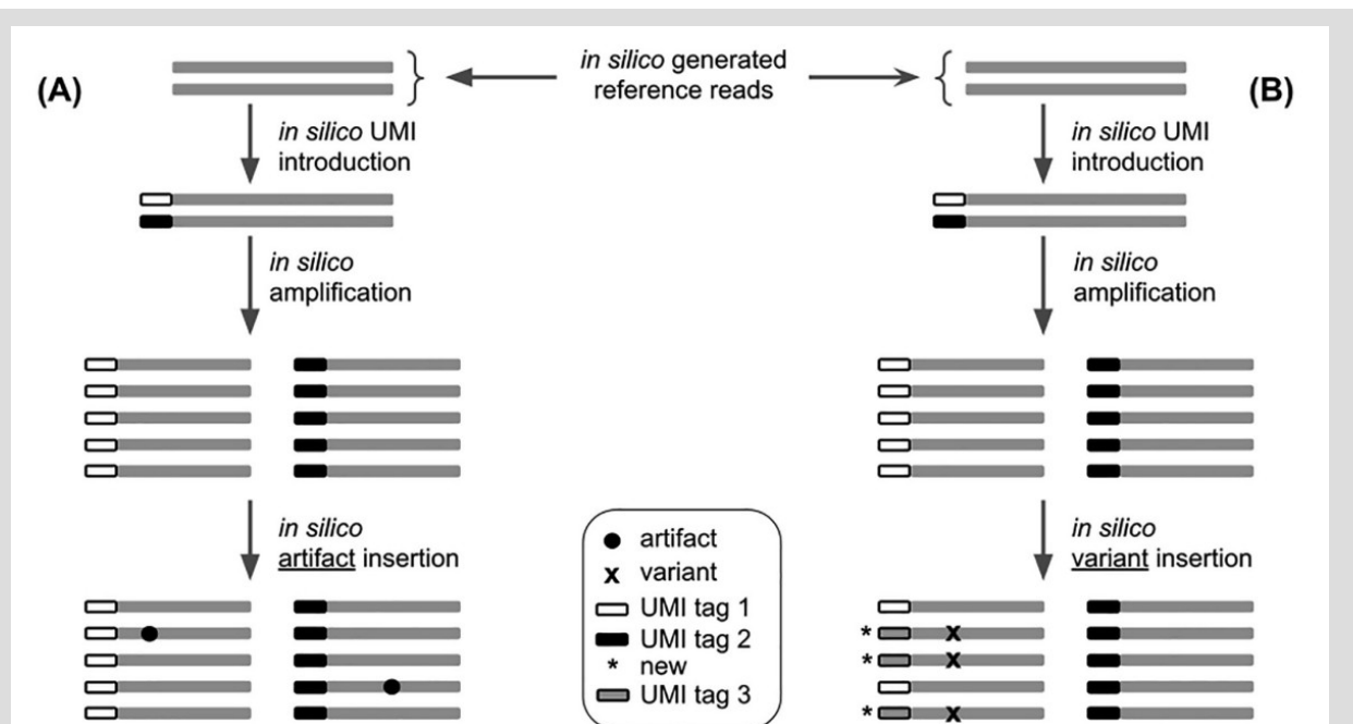
Figure 66: UMI-Gen - Introduction du bruit de fond de séquençage et des vrais positifs.
