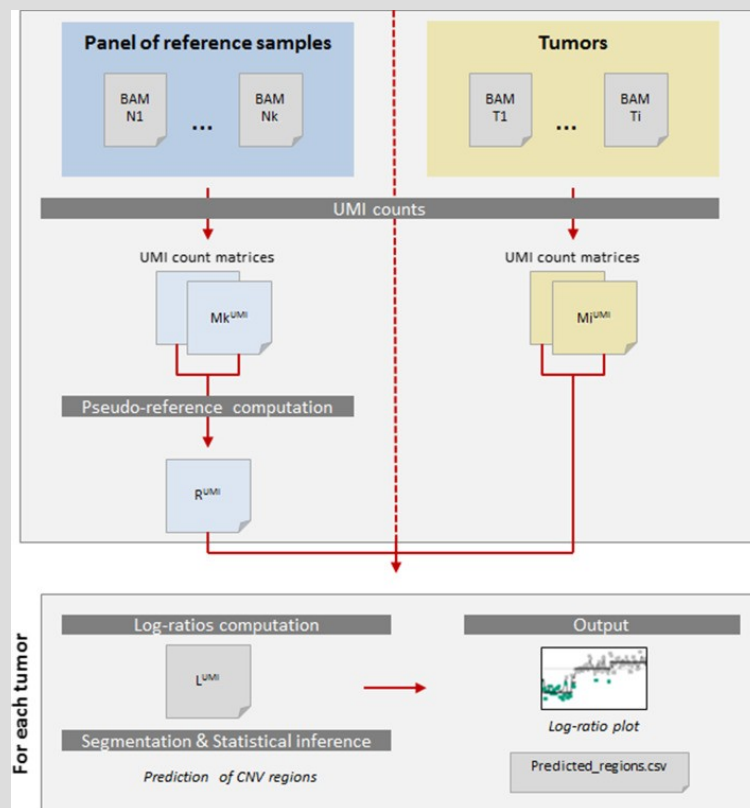
Figure 58: mCNA : fonctionnement de l'algorithme.
