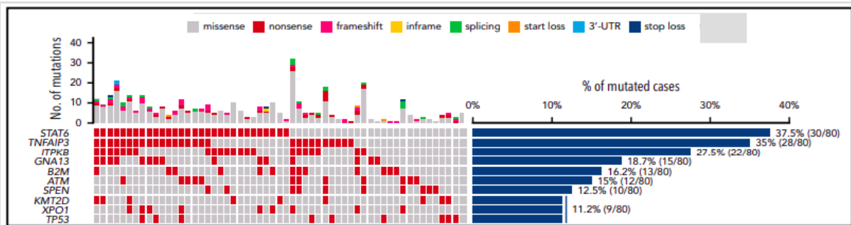
Figure 37: Profils mutationnels de 80 cfDNA de LH (adapté de V. Spina et al, Blood 2018)
