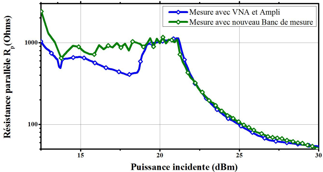
FIGURE 4.23 – Comparaison des mesures d'impédance (à 13.56 MHz) en fonction de la puissance incidente, entre la mesure effectuée par le banc de mesure décrit dans cette partie et par un VNA avec amplificateur. L'axe des ordonnées adopte une échelle logarithmique
