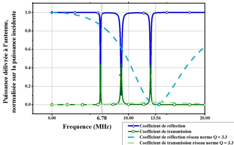
FIGURE 3.58 – Puissance transmise à l'antenne et réfléchié par le réseau terminé par l'antenne lorsque la puissance incidente est de 1 W, avant qu'une optimisation ne soit faite
