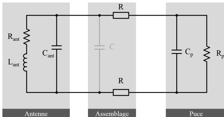
FIGURE 4.2 – Modèle électrique complet d'un tag, avec l'antenne, la puce, une capacité d'accord (optionnelle) et de connection "C", et des résistances de connection entre la puce et la carte, négligeables
