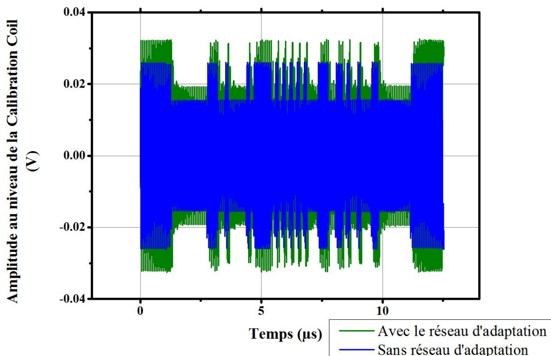
FIGURE 3.46 – Forme d'onde des signaux transmis par un lecteur avec et sans réseau d'adaptation. La tension visualisée est celle récupérée aux bornes de la bobine de calibration placée sur le Test PCD Assembly, comme indiqué en Fig. 2.10
