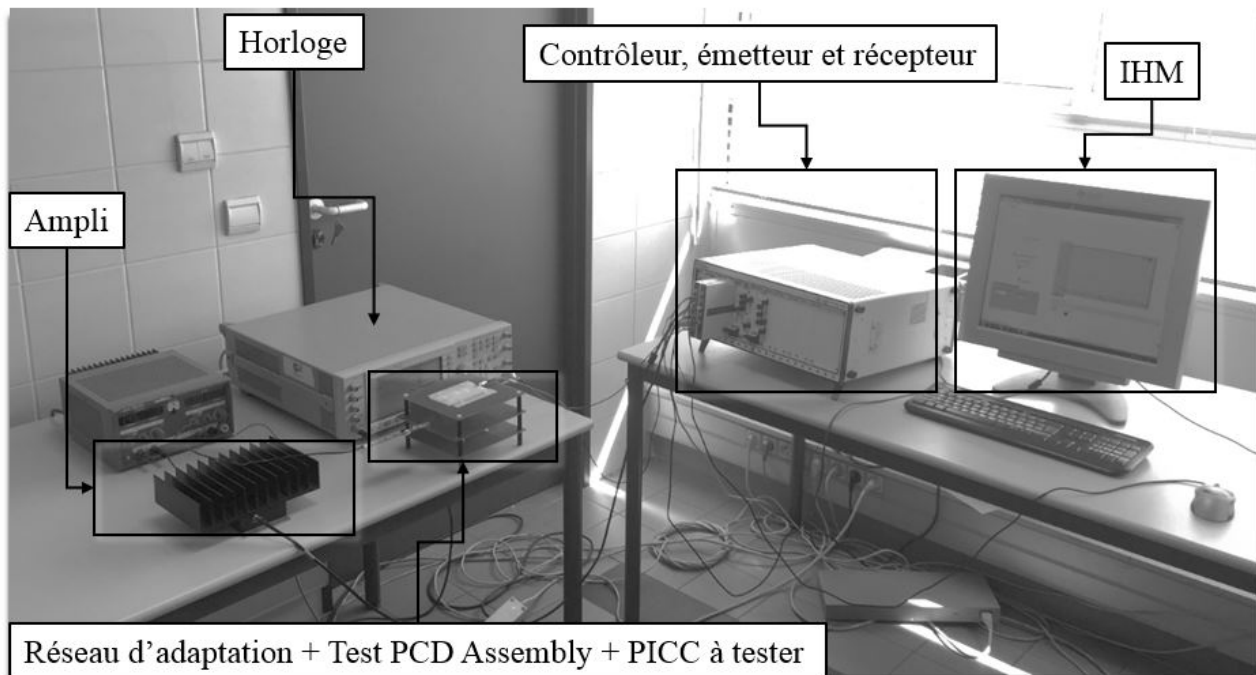
FIGURE 2.16 – Implémentation de la plateforme de pré-certification
