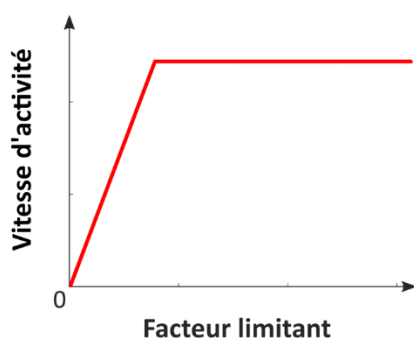
Figure I.4. Relation de Blackman entre l'activité d'une population et la présence du facteur limitant.
