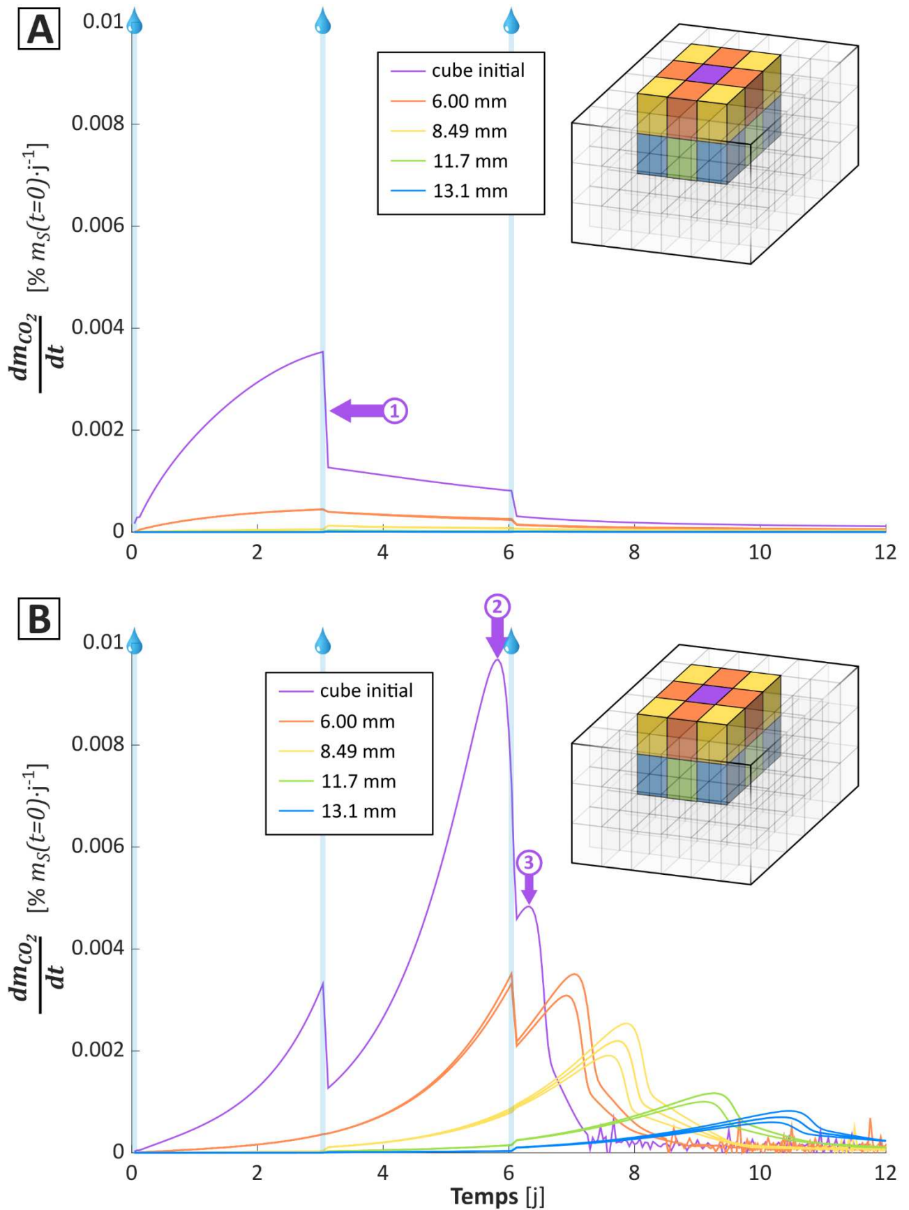
Figure III.6. Localisation des flux de carbone à travers les émissions de CO_2 , pour le modèle de Monod calibré en hydrostatique (A) et pour le modèle de Monod calibré en hydrostatique et percolation (B). Les paramètres biologiques correspondent à leur valeur calibrée, mais le
