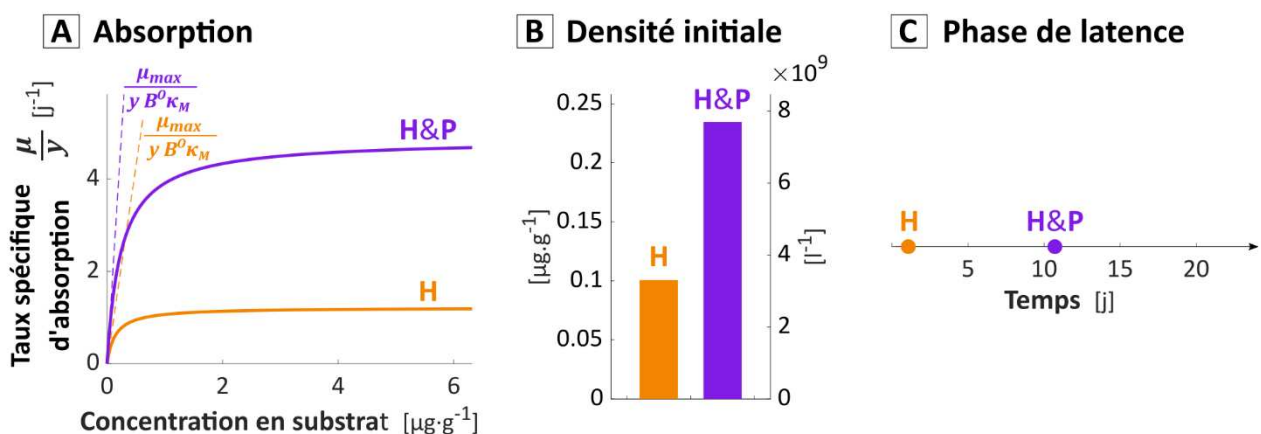
Figure III.2. Traits d'histoire de vie des modèles de Contois calibrés sur les données expérimentales de Pinheiro et al. (2015, 2018). Pour les légendes, se reporter à la figure précédente. Les efficacités maximales d'absorption sont représentées pour une densité bactérienne de référence B^0 = 5 \cdot 10^{-2} \mu\text{g}\cdot\text{g}^{-1} (masse de carbone bactérien par masse de sol sec).
