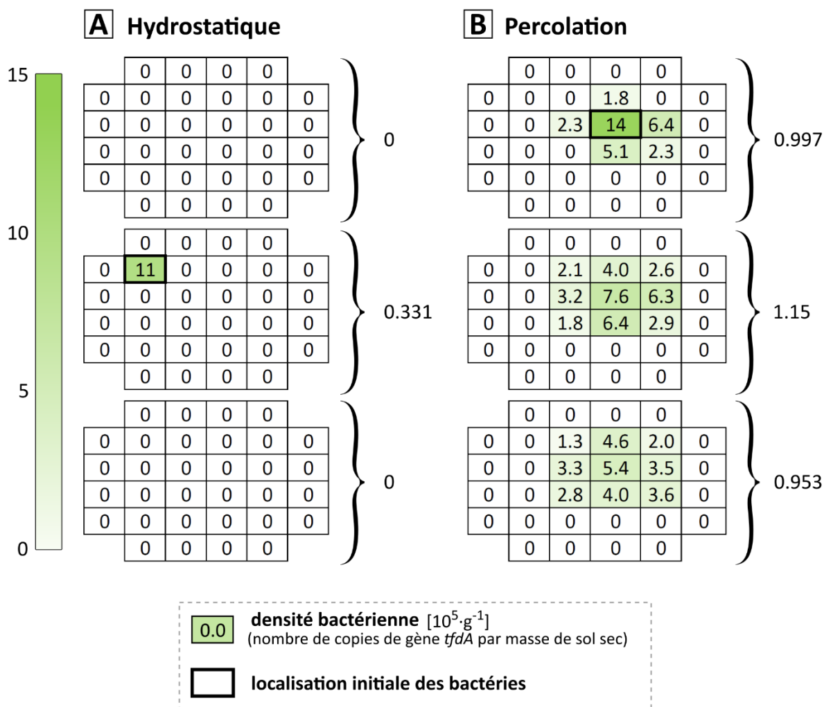
Figure II.6. Répartitions millimétriques finales des bactéries dégradantes du 2,4-D, dans l'expérience hétérogène colocalisée, en conditions hydrostatiques (A) et en percolation (B), après 24 jours. Les 96 cubes élémentaires des colonnes de sol sont représentés sur trois grilles correspondantes aux trois couches de sol. Les valeurs se réfèrent aux mesures finales du nombre de copies de gènes tfdA , aussi illustrées par l'échelle de couleur verte. Les nombres indiqués à droite des cartes représentent les densités moyennes par couche. Le cube avec les bordures épaisses indique la position initiale des bactéries. La limite de détection était 0.12 \cdot 10^5 \text{ g}^{-1} (copies de séquences tfdA par masse de sol sec). Les conditions aux bords étaient réfléchissantes (pas de fuite de carbone) à l'exception du bas de la colonne en contact avec une plaque de céramique permettant le maintien du potentiel hydrique. Lors des événements d'irrigation, l'eau était
