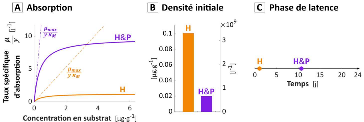
Figure III.1. Traits d'histoire de vie des modèles de Monod calibrés sur les données expérimentales de Pinheiro et al. (2015, 2018). Les paramètres décrivant l'activité métabolique des bactéries \mu_{max}/y et (1/y)\cdot\mu_{max}/\kappa_M (A), les densités initiales B(t=0) (B) et la durée de l'accommodation (C), définie comme 1/\alpha , sont illustrés pour le modèle calibré en hydrostatique seulement (en orange) et le modèle calibré en hydrostatique et percolation (en violet).
