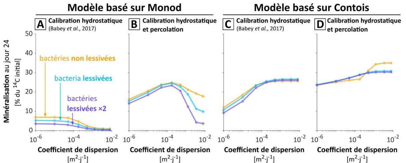
Figure III.14. Impact de la lixiviation des bactéries sur la minéralisation finale en fonction de la dispersion des bactéries, pour le traitement colocalisé en percolation. Trois modalités de lixiviation des bactéries sont représentées : pas de lixiviation (en orange), lixiviation des bactéries égale en proportion à celui du substrat (en bleu), lixiviation des bactéries égale en proportion au double de celui du substrat (en violet). Les résultats en bleu correspondent aux résultats présentés précédemment dans le manuscrit de la section III.1.2. Les résultats sont montrés pour les modèles de Monod (A-B) et de Contois (C-D), pour les jeux de paramètres biologiques calibré sur les traitements hydrostatiques seuls (A et C) ou calibré sur les traitements hydrostatiques et en percolation (B et D).
