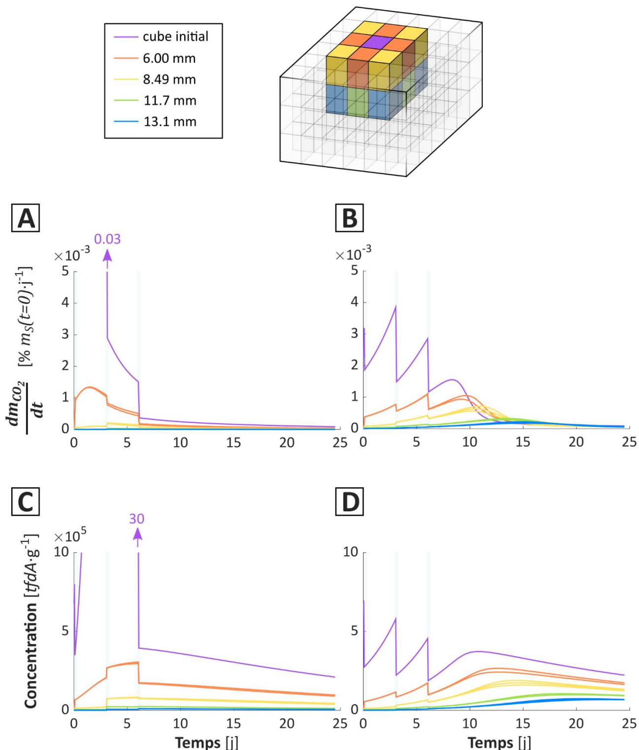
Figure III.8. Localisation des flux de carbone à travers la dynamique du CO 2 (A, B) et des bactéries (C, D), pour les bactéries copiotrophes (A, C) et oligotrophes (B, D) « modèles ». Les deux jeux de paramètres sont définis en section III.1.4.2. Le coefficient de dispersion d_{disp} est choisi identique
