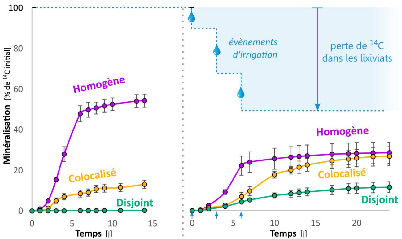
Figure II.3. Production cumulée de CO 2 mesurée dans les expériences de Pinheiro et al., (2018, 2015). Les noms des expériences se rapportent à la Figure II.1.
