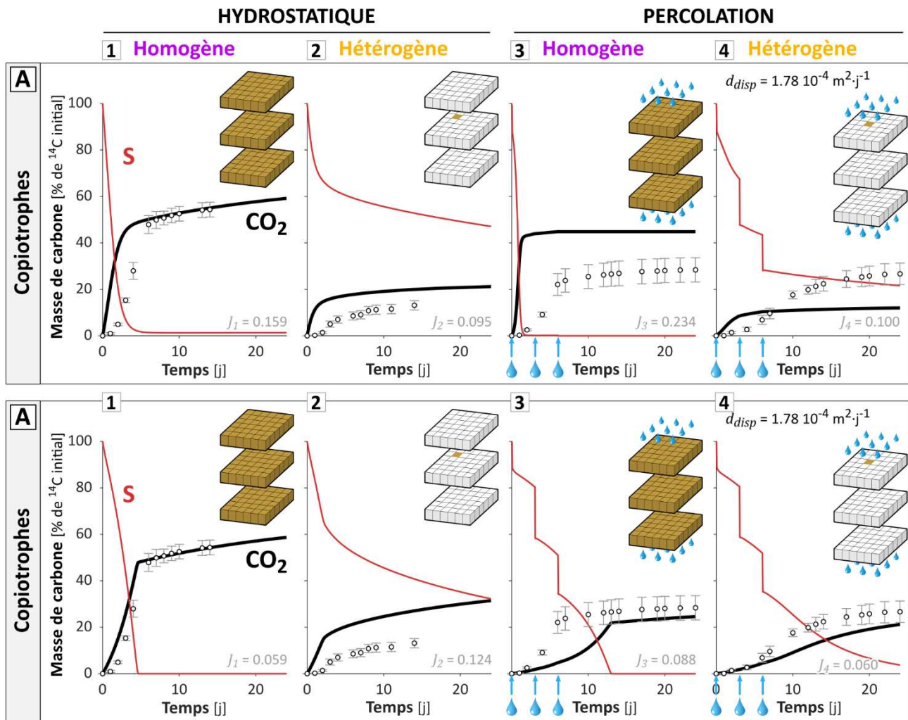
Figure III.5. Dynamiques de minéralisation prédites avec le modèle de Monod pour les jeux de paramètres représentant des bactéries copiotrophes (A) et oligotrophes (B) « modèles ». Les configurations expérimentales correspondantes sont illustrées dans l'angle supérieur droit de chaque graphique. L'adéquation entre les observations et les simulations est indiquée par la valeur de la divergence J en bas des graphiques et peut être évaluée visuellement par la proximité entre la ligne noire et les points, représentant respectivement les résultats du modèle et les données expérimentales. La ligne rouge représente la masse de ^{14}\text{C} du substrat restant dans la colonne de sol. Dans les expériences en percolation (A3-4 et B3-4), environ 51% de la masse initiale de ^{14}\text{C} a été perdue par lixiviation lors de chaque événement de percolation ( t = 0, 3 et 6 jours, flèches bleues).
