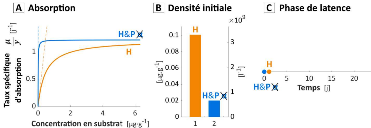
Figure III.3. Traits d'histoire de vie des modèles de Monod calibrés sur les données expérimentales, en hydrostatique (en orange) et en percolation et hydrostatique mais sans latence \alpha (en bleu).
