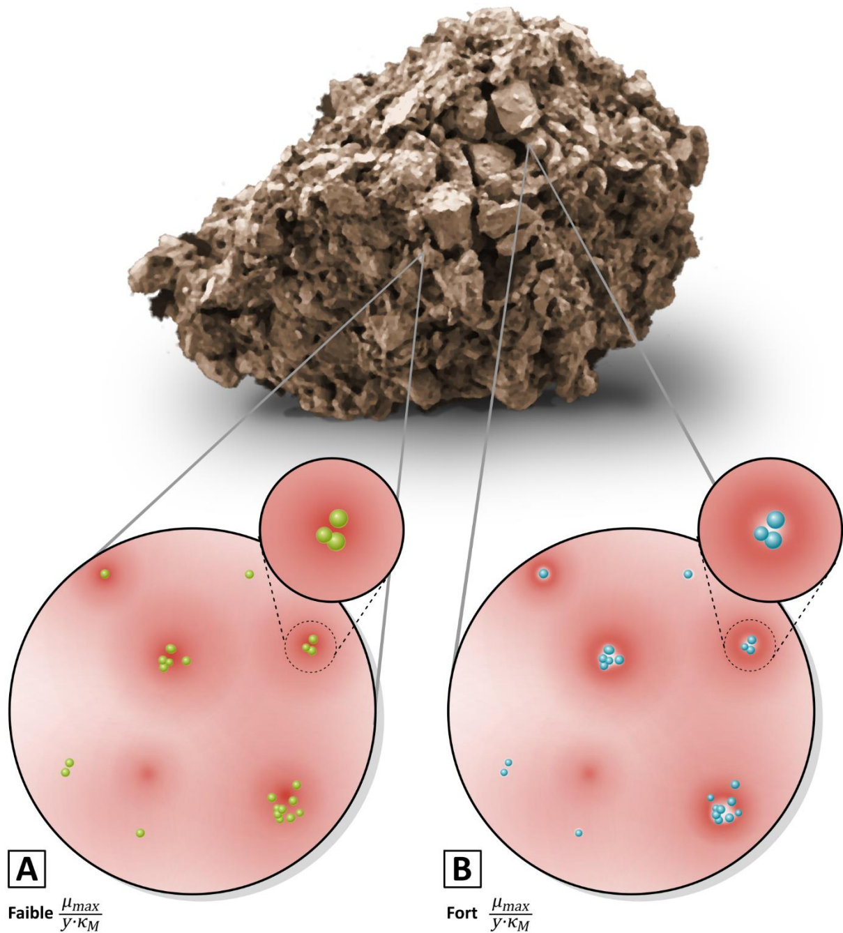
Figure III.9. Représentation graphique de deux situations opposées en termes d'impact de la dispersion. Le substrat (en rouge) présente une distribution hétérogène similaire dans les deux situations, avec quelques zones plus propices à recevoir des apports organiques et donc présentant des concentrations en substrat plus élevées. Les bactéries sont placées de manière similaire dans les deux situations, c'est à dire principalement agglomérées à proximité des zones concentrées en substrat, mais les bactéries vertes (A) ont une faible efficacité maximale d'absorption du substrat tandis que les bactéries bleues (B) ont une forte efficacité maximale d'absorption. Il en résulte que les bactéries vertes sont limitées par la dilution du substrat tandis que les bactéries bleues sont limitées par la compétition locale entre elles. Les quelques bactéries bleues solitaires et dispersées dans la partie gauche sont par contre épargnées du problème de l'épuisement local de la quantité de substrat disponible. La dispersion des bactéries (et/ou du
