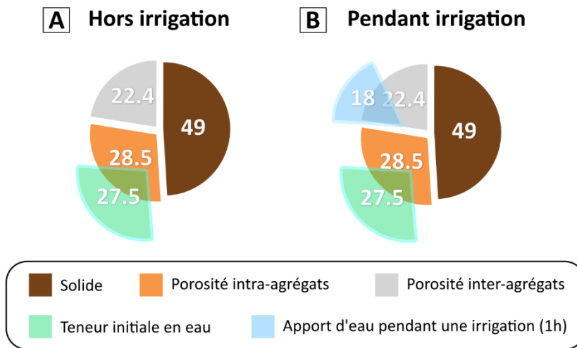
Figure II.2. Bilan de l'évolution de la teneur en eau. Pour les expériences hydrostatiques et les expériences en percolation en dehors des épisodes d'irrigation, la teneur en eau est maintenue constante (A). Pour les expériences en percolation pendant les épisodes d'irrigation, la teneur en eau fluctue temporairement (B). Les trois épisodes d'irrigation apportent approximativement l'équivalent d'un volume poral en eau. Les valeurs en blanc sont indiquées en pourcentage.
