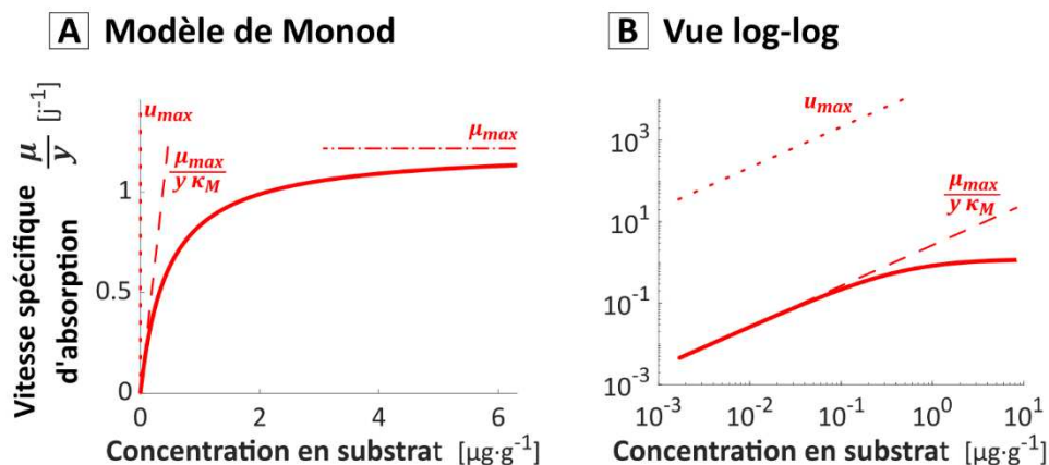
Figure I.5. Modèle de Monod - Relation entre la concentration en substrat et la vitesse d'absorption, avec les paramètres calibrés issus de (Babey et al., 2017). La relation est représentée en traits continus. Dans ce modèle, la vitesse d'absorption tend vers une valeur limite ( \mu_{max} ) quand la concentration en substrat augmente (traits pointillés alternés). A l'inverse, lorsque la concentration en substrat approche zéro, l'absorption bactérienne devient proportionnelle à la concentration en substrat d'un facteur (1/y) \cdot \mu_{max}/\kappa_M (traits pointillés longs), appelé dans ce travail « efficacité maximale d'absorption ». Ce facteur admet une limite physique théorique u_{max} appelé « limite collisionnelle » (traits pointillés courts). Celle limite est ici plus de 8000x supérieure à l'efficacité maximale d'absorption. Le graphique (A) est représenté en échelle logarithmique sur le graphique (B) afin de faciliter la visualisation de la limite collisionnelle.
