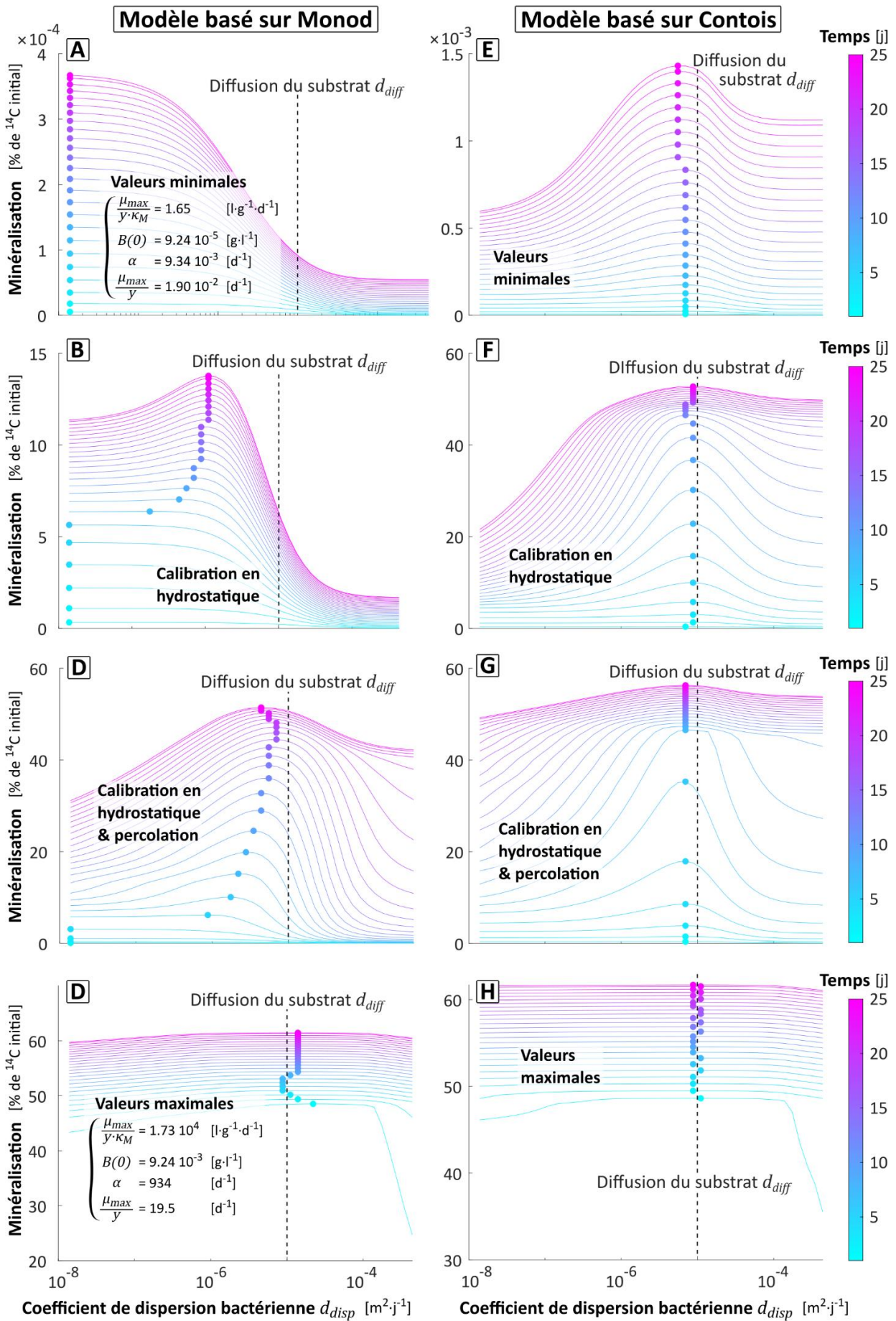
Figure IV.6. Comparaison de la dynamique temporelle de l’optimum de dispersion entre les
